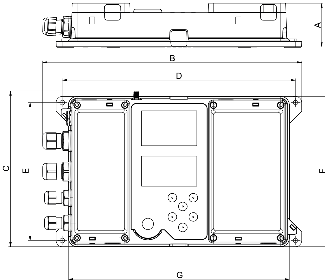
Figure 4 Modus mini - dimensions
