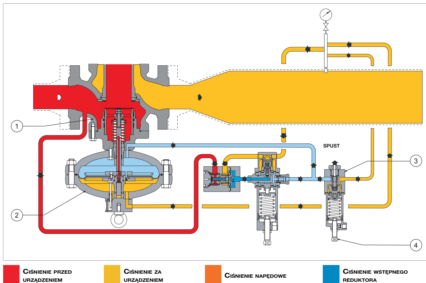
Rys. 4.9. Zawór przyspieszający M/A
