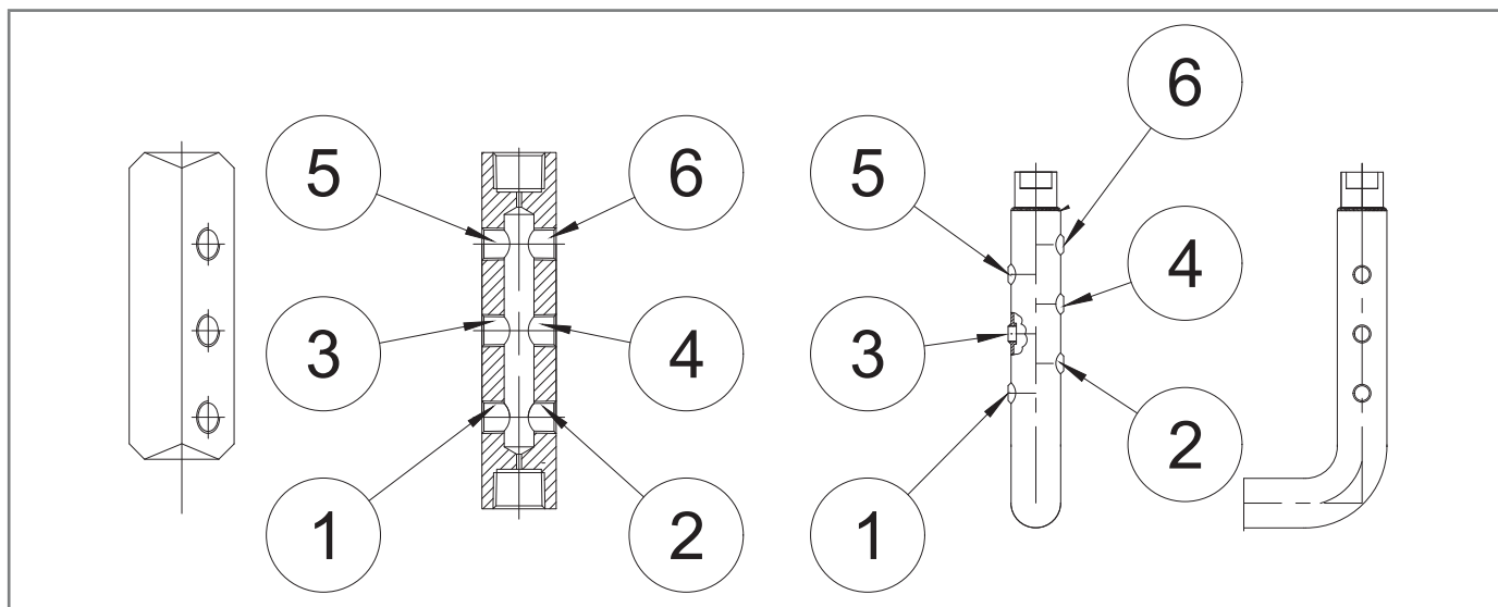
Rys. 6.28. Połączenia urządzenia
