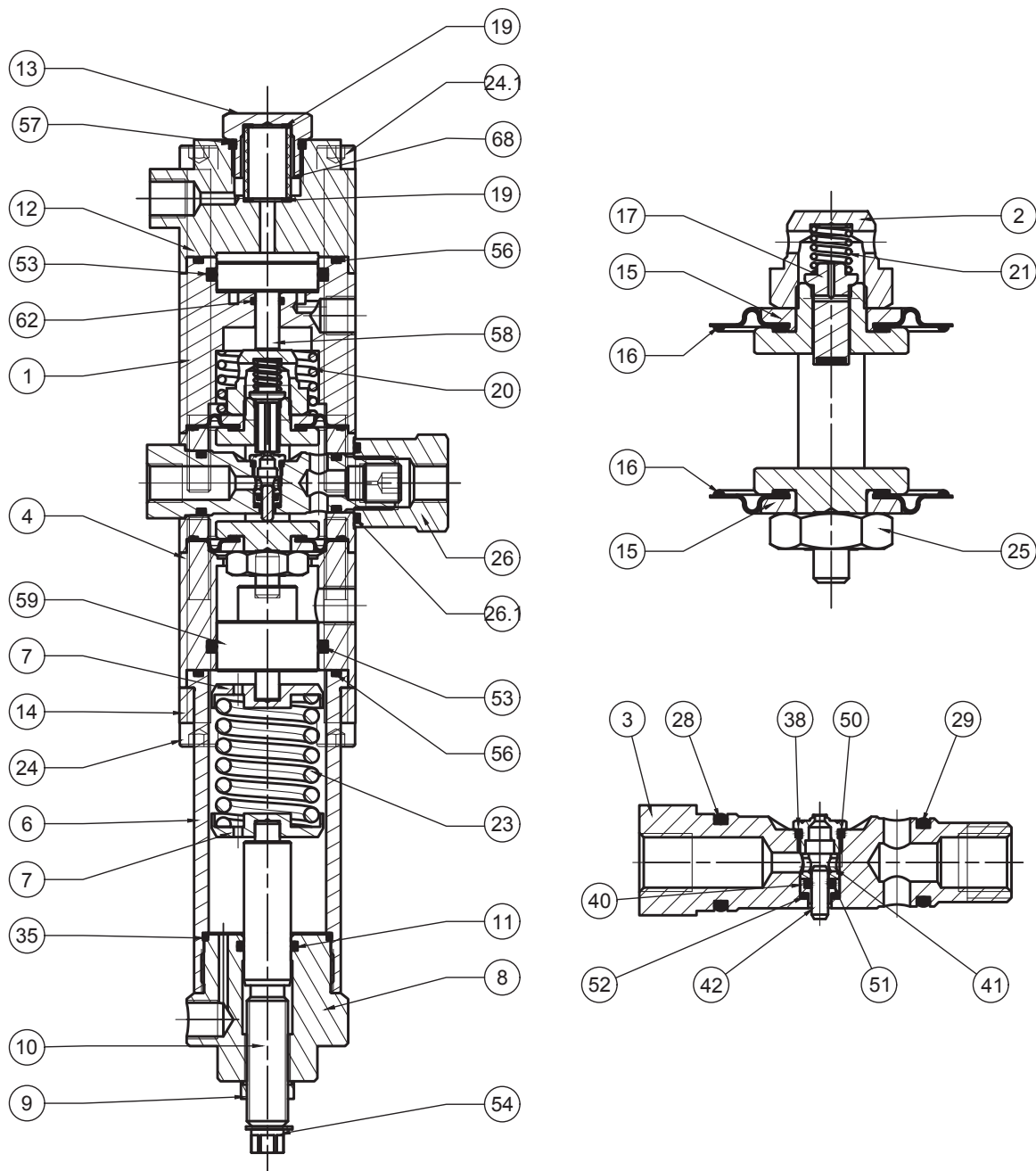
Regulator ciśnienia R44/SS
