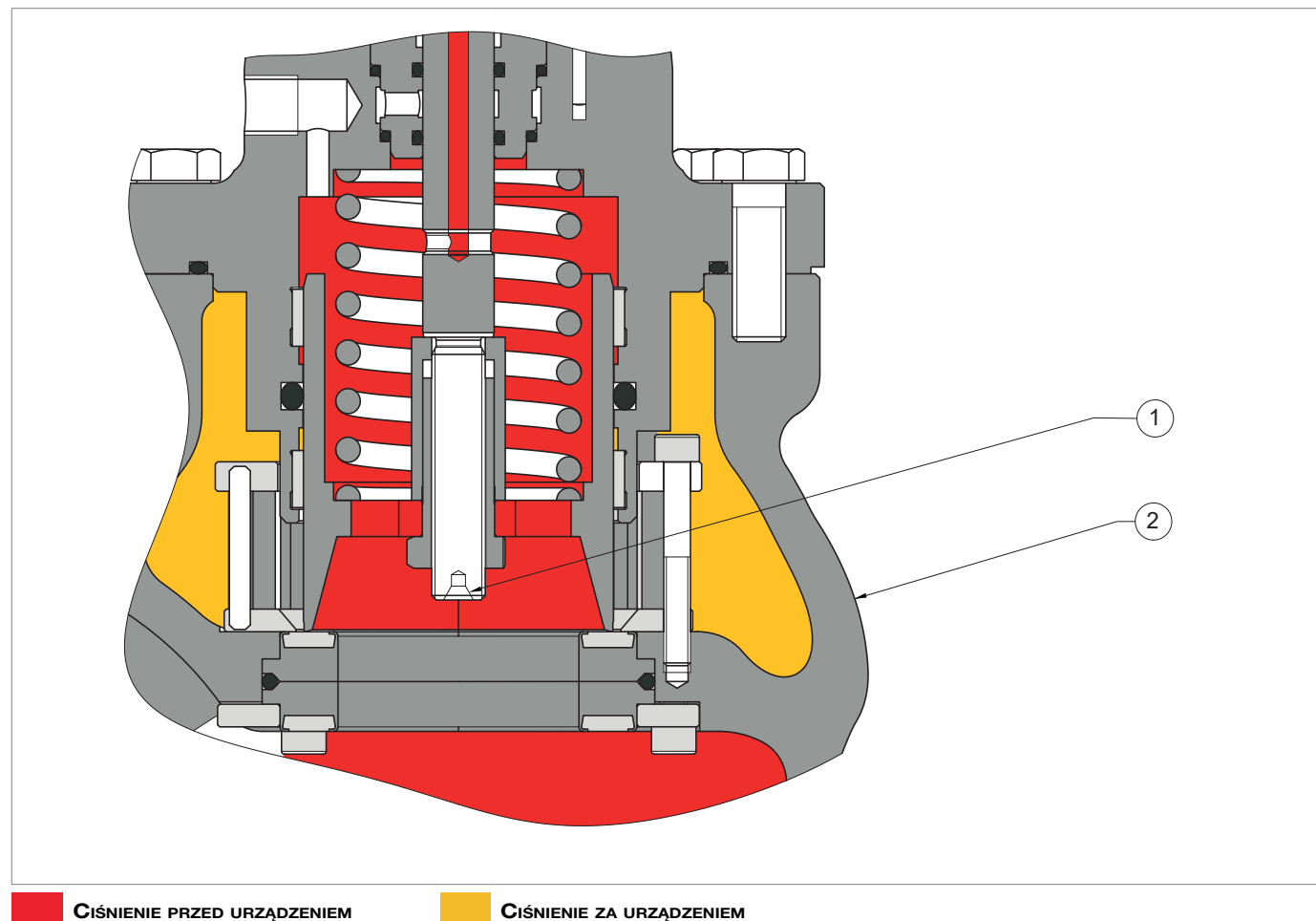
Rys. 4.4. Wbudowany tłumik LDB/171
