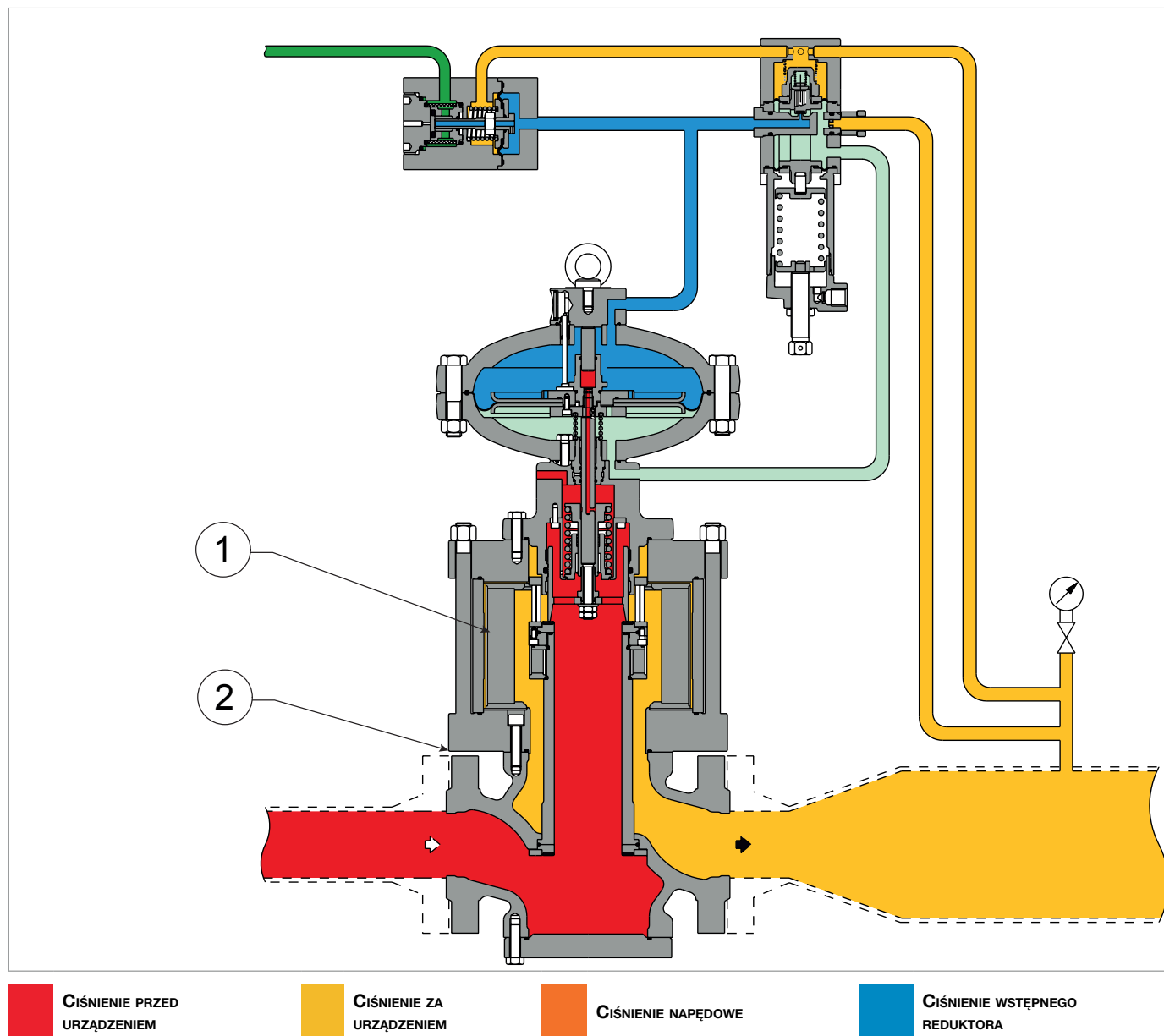
Rys. 4.3. Wbudowany tłumik DB/819
