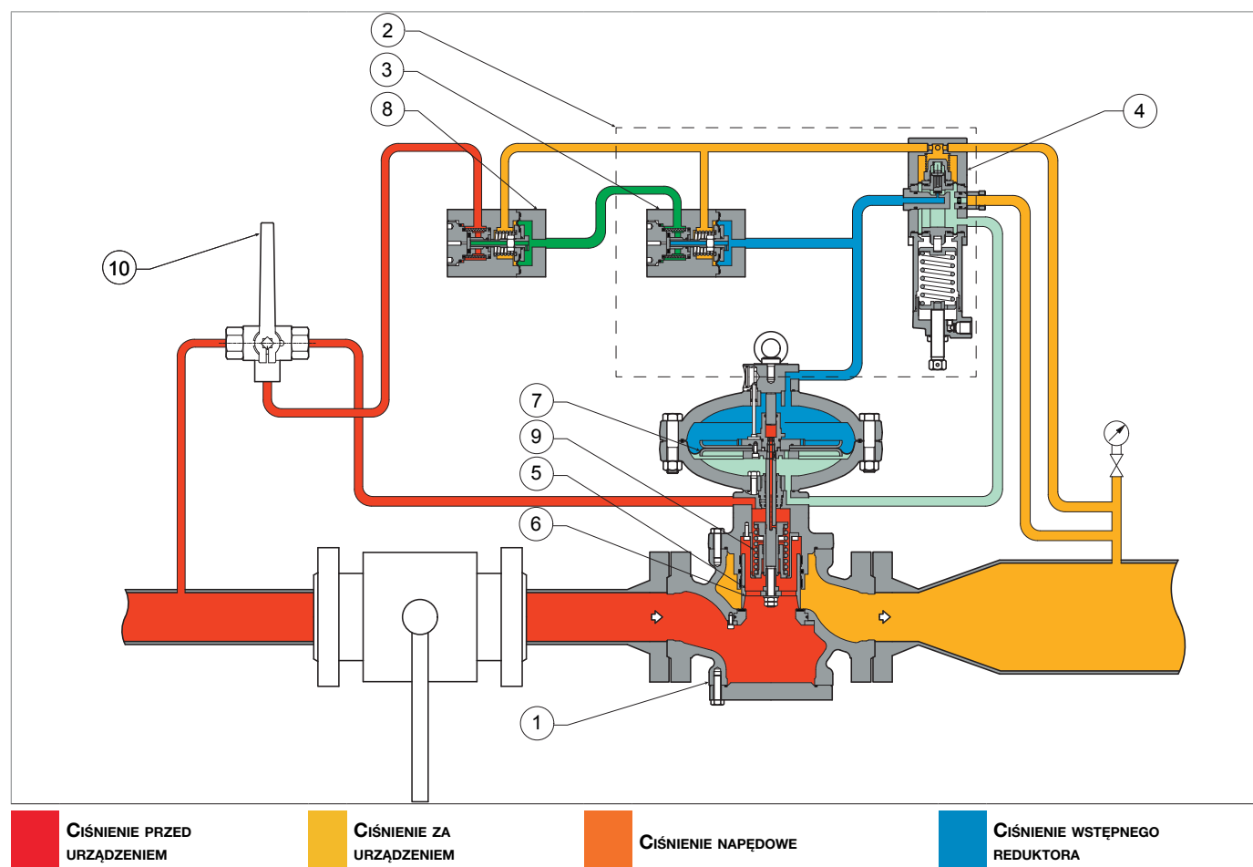
Rys. 4.1. Opis ogólny REFLUX 819/FO
