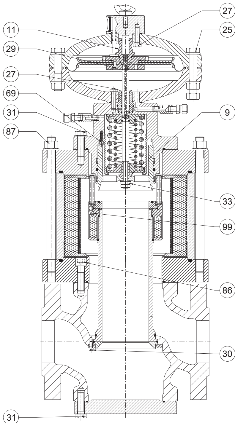
Rys. 9.40. Momenty dokręcania REFLUX 819/FO + Tłumik DB/819
