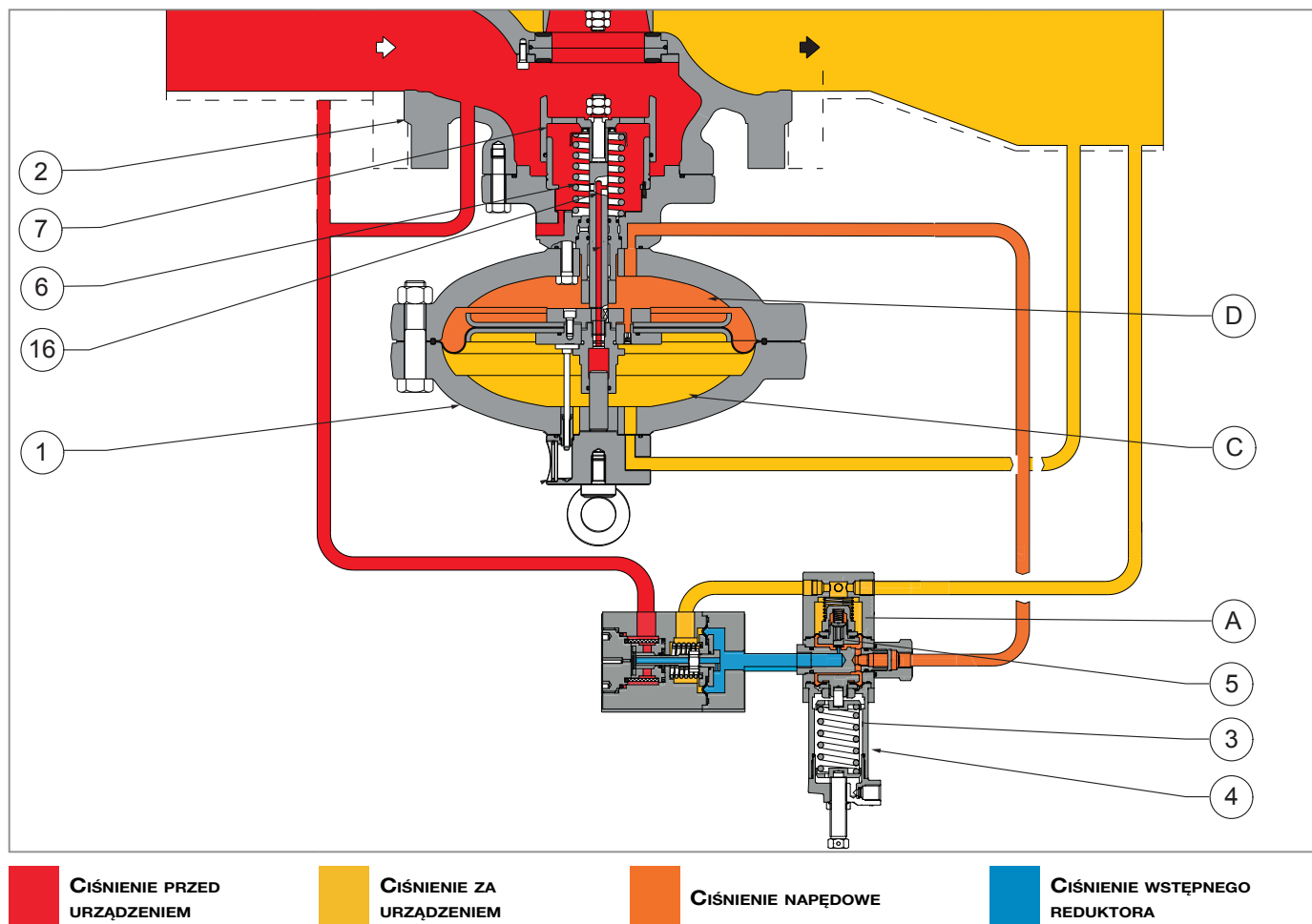
Rys. 4.8. Działanie wbudowanego monitora w przypadku awarii głównego regulatora
