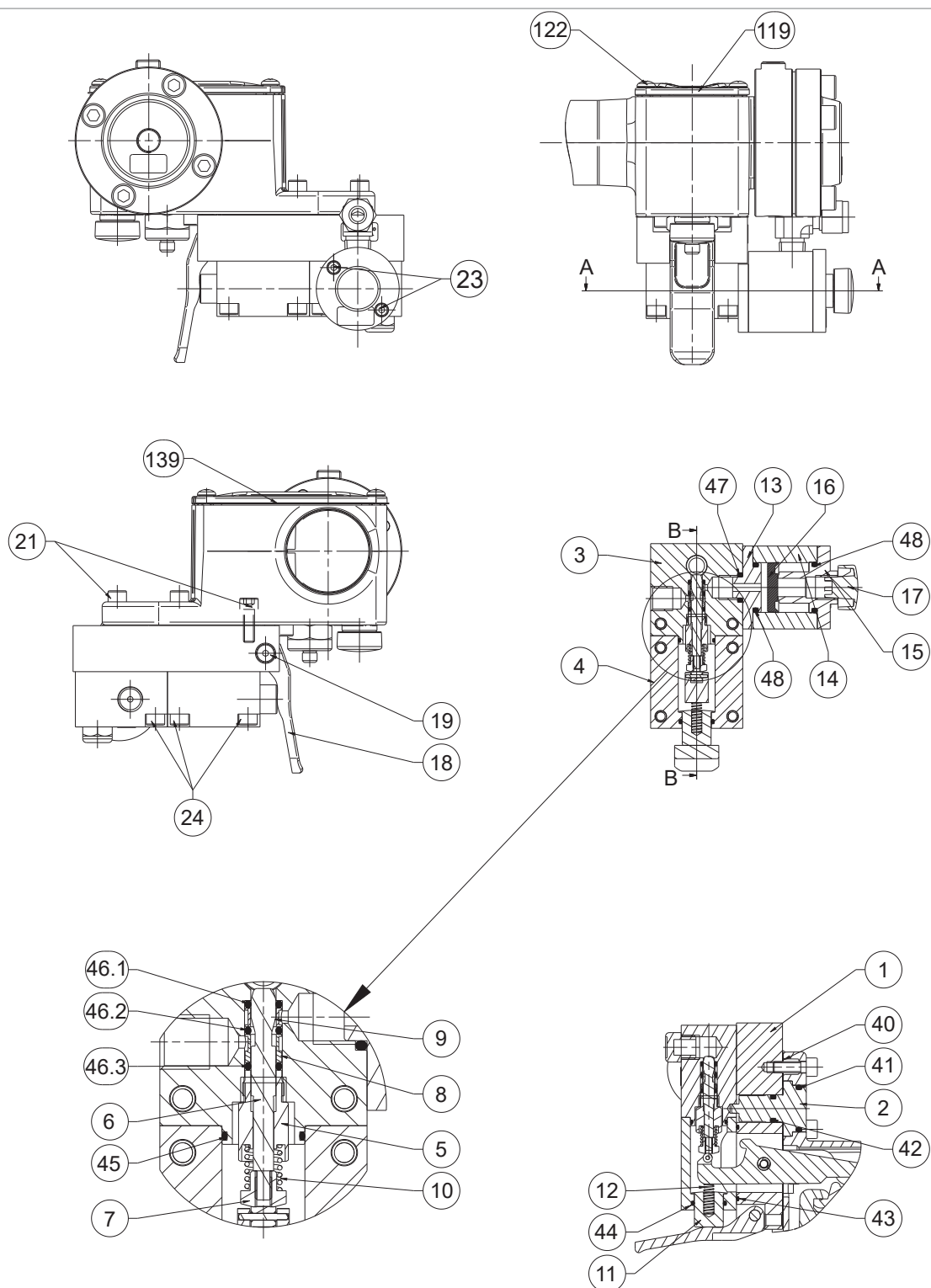
Rys. 9.84. Zawór 3/2
