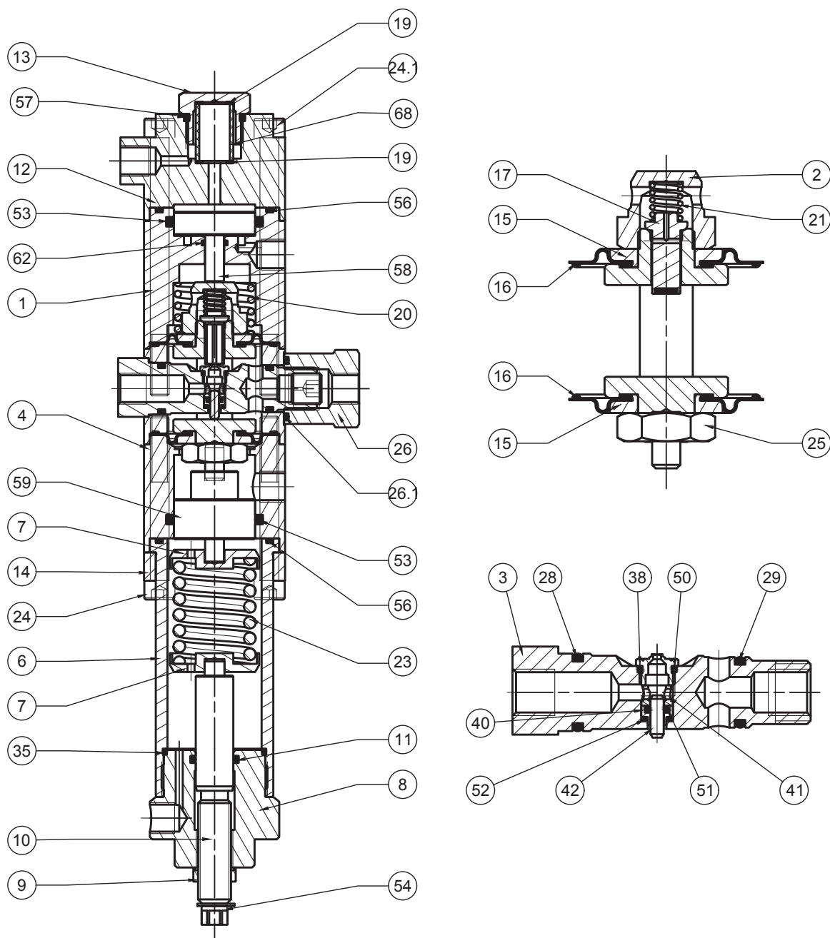
Rys. 9.82. Regulator ciśnienia R44/SS
