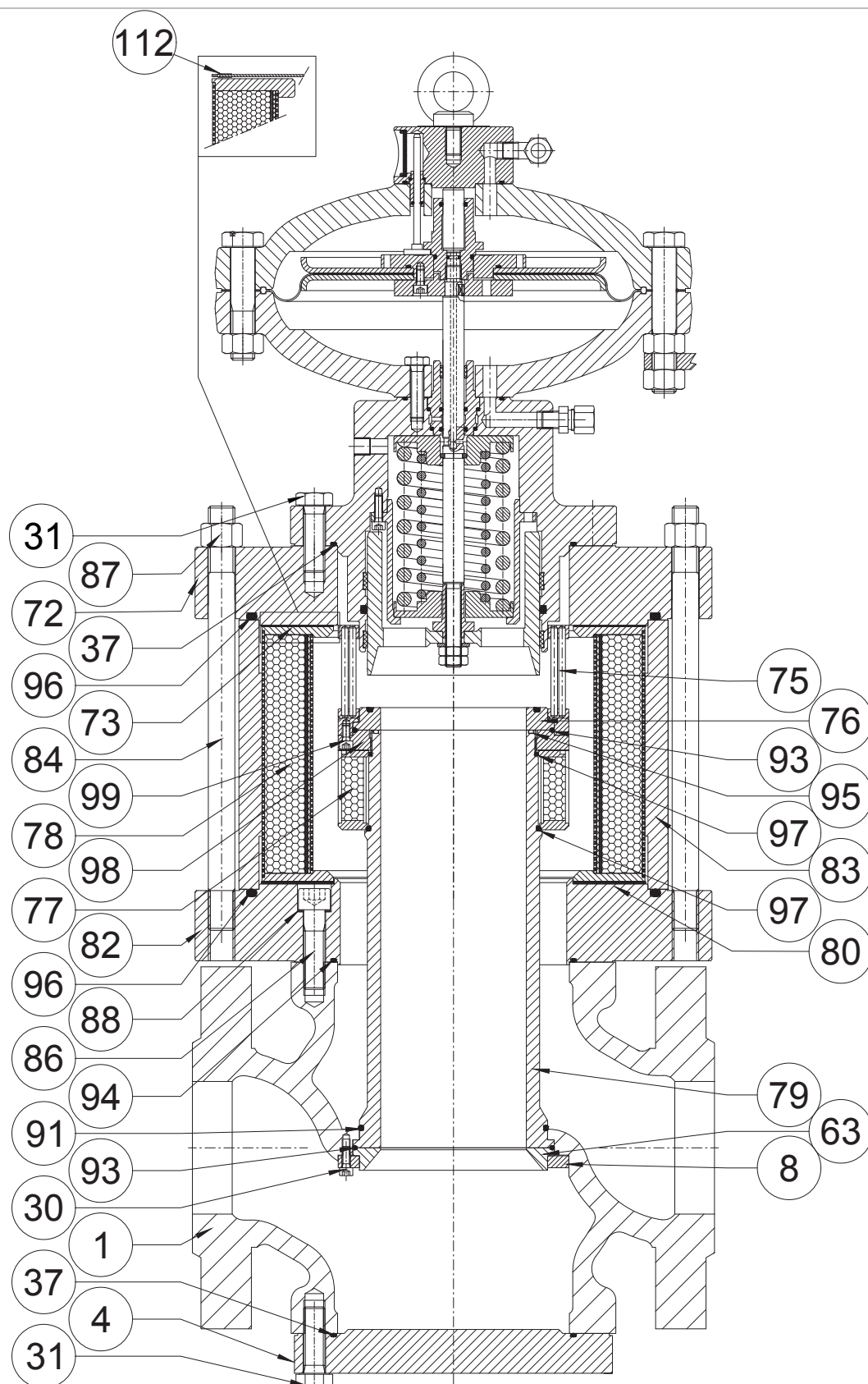
Rys. 9.60. Tłumik DB/819
