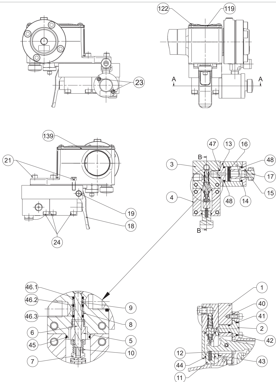
Zawór 3/2
