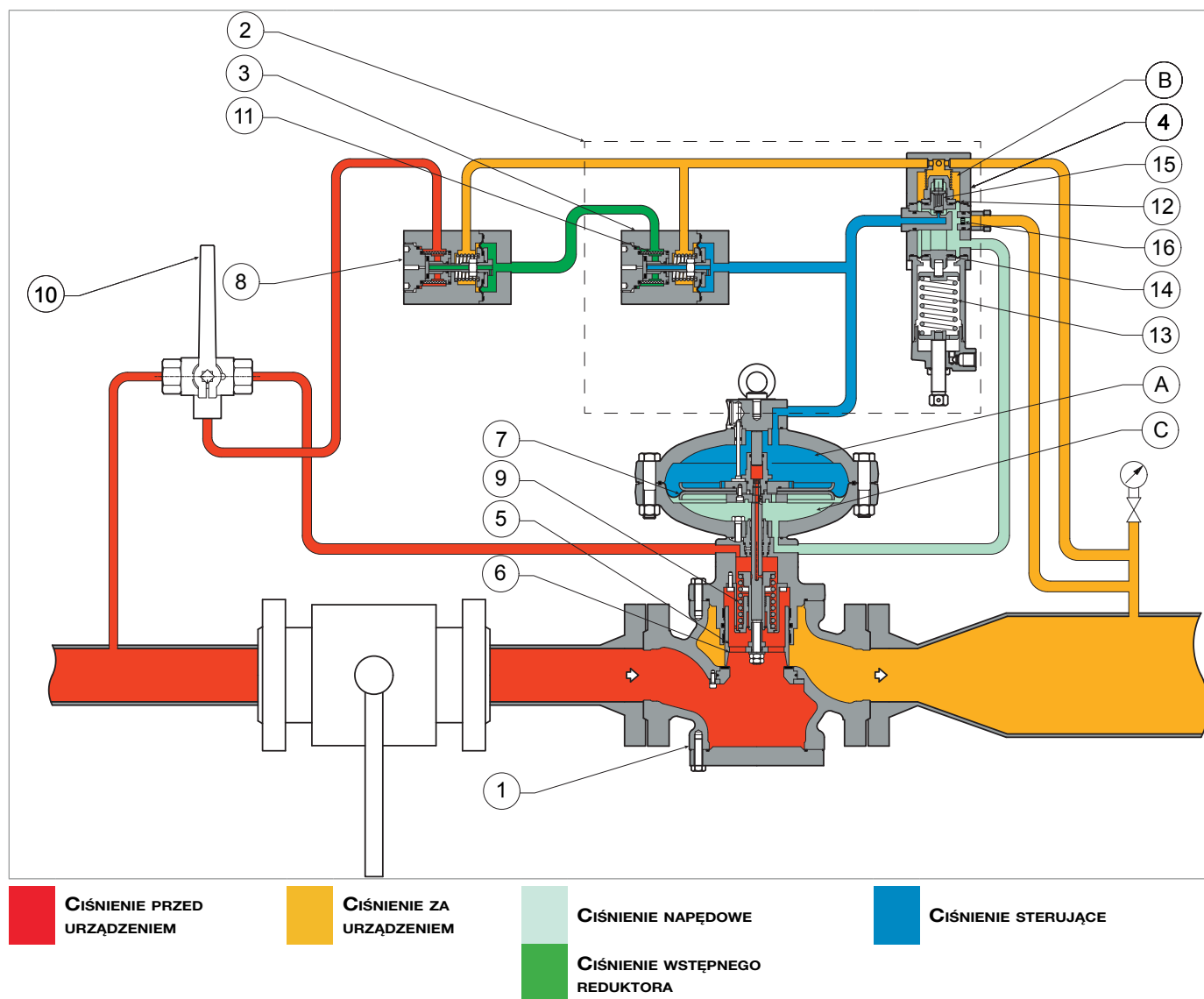
Rys. 4.2. Działanie REFLUX 819/FO
