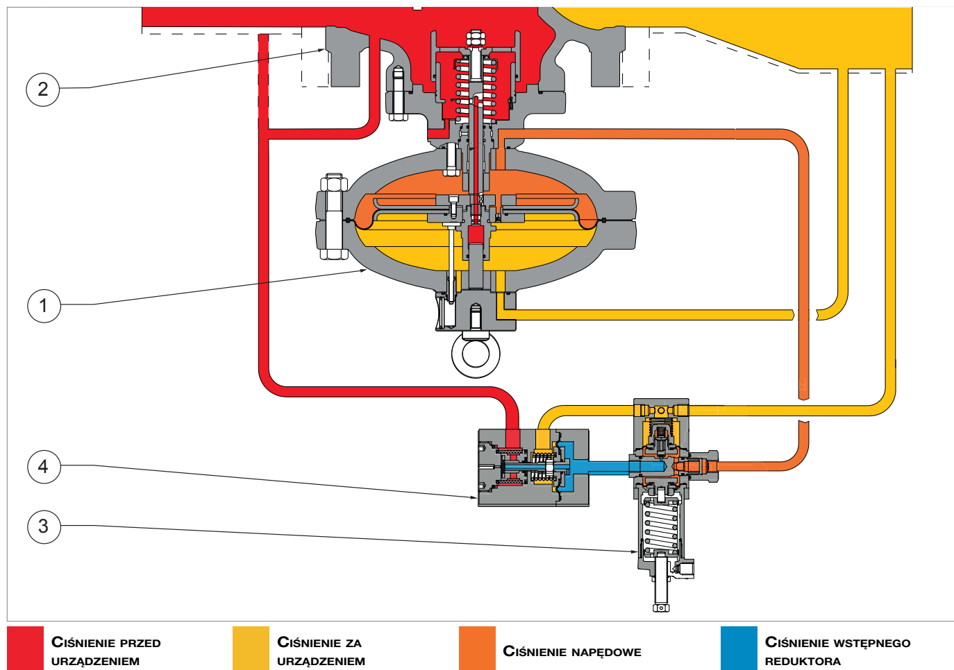
Rys. 4.7. Działanie wbudowanego monitora w trybie czuwania
