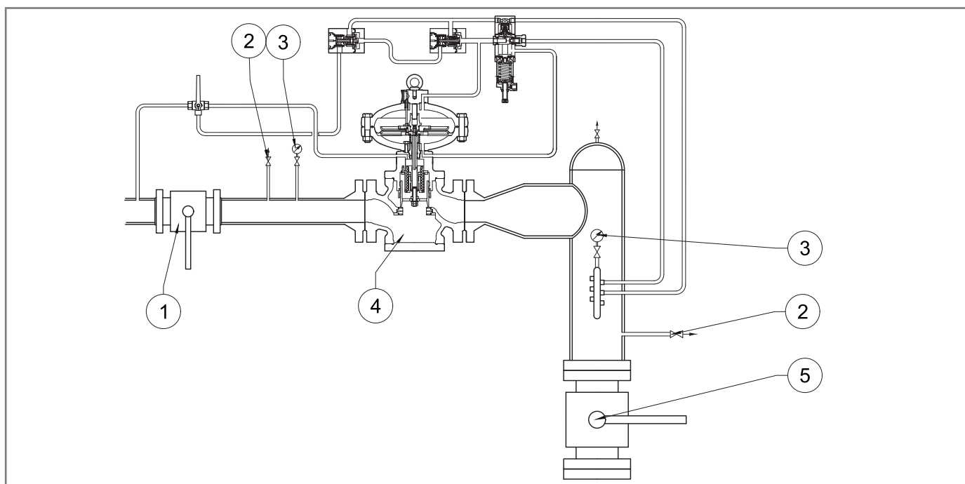
Rys. 6.23. Instalacja zespołu
