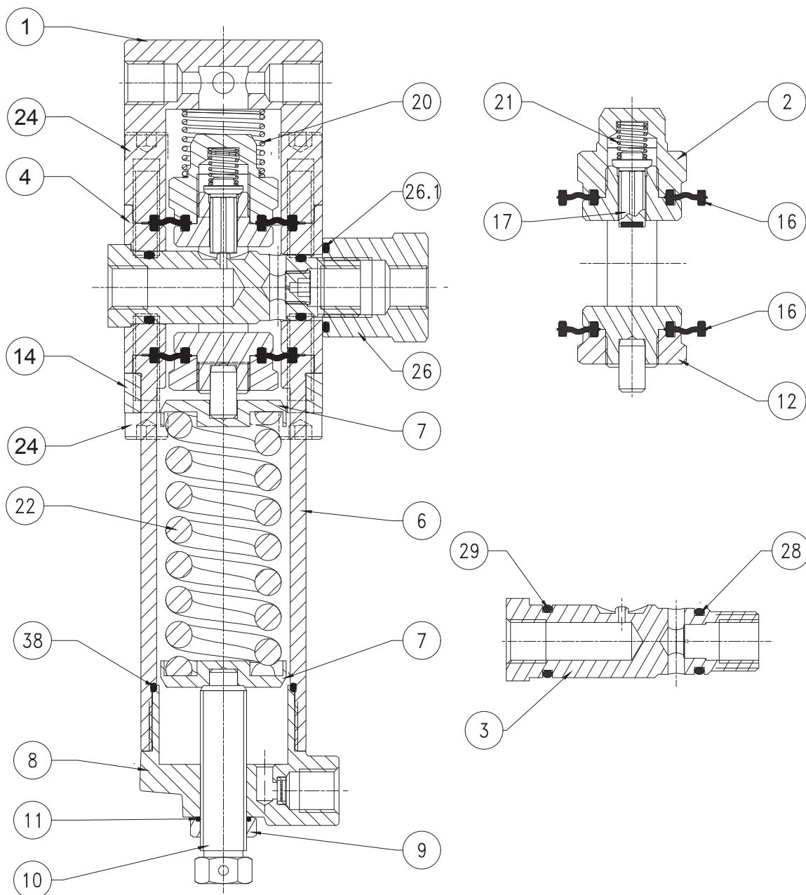
Urządzenie sterujące 207/A/FO i 207/A
