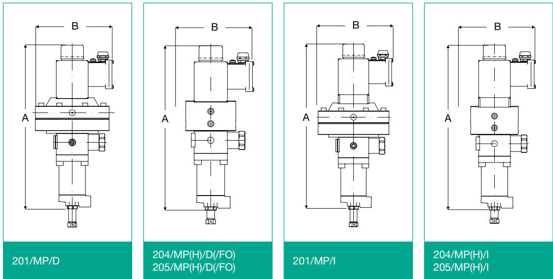
Figura 19 Dimensiones del piloto magnético serie 200/MP
