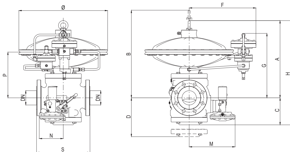
Figure 12 Dimensions Reval 182 + SA
