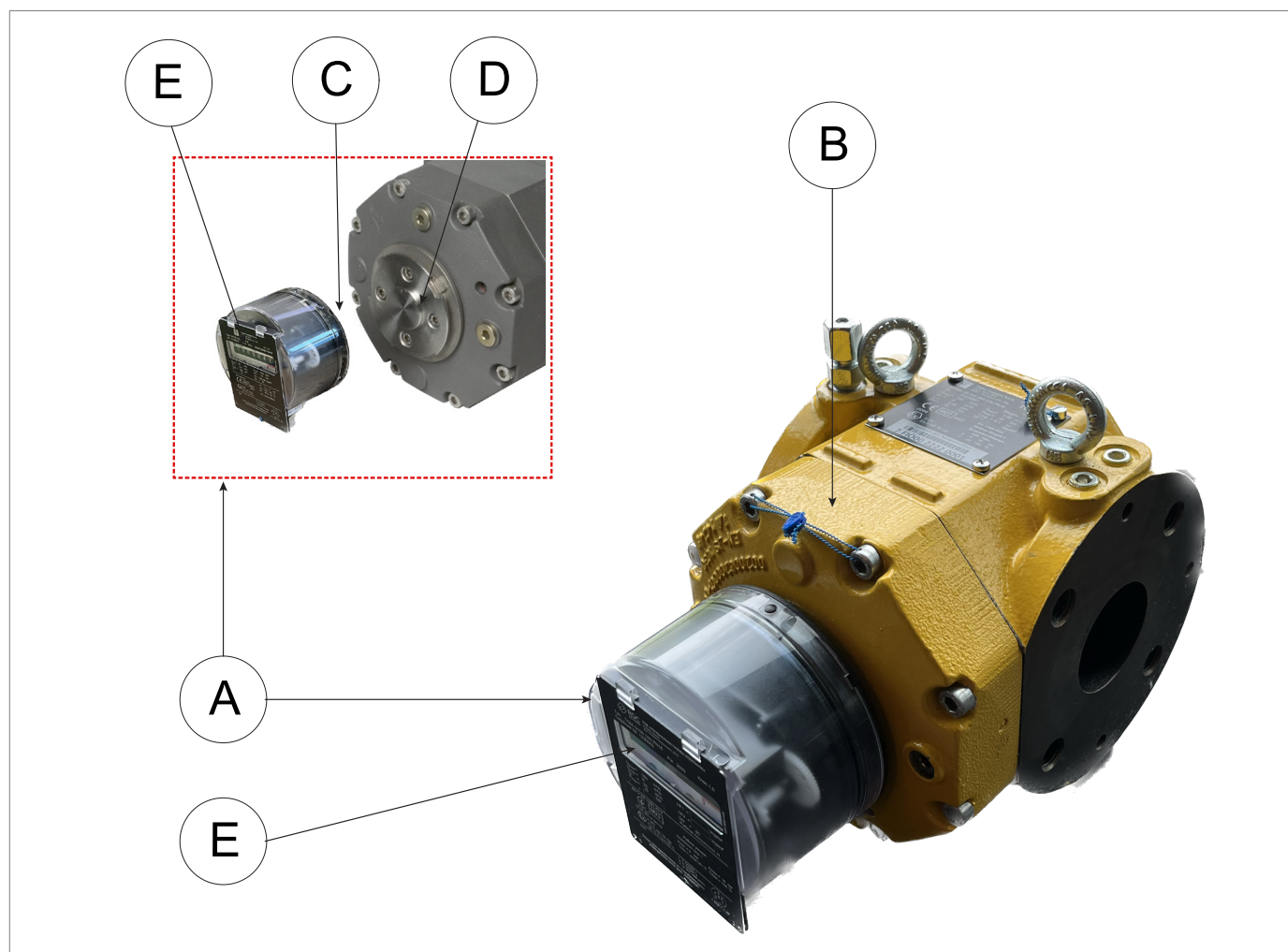
Fig. 4.2. Gruppo totalizzatore
