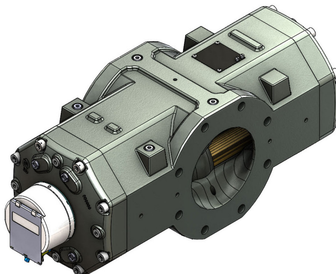
Fig. 4.4. Versione Twin
