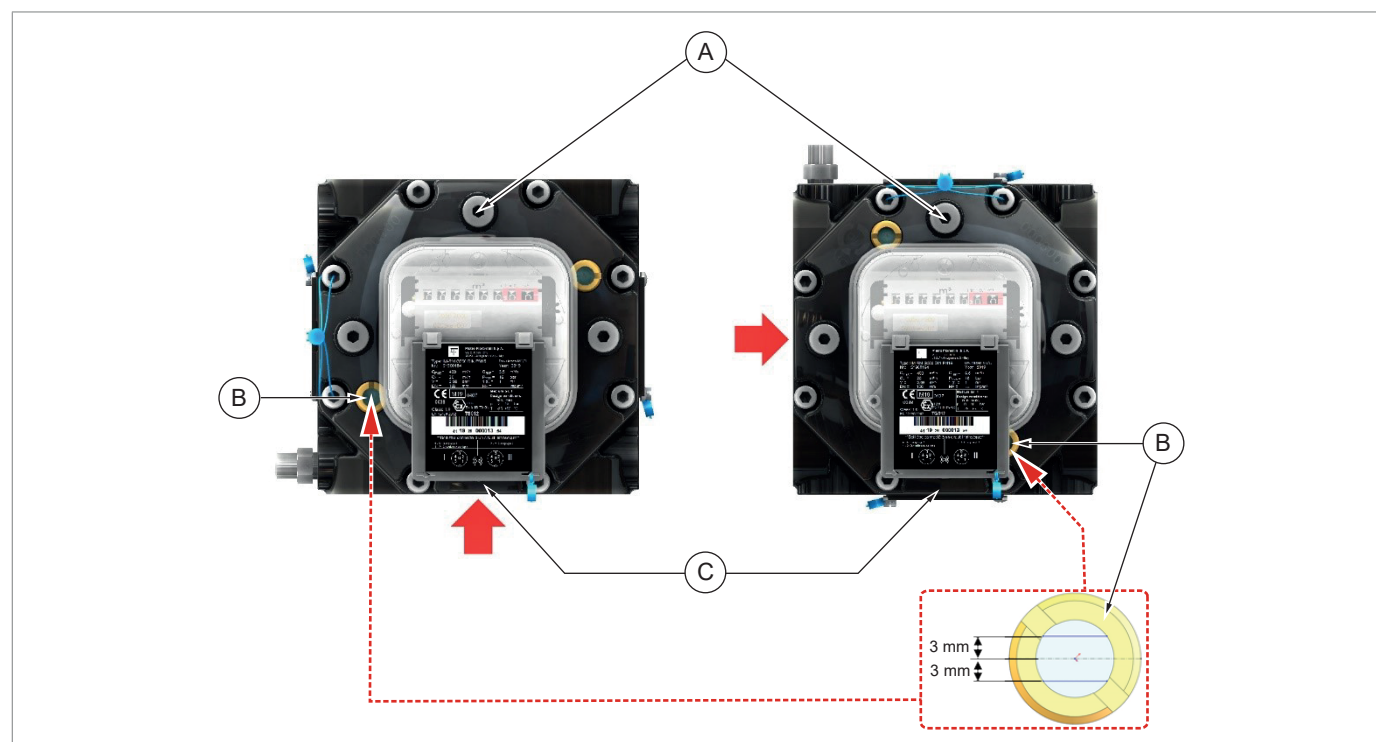
Fig. 6.5. Lubrificazione
