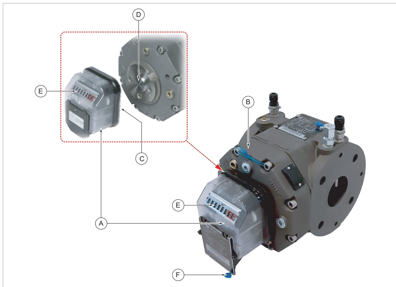
Fig. 4.2. Gruppo totalizzatore
