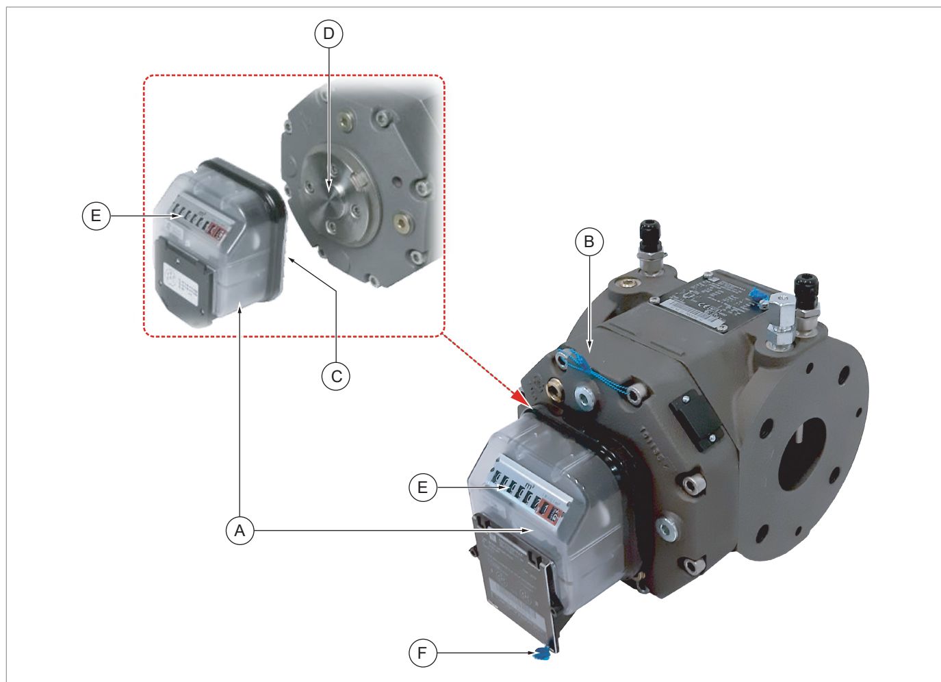
Fig. 4.2. Groupe totalisateur
