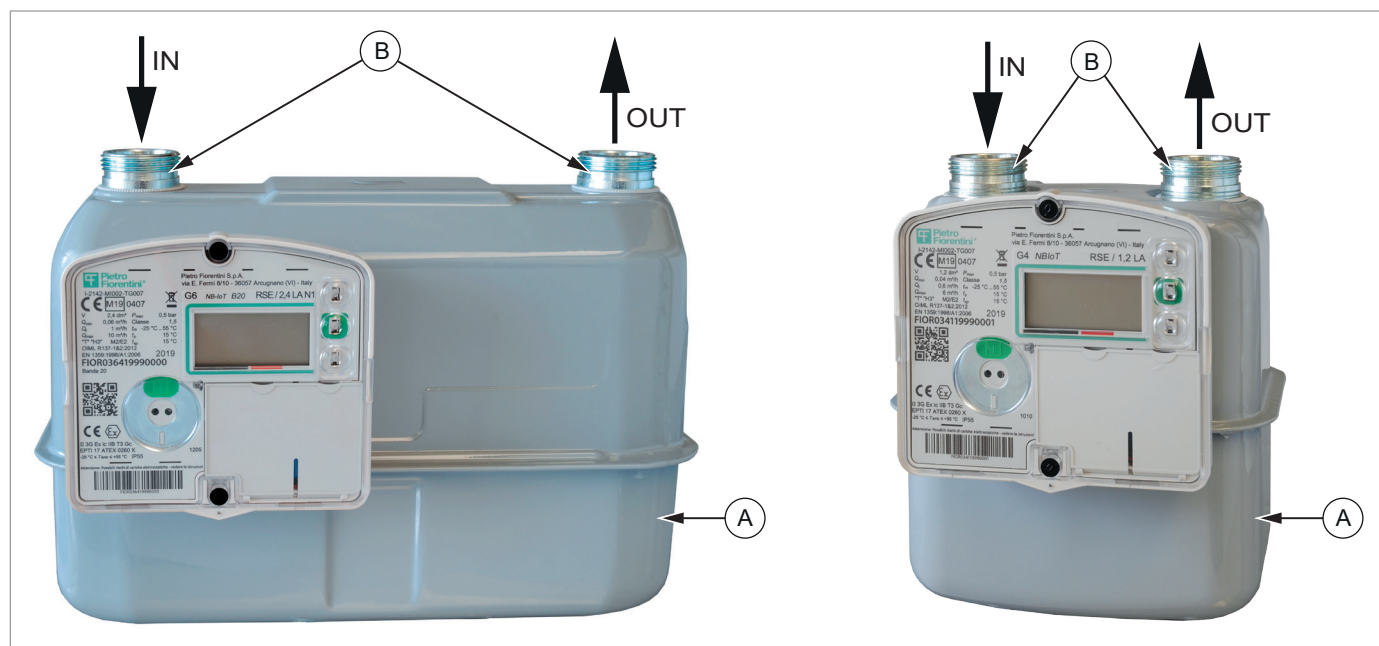
Fig. 7.9. Procedura d'installazione
