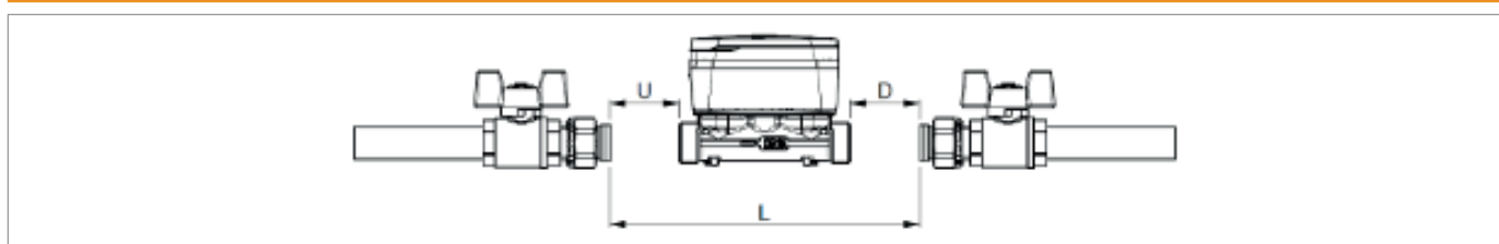
Fig. 7.9. Distance entre le compteur SSM-AQUO et les joints
