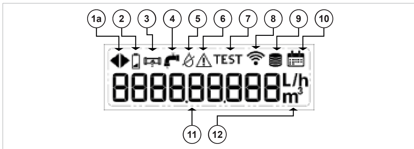
Fig. 5.4. Écran LCD SSM-AQUO (version A)
