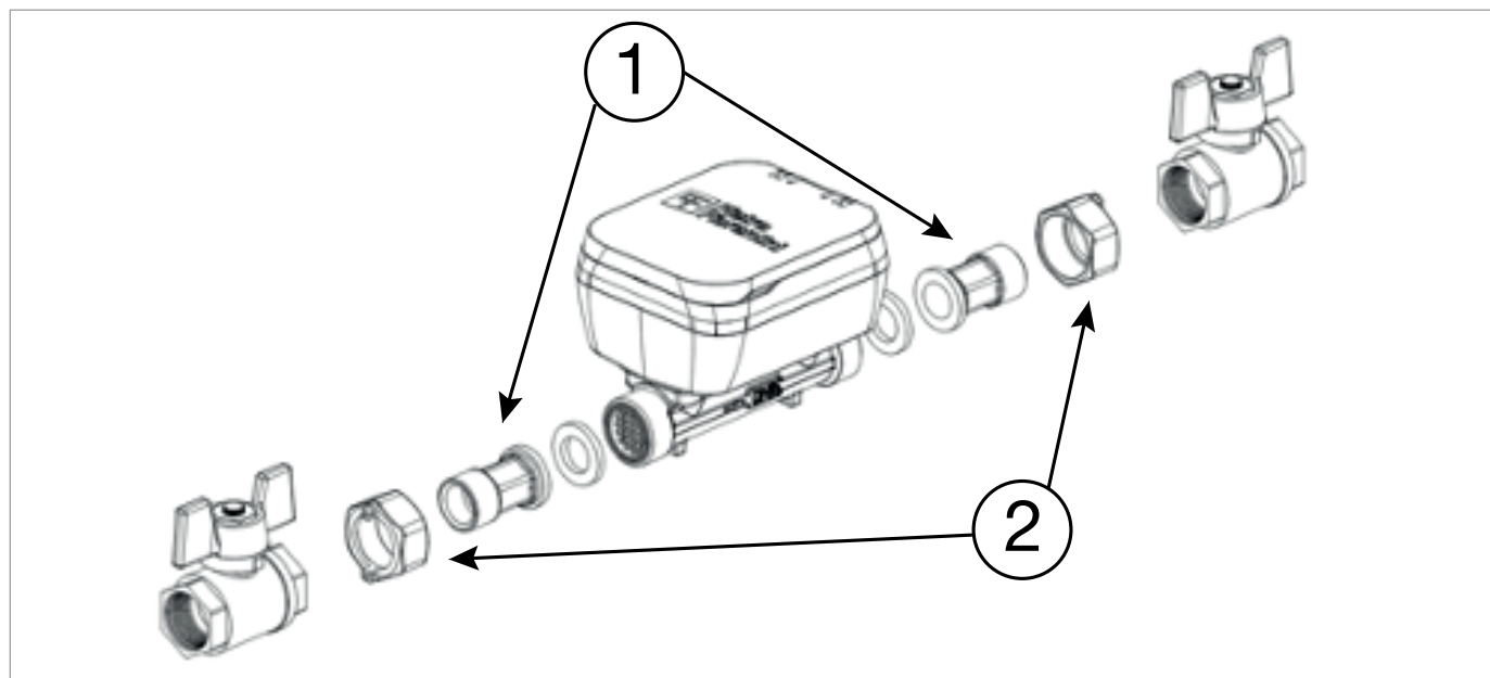
Fig. 7.11. Joints du compteur
