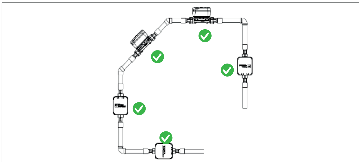
Fig. 7.10. Positions d'installation possibles
