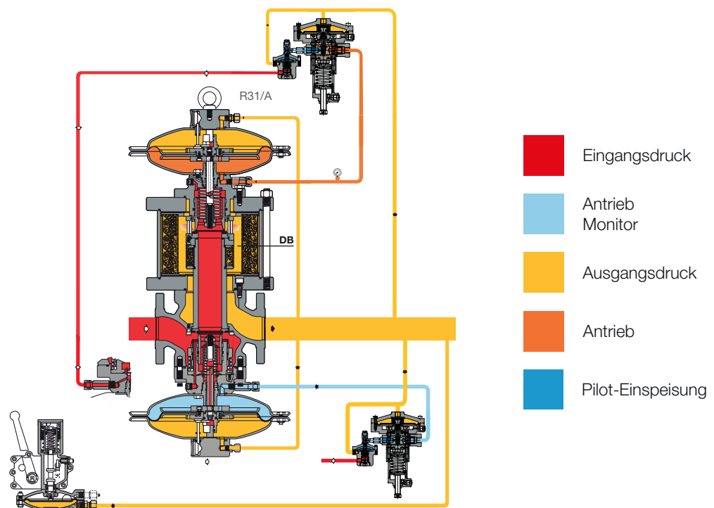
Abbildung 5 Terval/R mit Schalldämpfer DB/182
