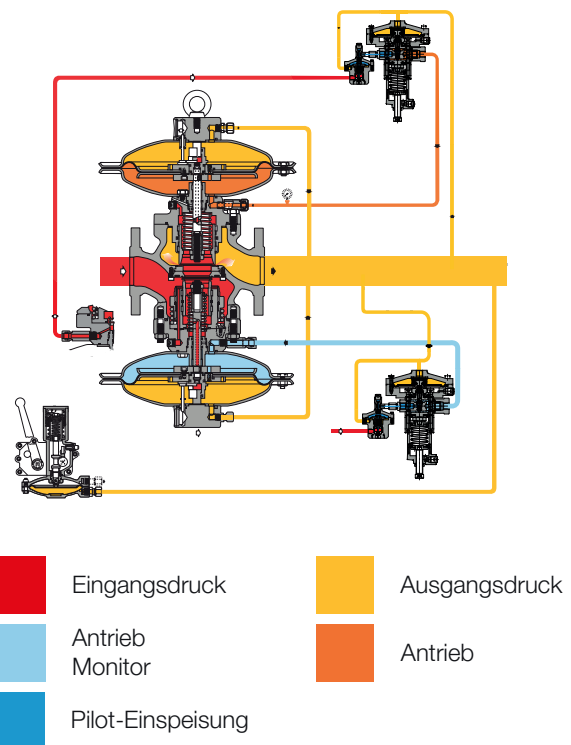
Abbildung 4 Terval/R PM/182
