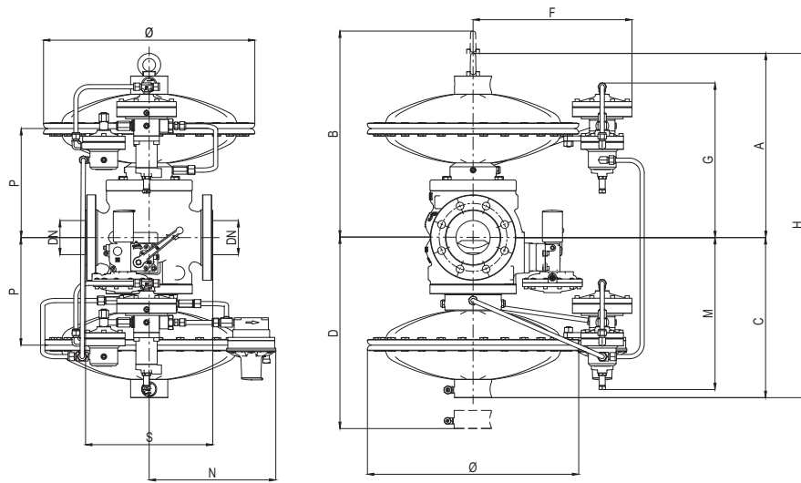
Abbildung 7 Terval/R - Abmessungen
