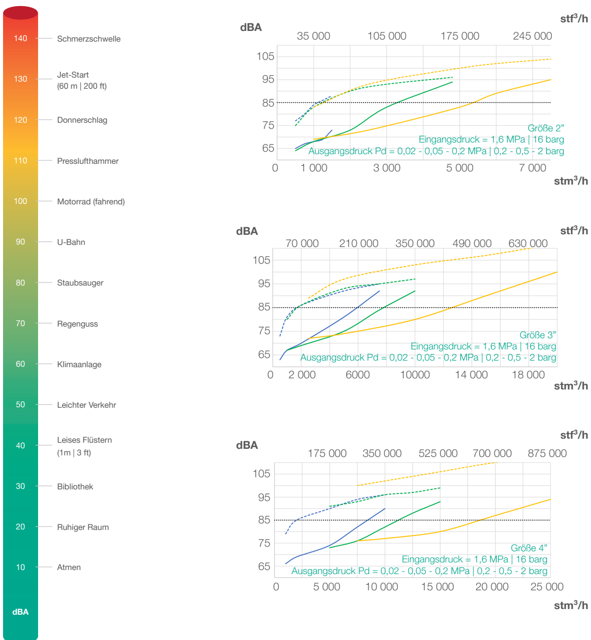
Diagramm 1 Wirksamkeitskurven des Schalldämpfers von Terval/R
