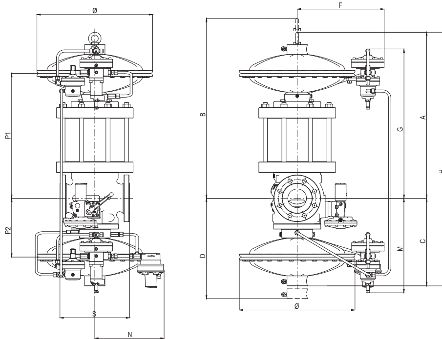
Abbildung 8 Terval/R + DB/182
