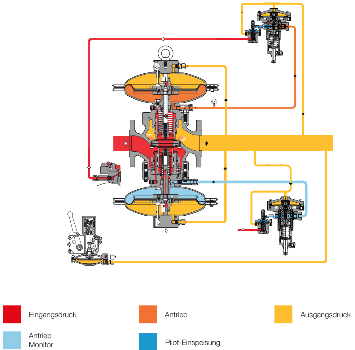
Abbildung 2 Terval/R
