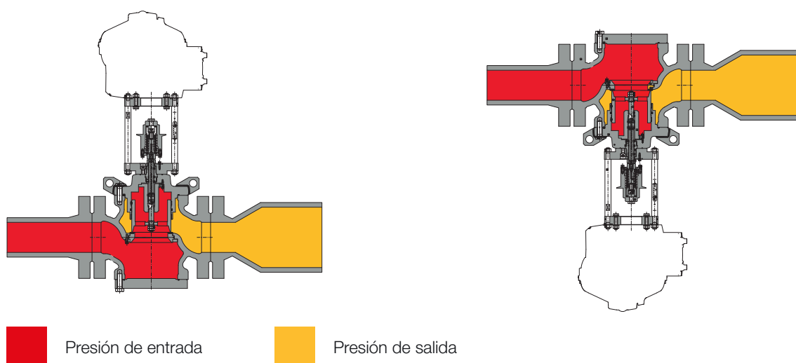
Figura 5 Instalación recomendada para Syncroflux
