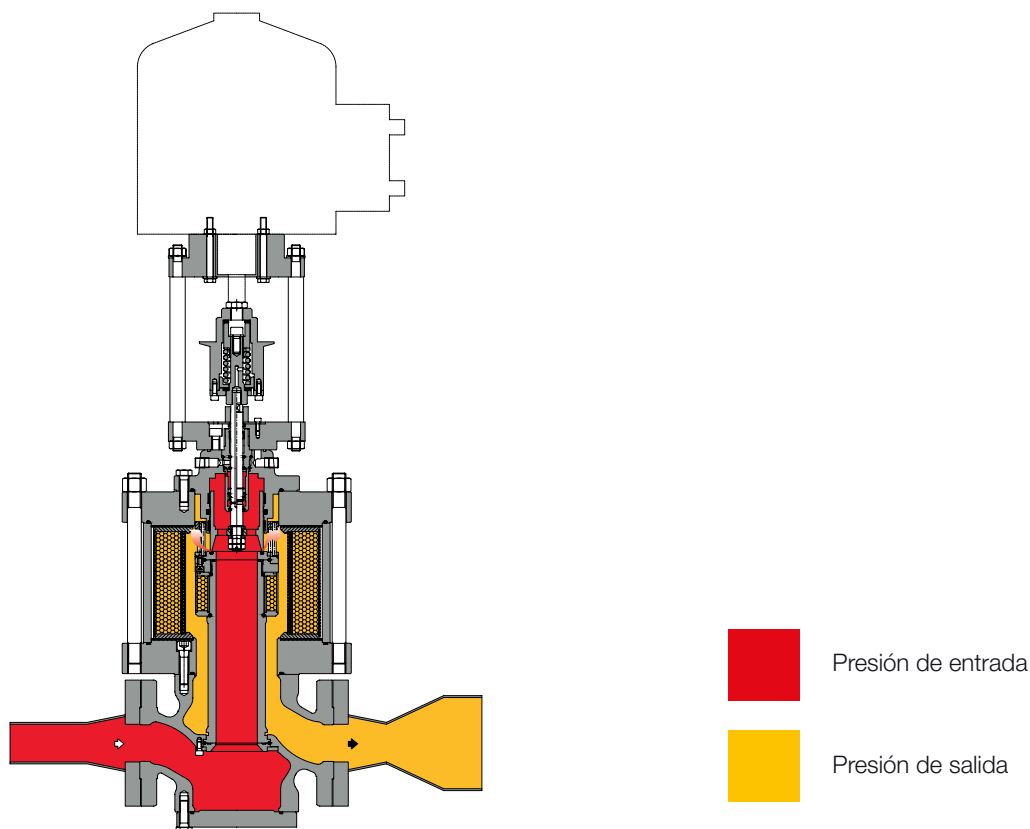
Figura 6 Syncroflux con silenciador DB/819
