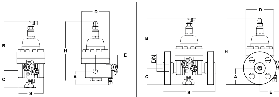
Figura 5 Dimensiones de Staflux Mini
