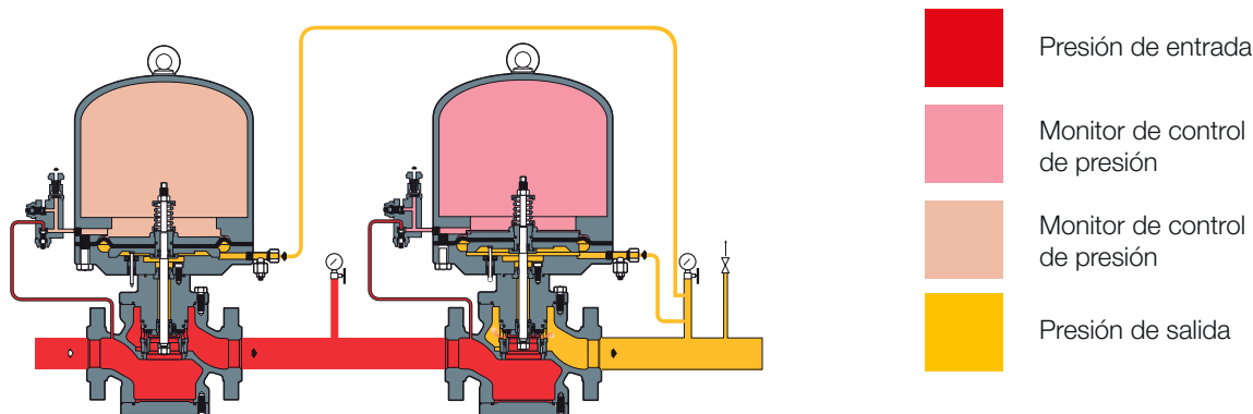
Figura 5 Staflux 185 con configuración de monitor en línea
