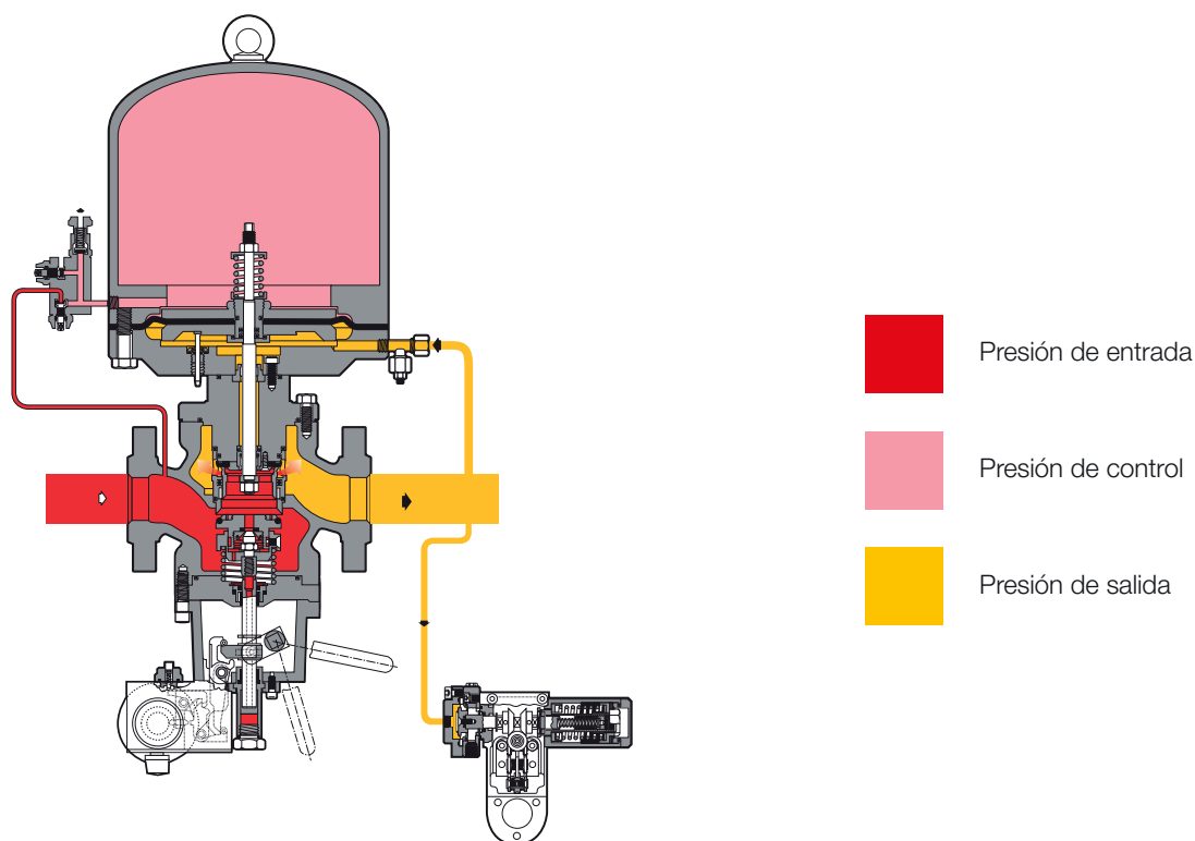
Figura 6 Staflux 185 con SB/185
