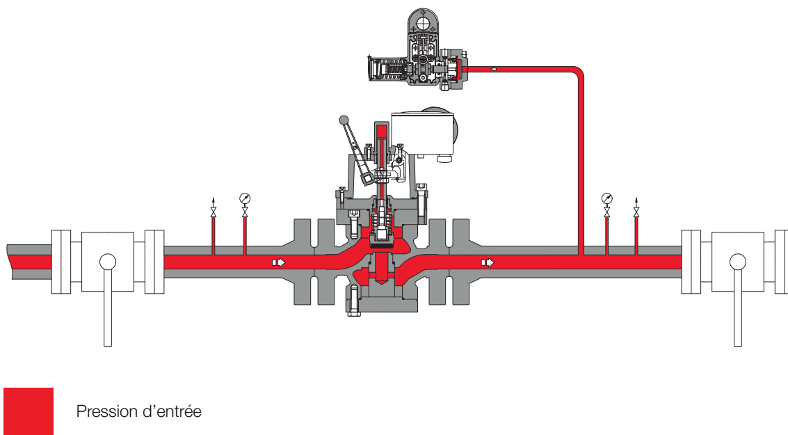
Figure 4 Installation en ligne SBC 187
