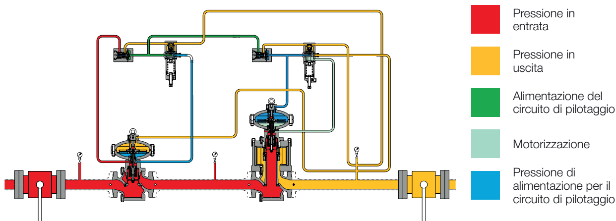
Figura 5 Reflux 819/FO regolatore principale con Reflux 819 monitor in linea
