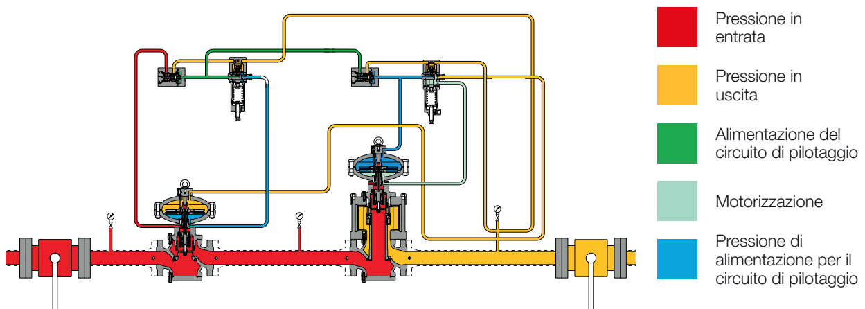
Figura 5 Reflex 819/FO regolatore principale con Reflex 819 monitor in linea
