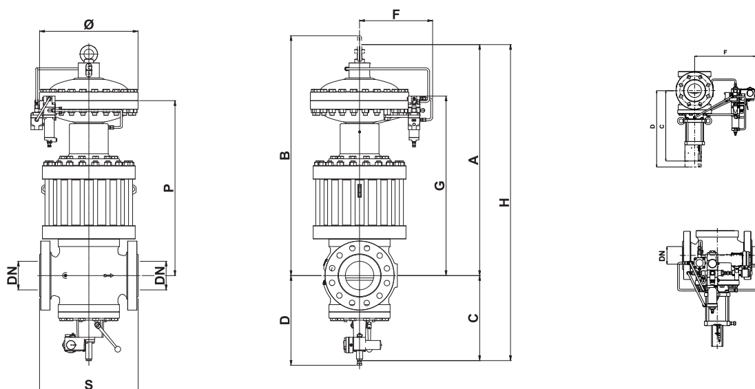
Figure 15 Dimensions du Reflux 819/FO + DB/819 + SB/82 ou HB/97
