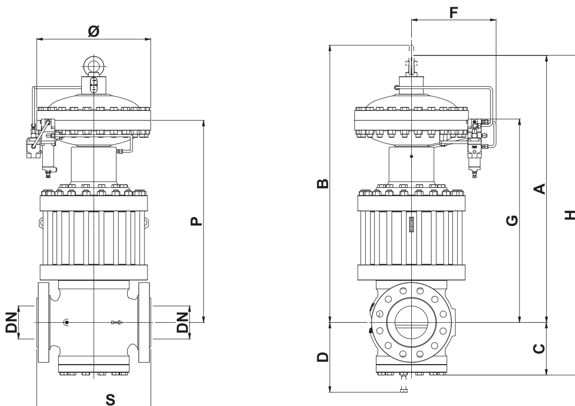
Figure 14 Dimensions du Reflux 819/FO + DB/819
