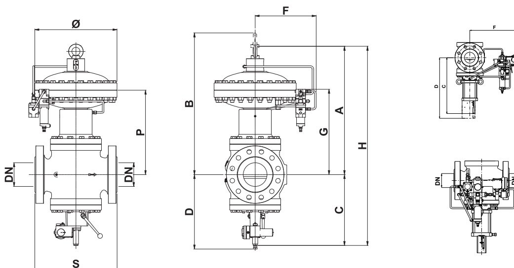
Figure 12 Dimensions du Reflux 819/FO + SB/82 ou HB/97
