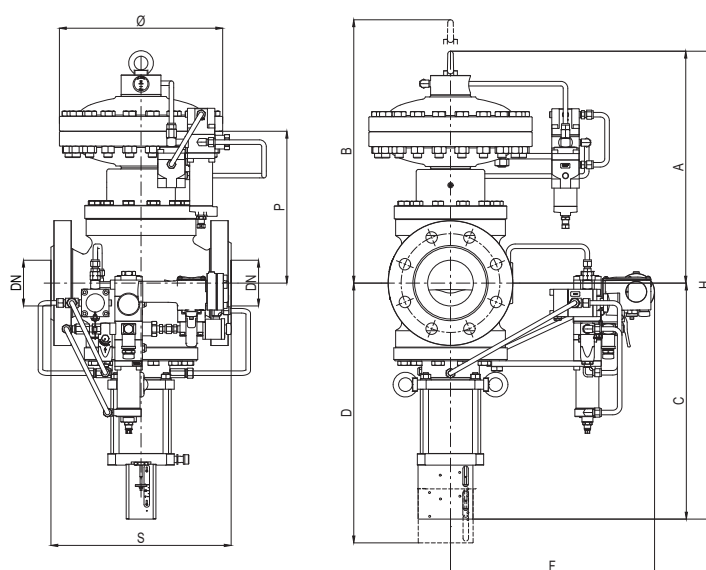
Figure 11 Dimensions du Reflux 819/FO
