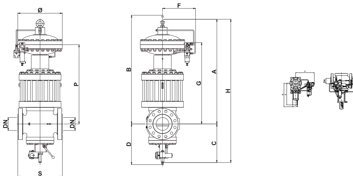
Abbildung 14 Reflux 819/FO + DB/819 + SB/82 oder HB/97 Maße
