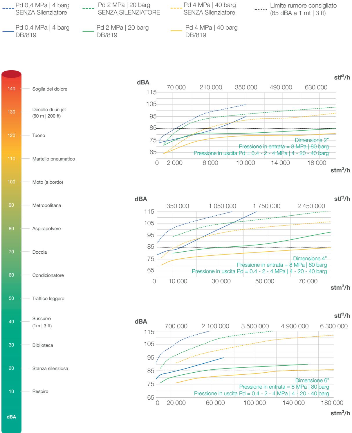
Grafico 1 Grafici di efficienza del silenziatore Reflux 819
