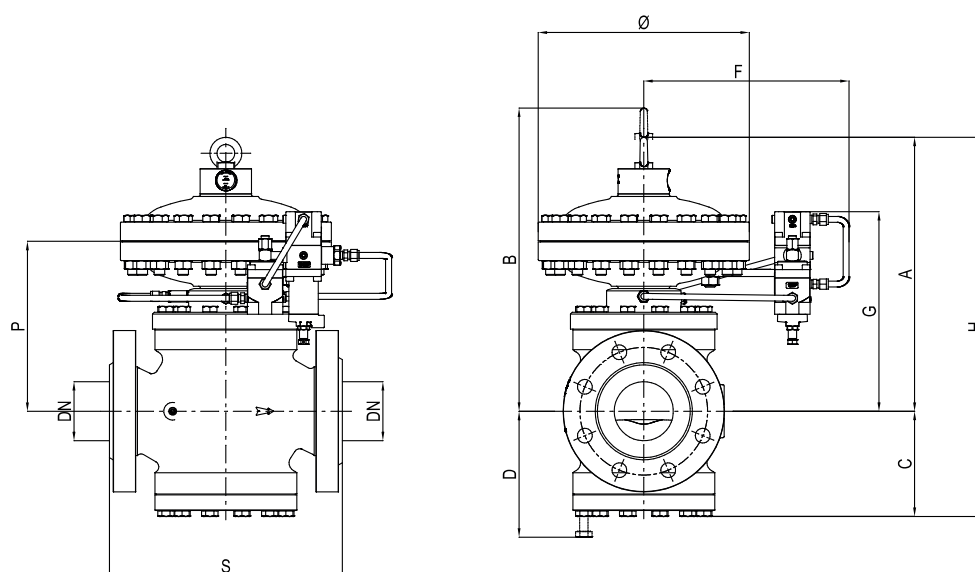
Figura 11 Dimensioni Reflux 819
