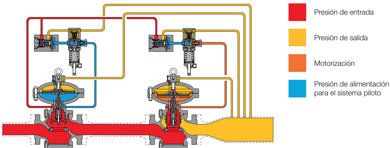
Figura 5 Monitor en línea de Reflux 819
