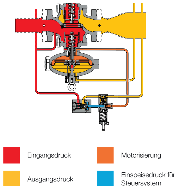
Abbildung 6 Reflux 819 mit SB/819
