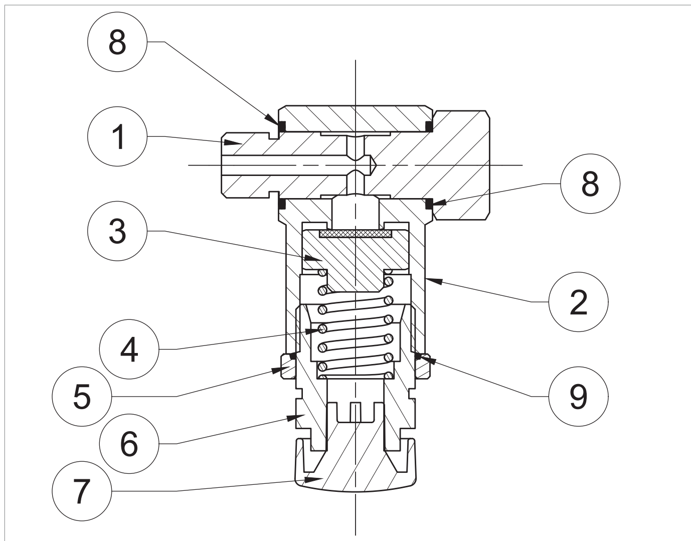
Fig. 9.83. Válvula de seguridad VS/FI para LINE OFF 2.0
