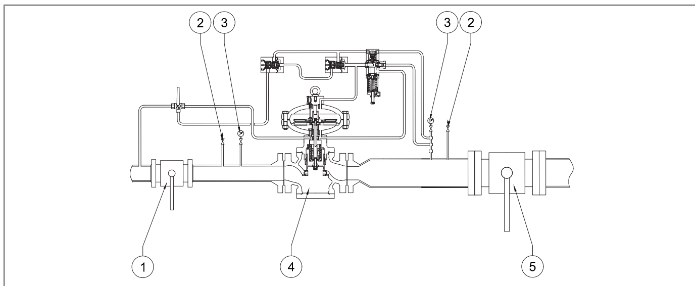
Fig. 6.22. Instalación en línea
