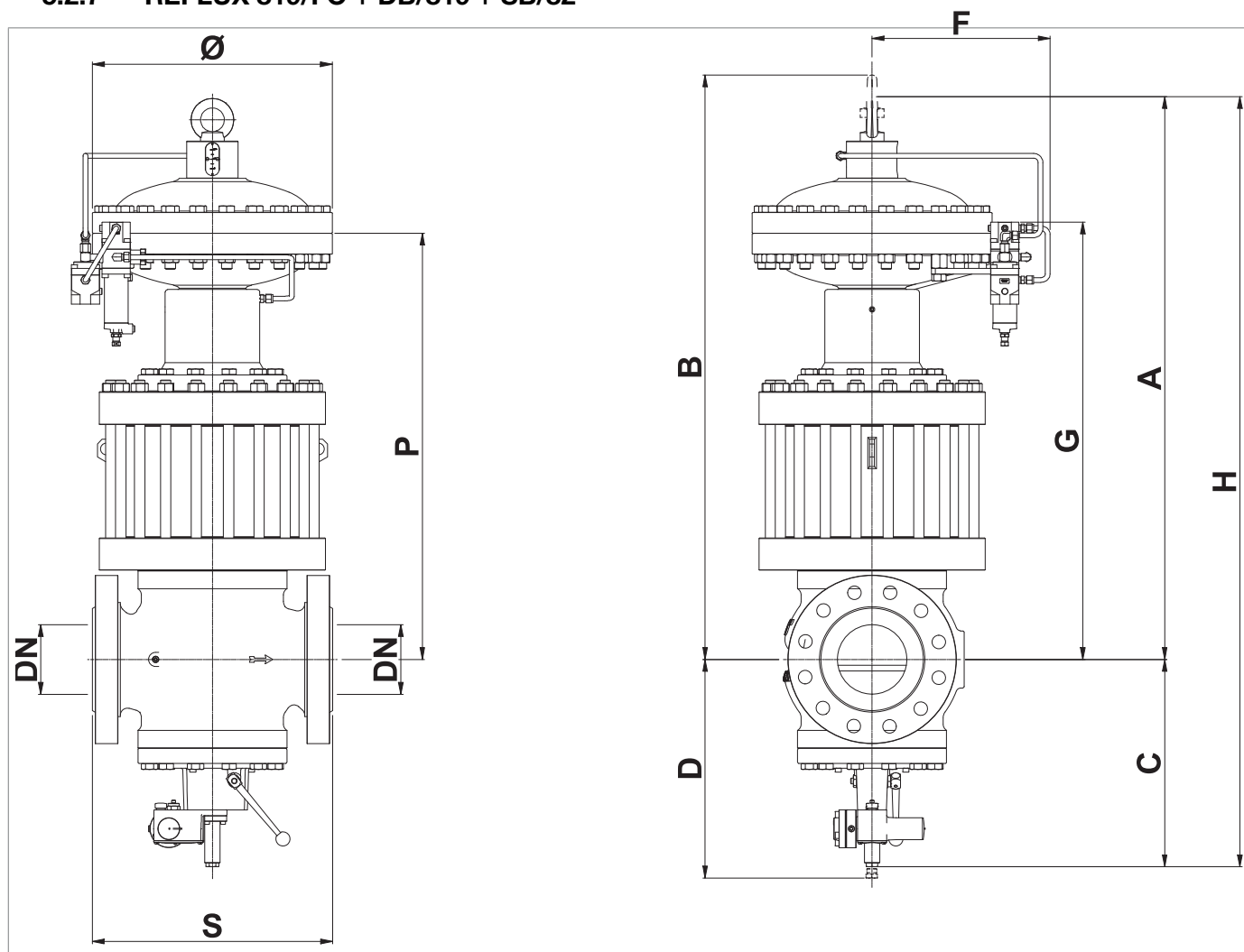
Fig. 5.20. Características físicas REFLUX 819/FO + DB/819 + SB/819
