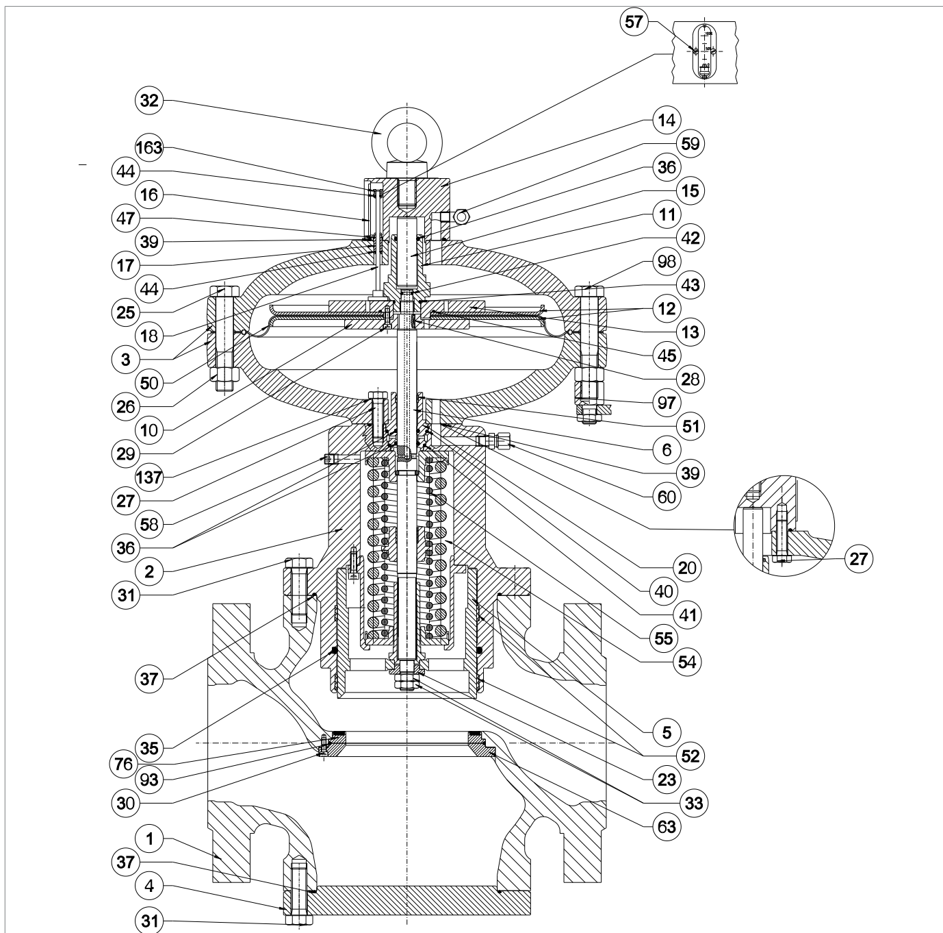
Fig. 9.57. Regulador REFLUX 819/FO 4" ÷ 8"
