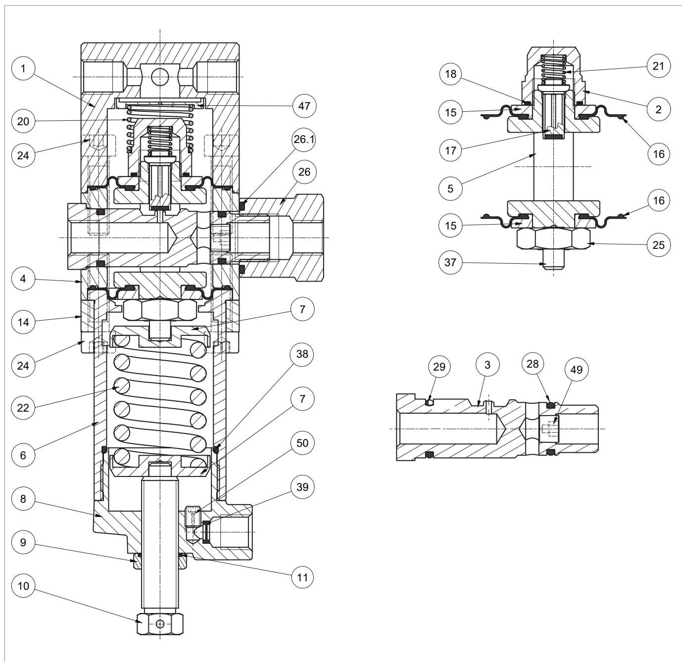
Fig. 9.65. Piloto 204/A/FO-204/A y 205/A/FO-205/A
