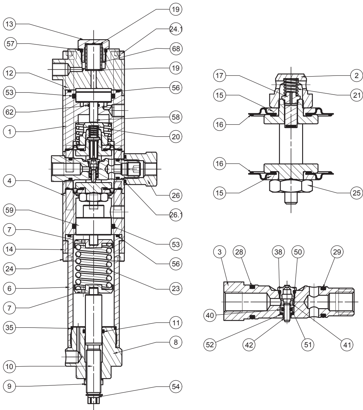
Regulador de presión R44/SS
