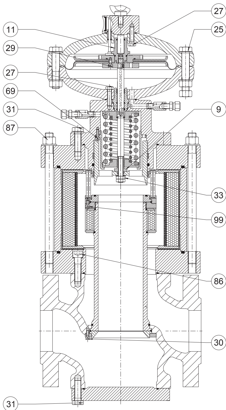
Pares de apriete REFLUX 819/FO + Silenciador DB/819
