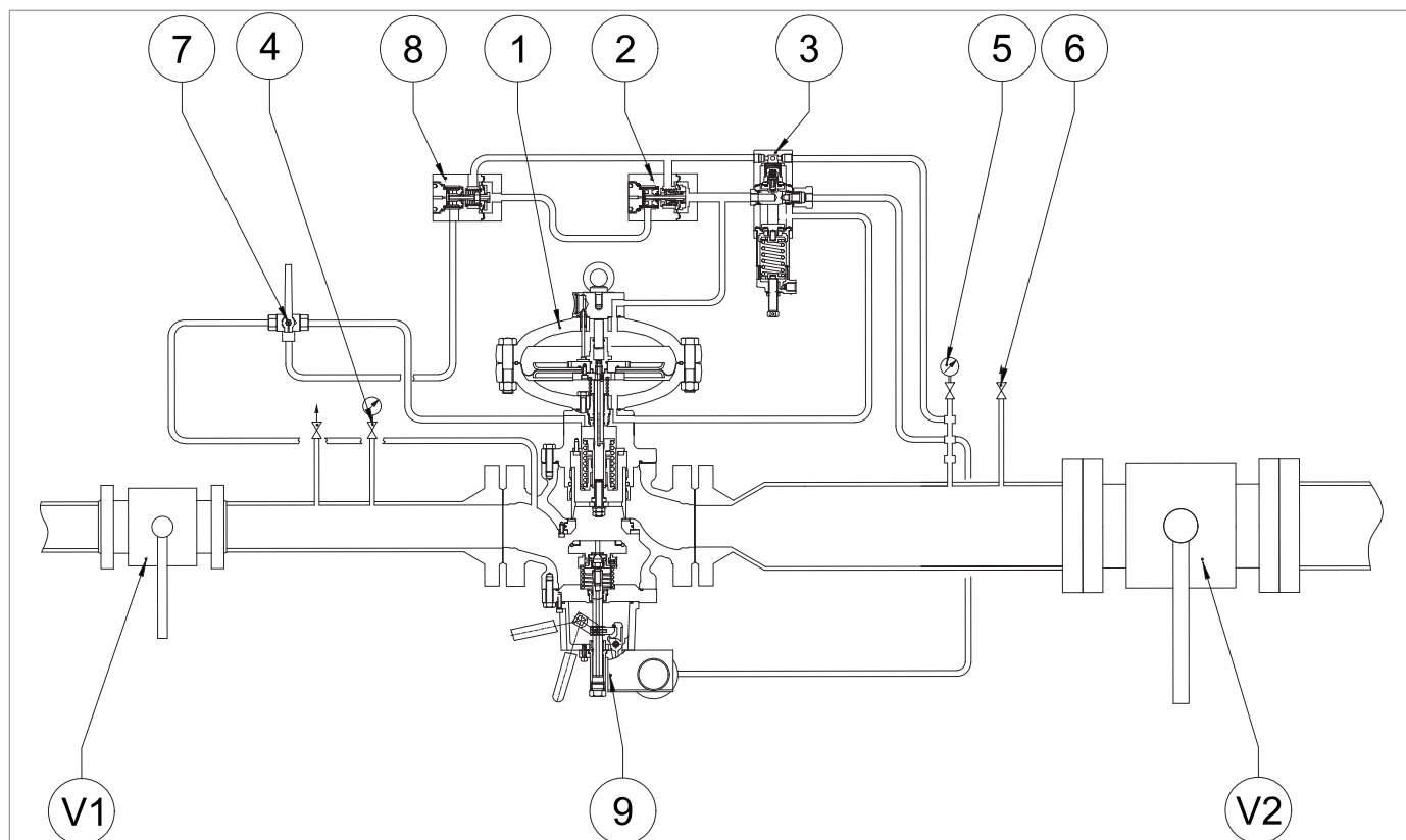
Fig. 8.32. Estanqueidad de la válvula de bloqueo incorporada SB/82
