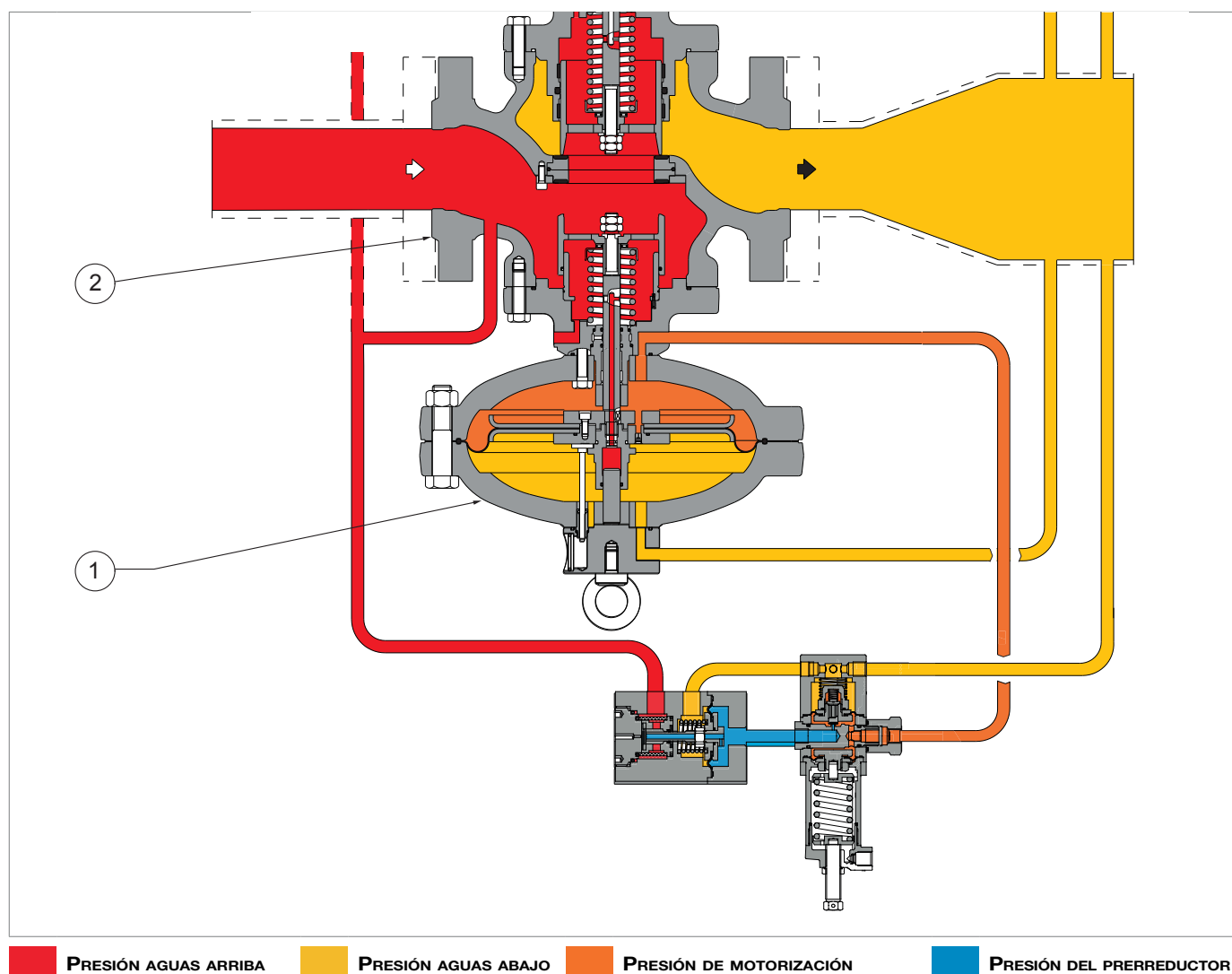
Fig. 4.5. REFLEX 819/FO con monitor PM/819
