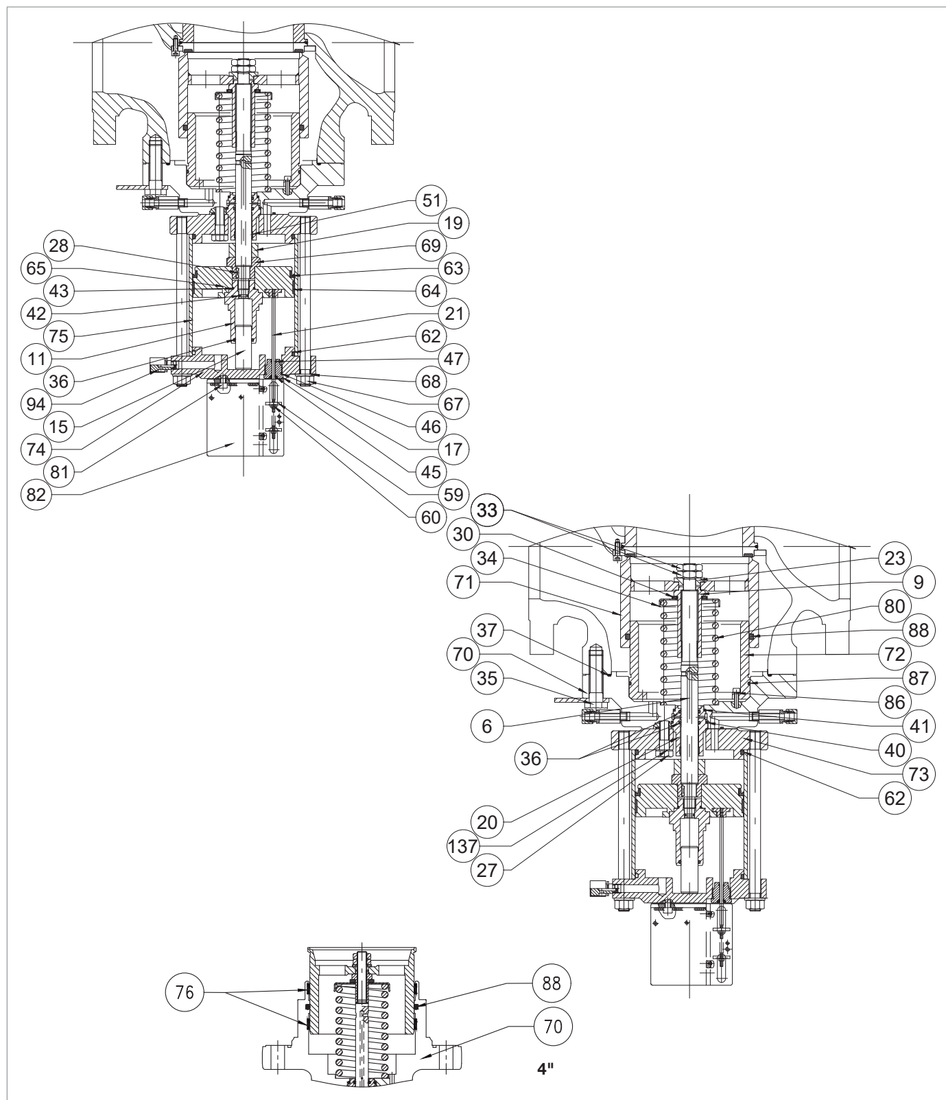
Fig. 9.78. Válvula de bloqueo incorporada HB/97
