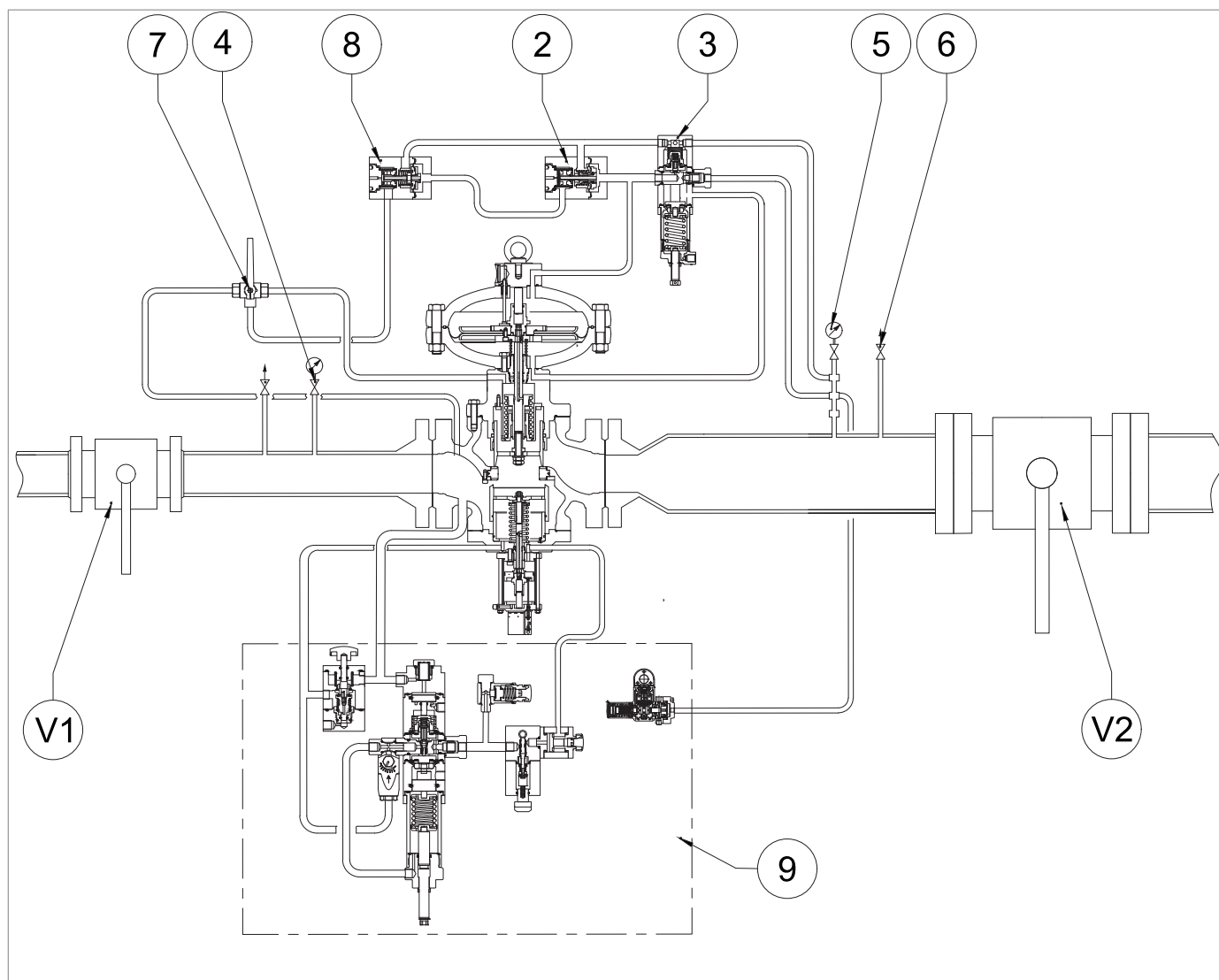
Fig. 8.35. Estanqueidad de la válvula de bloqueo incorporada HB/97
