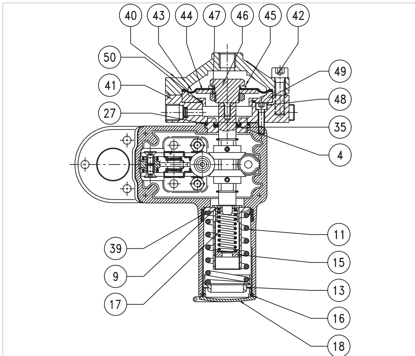
Fig. 9.75. Presostato Mod. 102M/102MH
