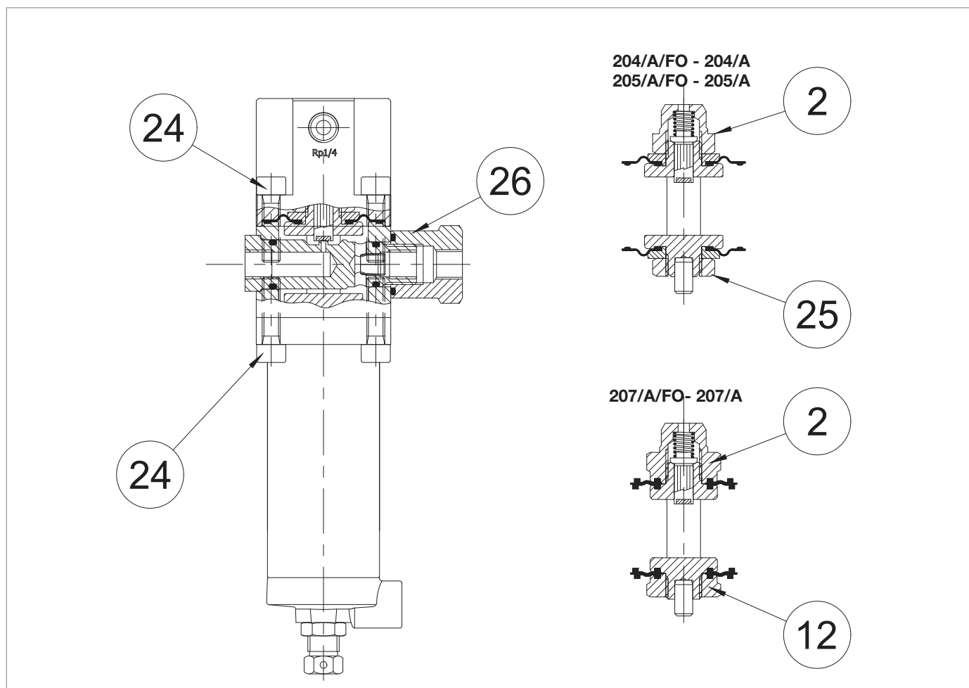
Fig. 9.42. Pares de apriete pilotos serie 200/A y 200/A/FO
