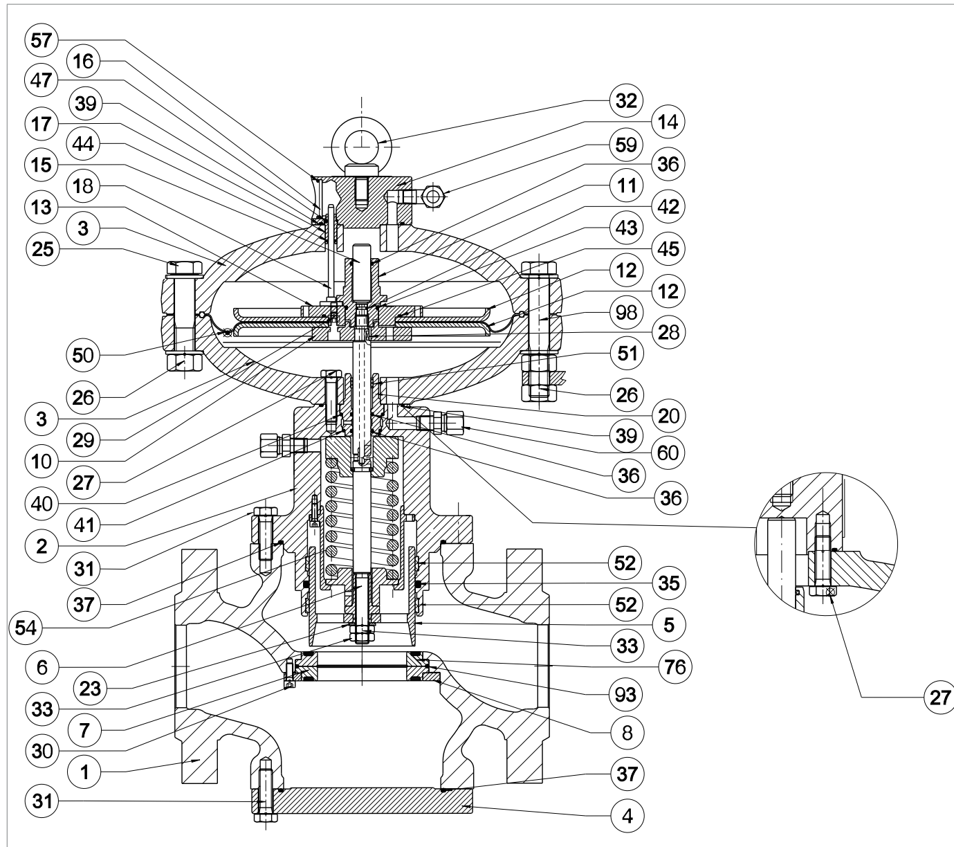
Regulador REFLUX 819/FO 2" ÷ 3"
