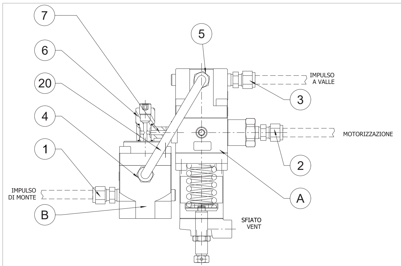
Fig. 9.69. Piloto serie 200/A y R14/A
