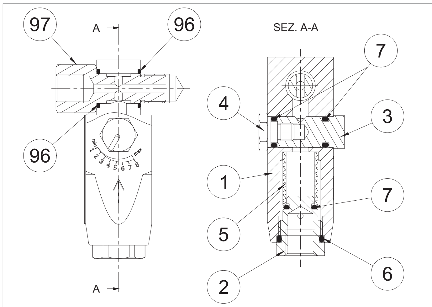
Fig. 9.81. Válvula de laminación AR100
