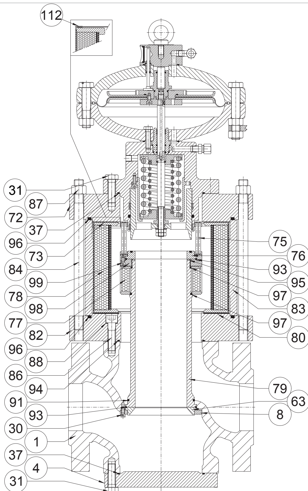
Fig. 9.60. Silenciador DB/819
