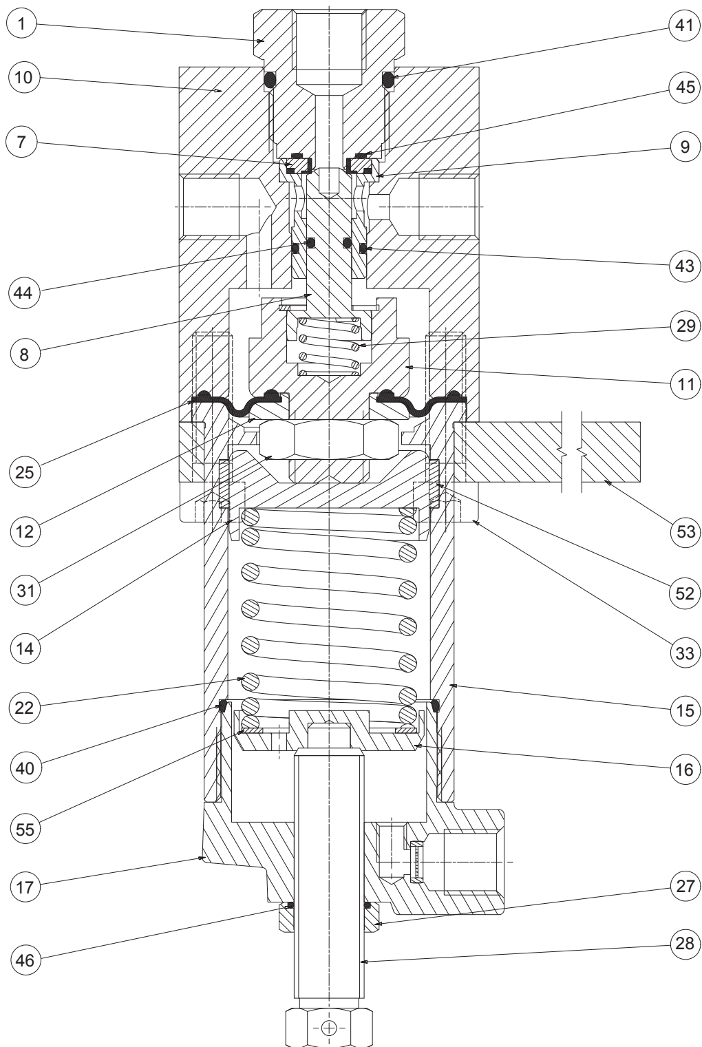
Válvula aceleradora M/A
