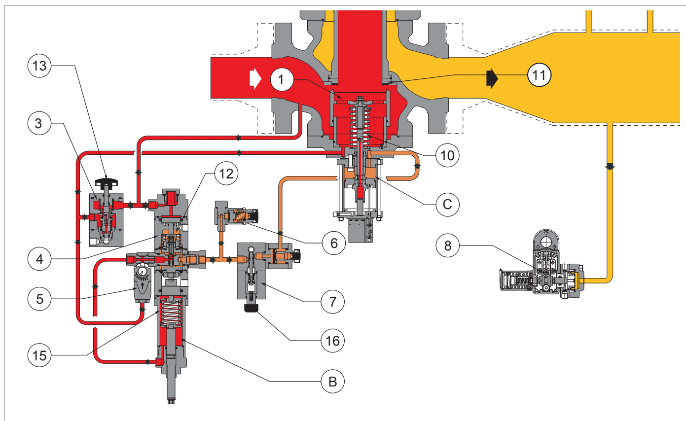
Fig. 4.12. REFLUX 819/FO con válvula de bloqueo incorporada HB/97
