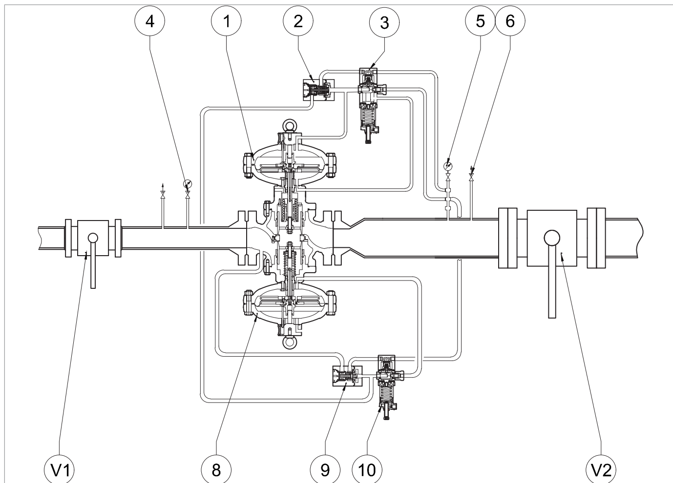
Fig. 8.30. Puesta en servicio del regulador PM/819 con monitor integrado
