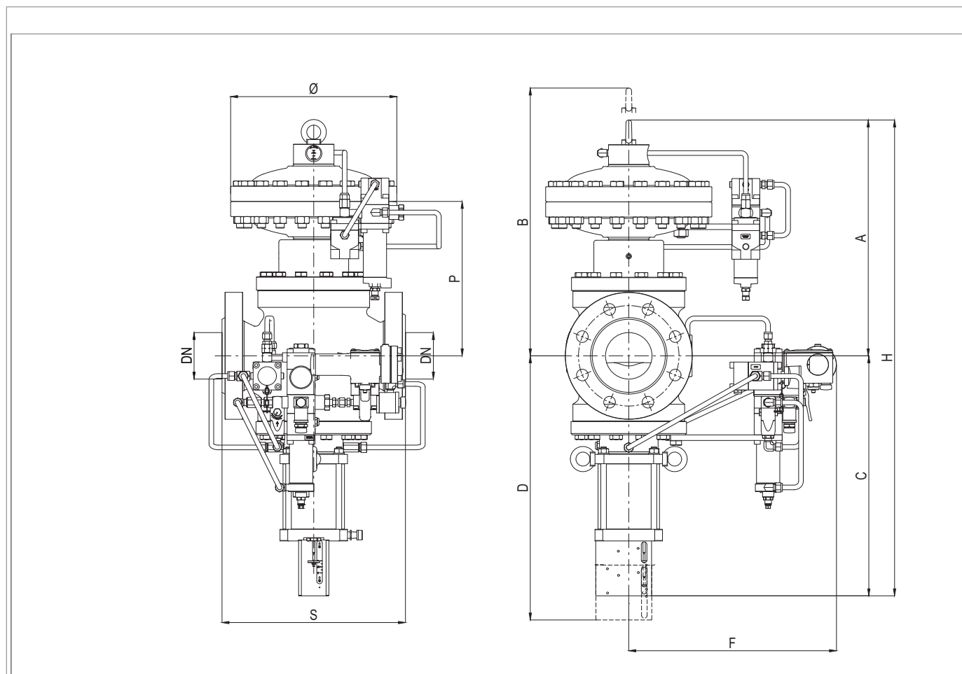
Fig. 5.14. Características físicas REFLUX 819/FO (+LDB/171)
