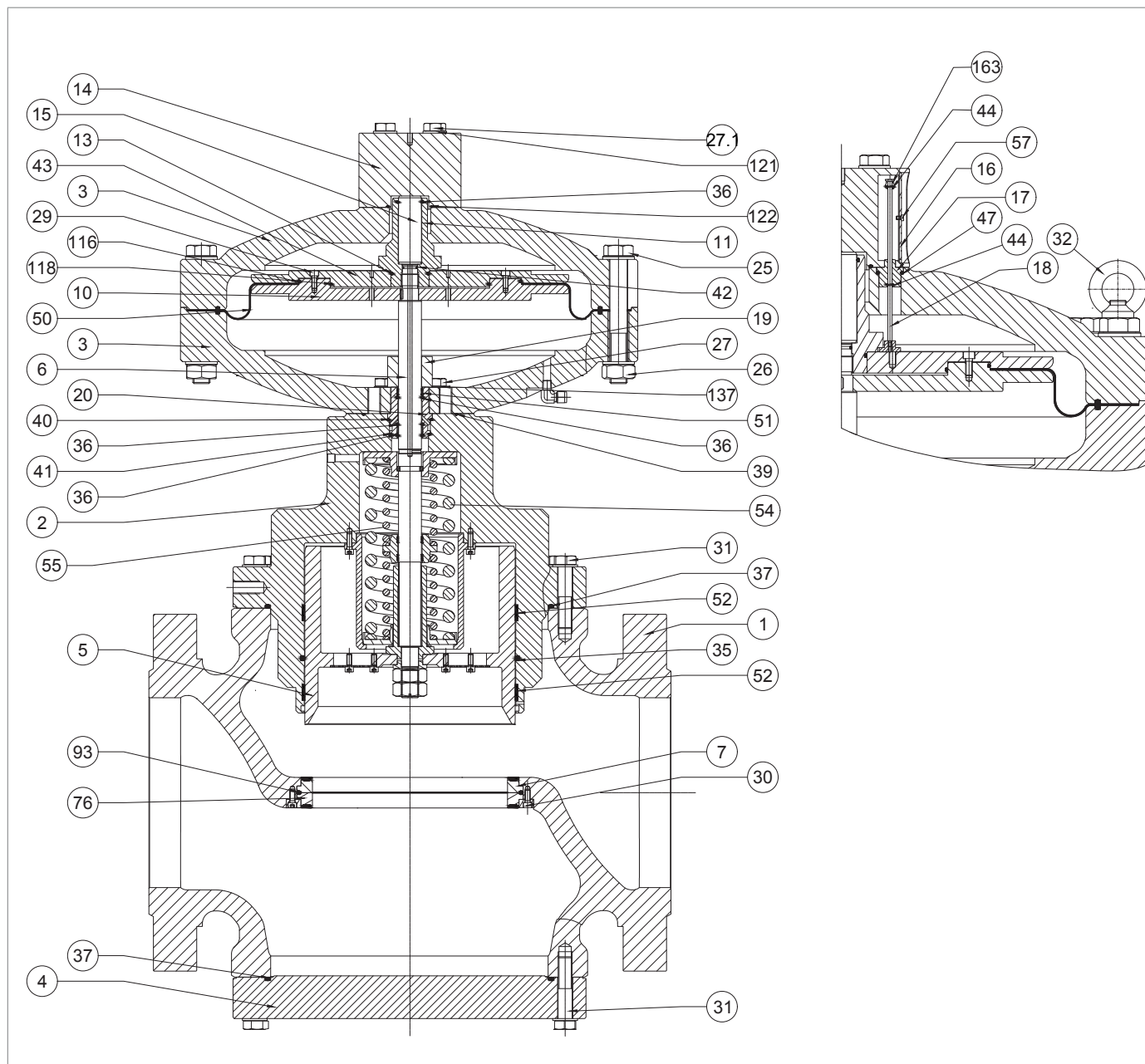
Regulador REFLEX 819/FO 12"
