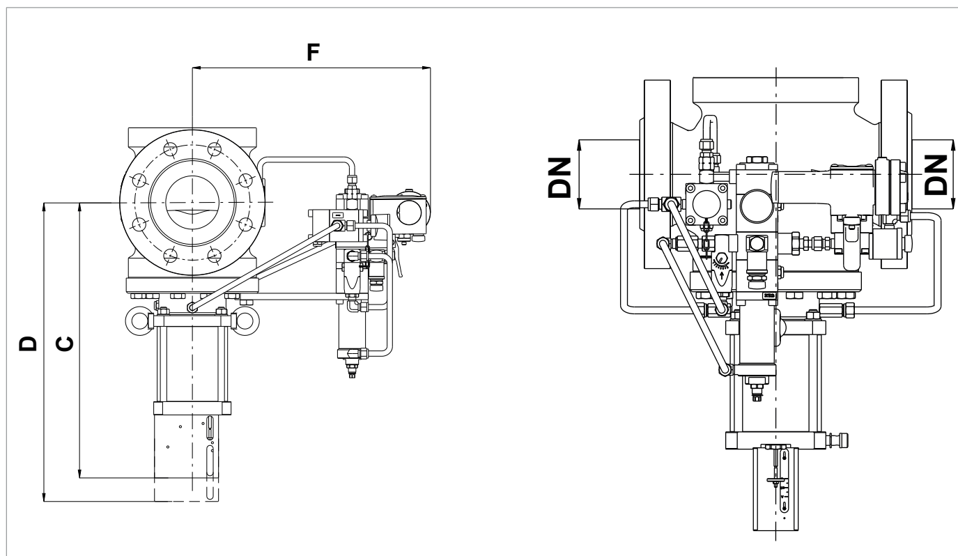
Fig. 5.18. Características físicas REFLUX 819/FO + HB/97
