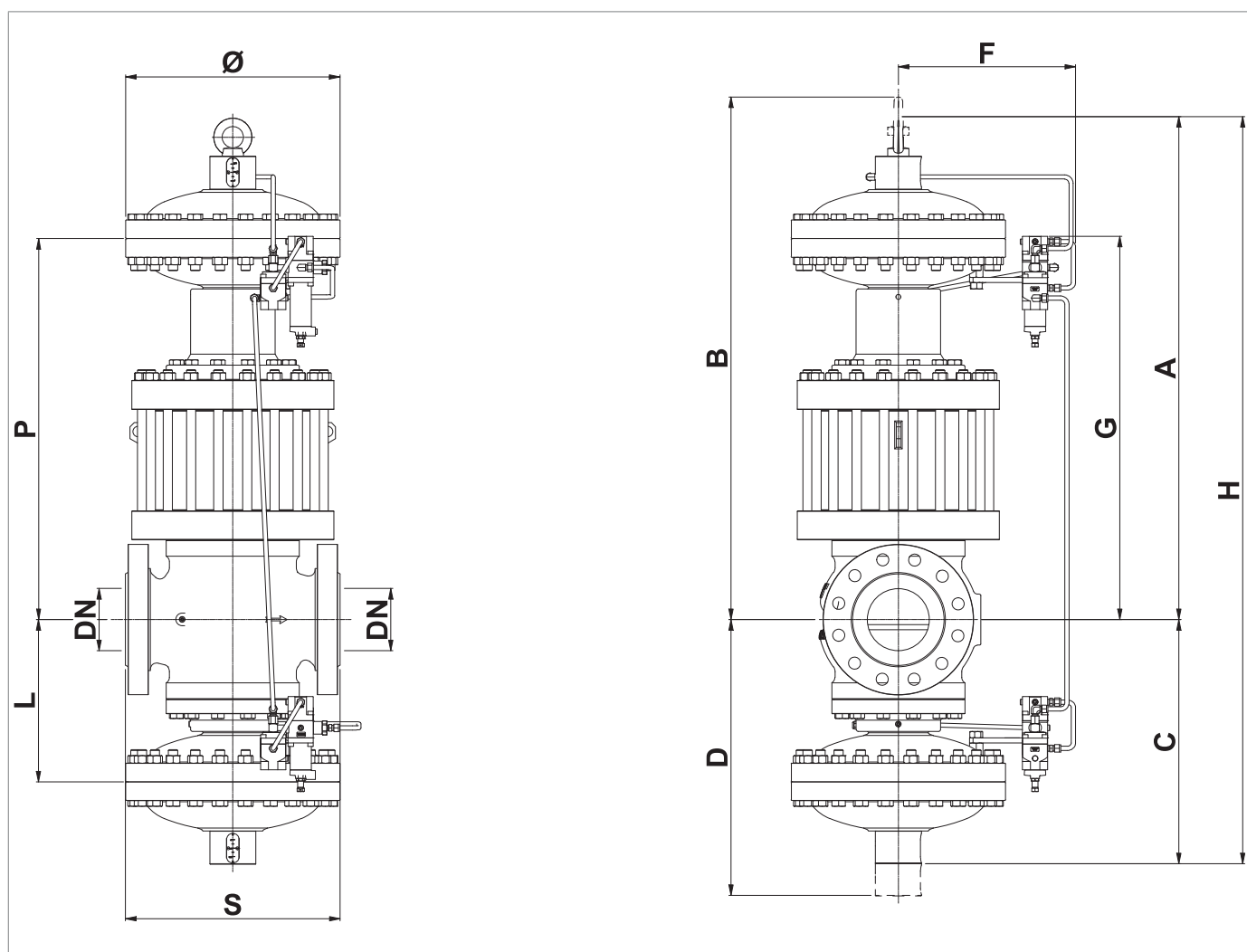
Fig. 5.19. Características físicas REFLUX 819/FO + DB/819 + PM/819
