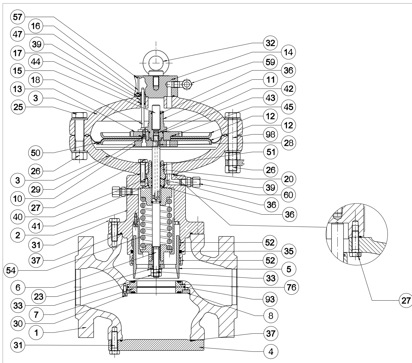
Fig. 9.56. Regulador REFLUX 819/FO 2" ÷ 3"
