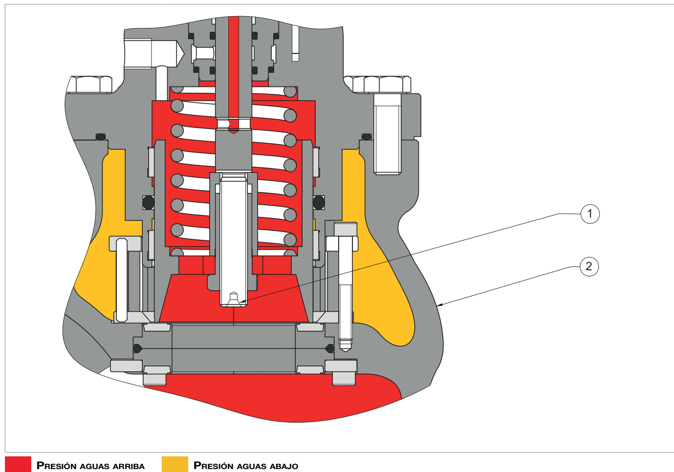
Fig. 4.4. Silenciador incorporado LDB/171
