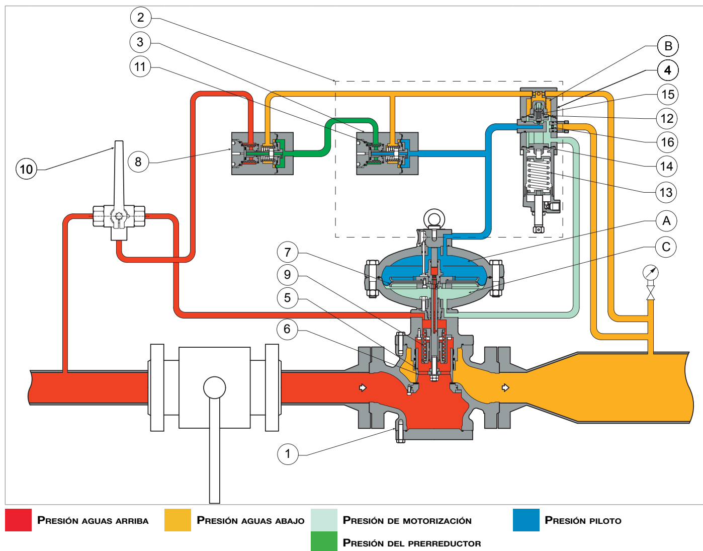
Fig. 4.2. Funcionamiento REFLUX 819/FO
