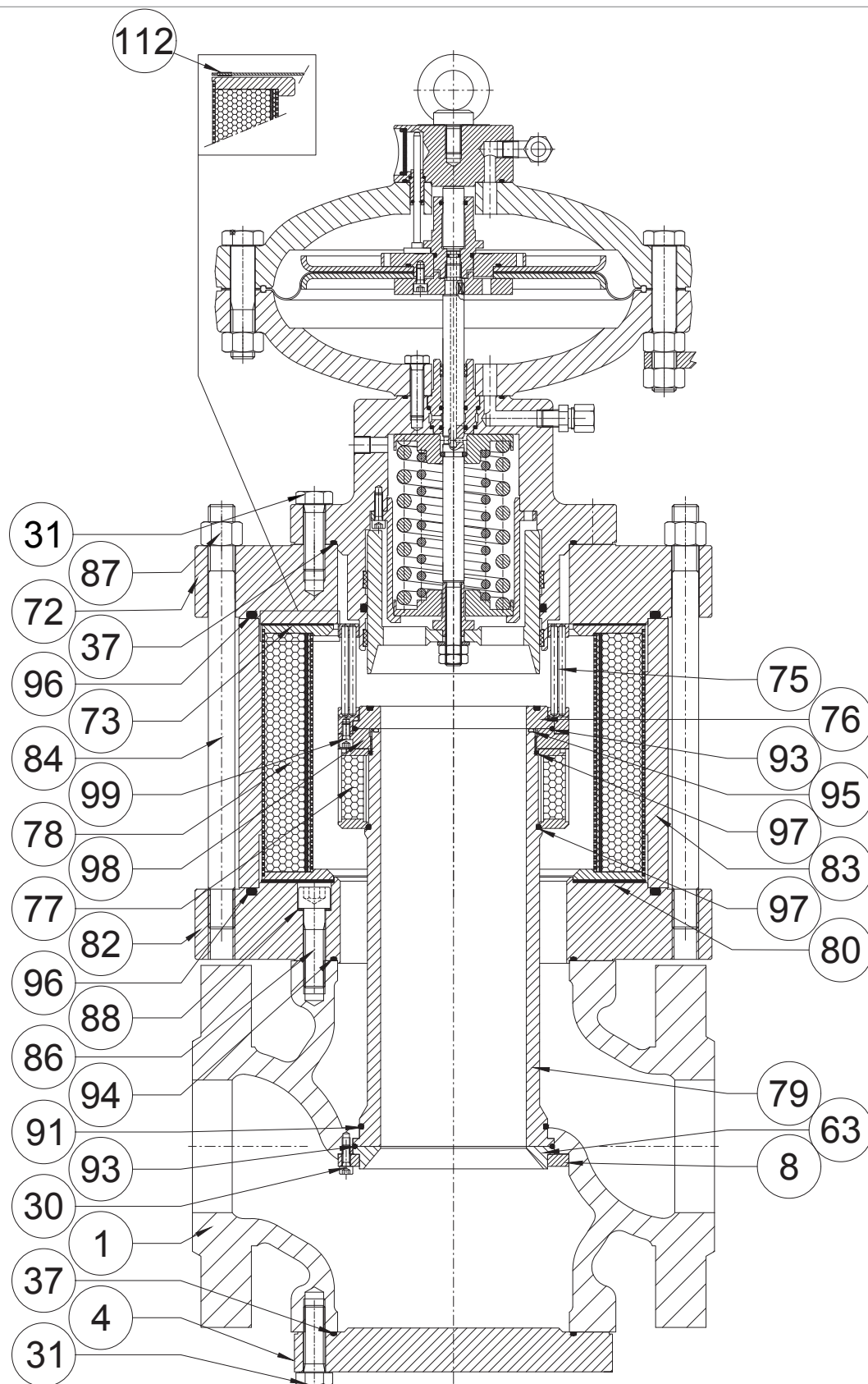
Silenciador DB/819
