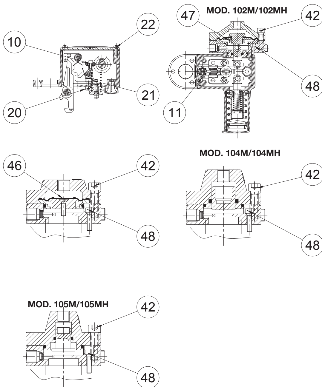
Fig. 9.49. Pares de apriete de los presostatos modelos 102M/102MH ÷ 105M/105MH
