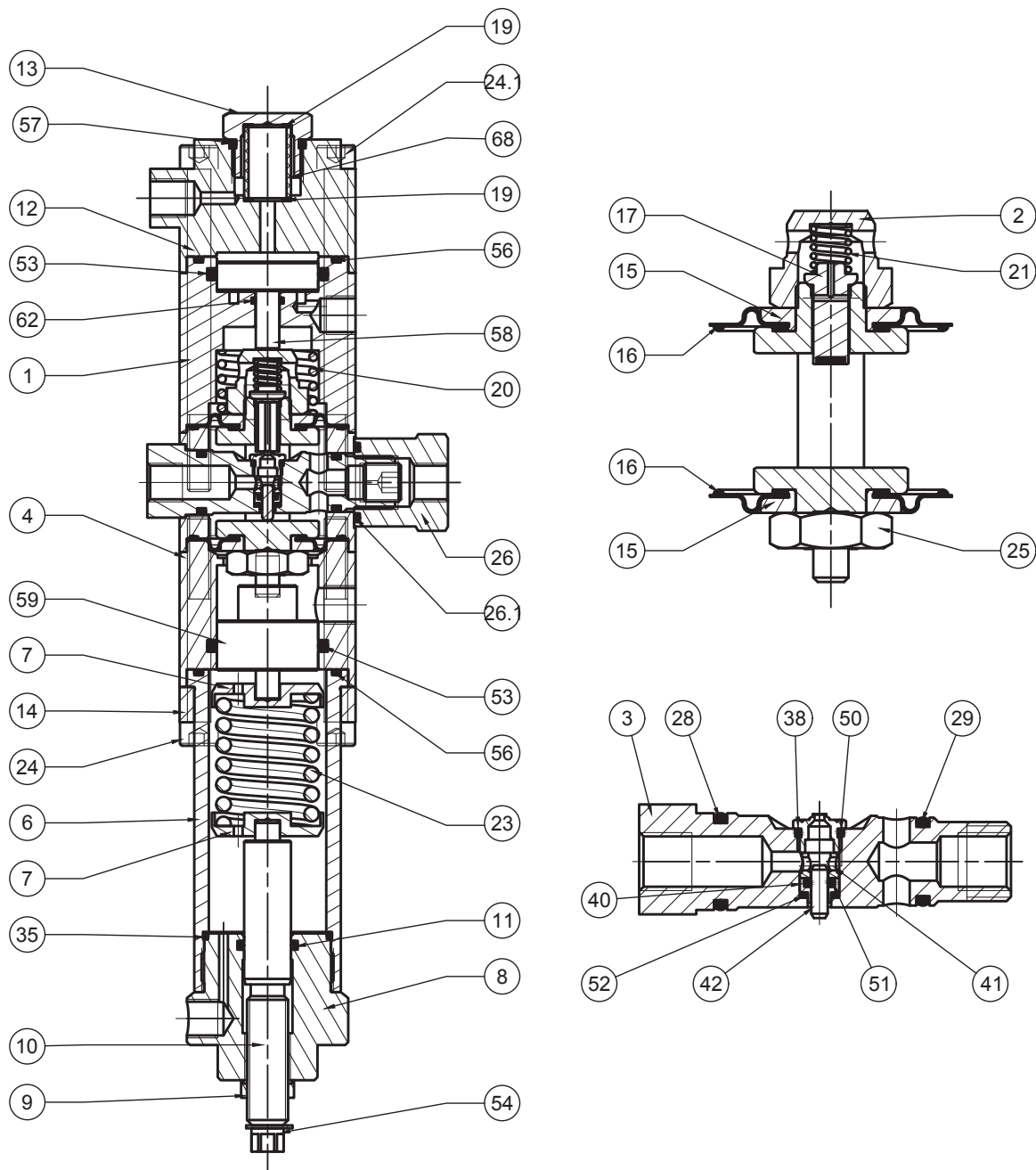
Fig. 9.82. Regulador de presión R44/SS
