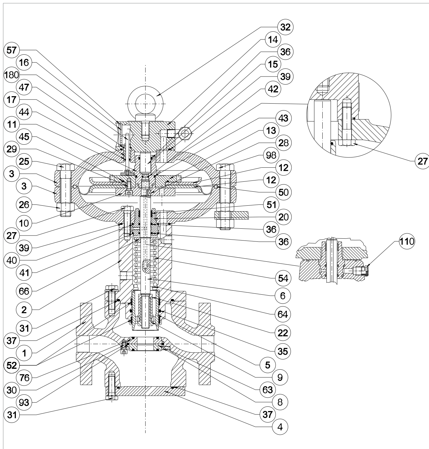
Fig. 9.55. Regulador REFLUX 819/FO 1"
