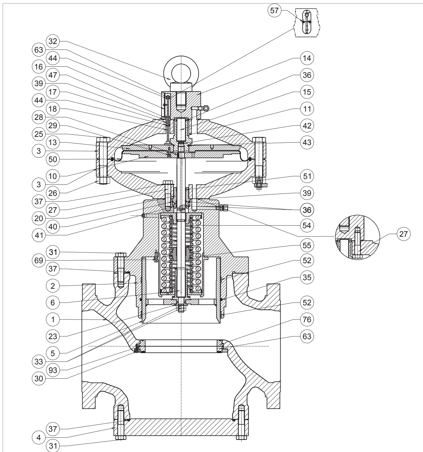
Fig. 9.58. Regulador REFLUX 819/FO 10"
