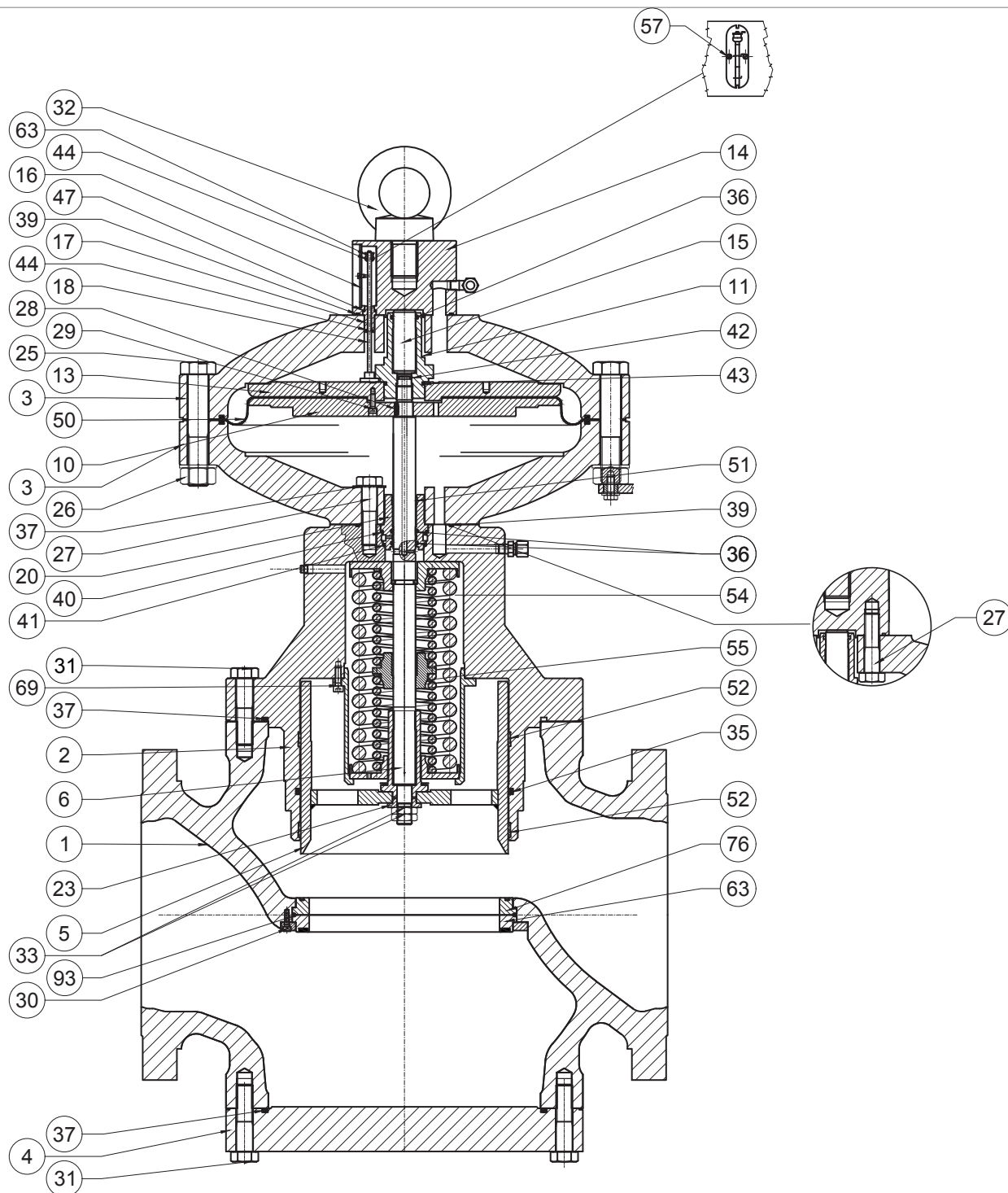
Regulador REFLUX 819/FO 10"
