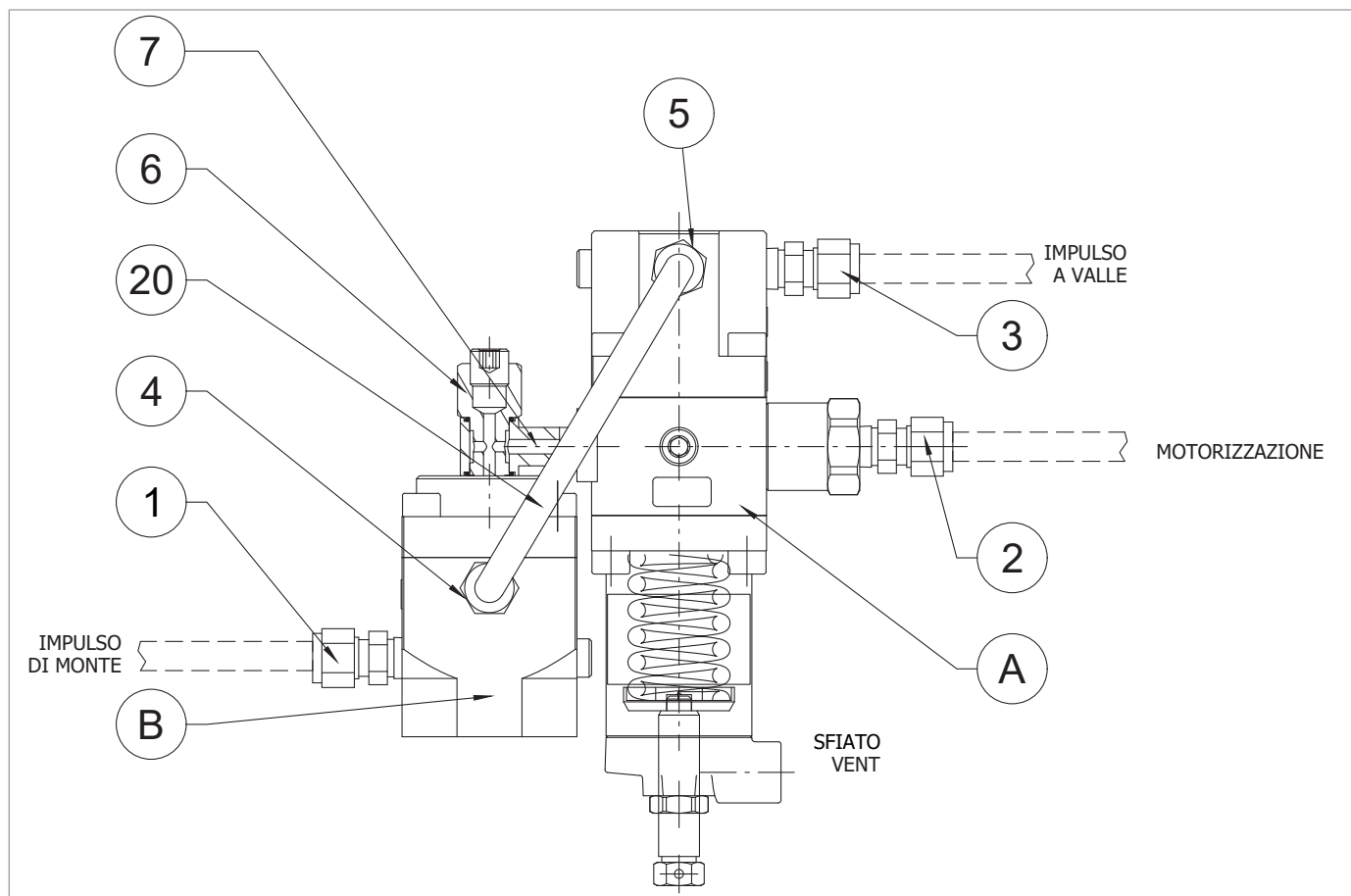
Fig. 9.64. Piloto serie 200/A y R14/A
