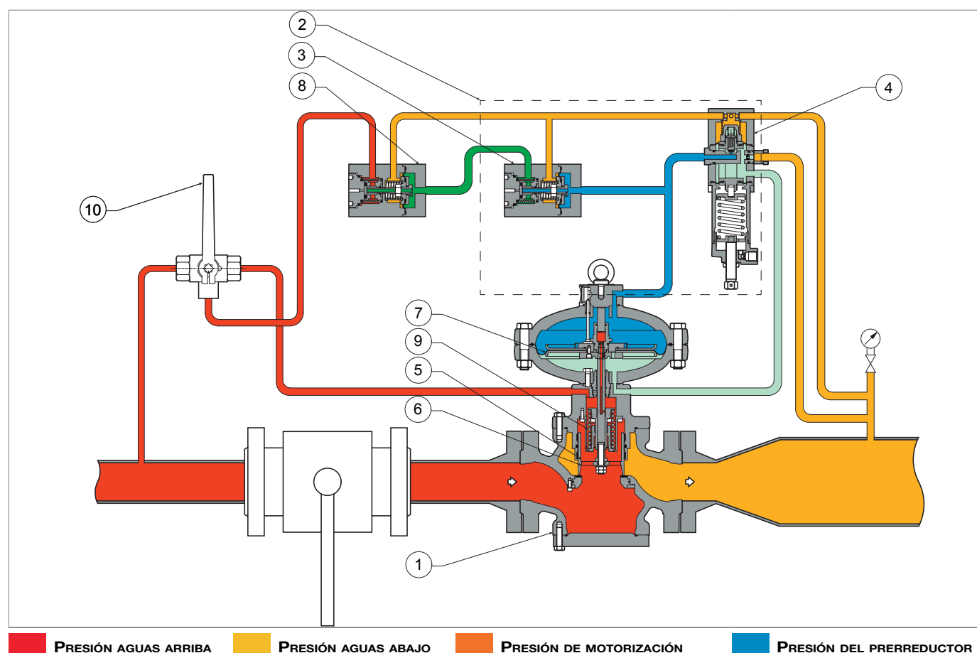
Fig. 4.1. Descripción general REFLUX 819/FO
