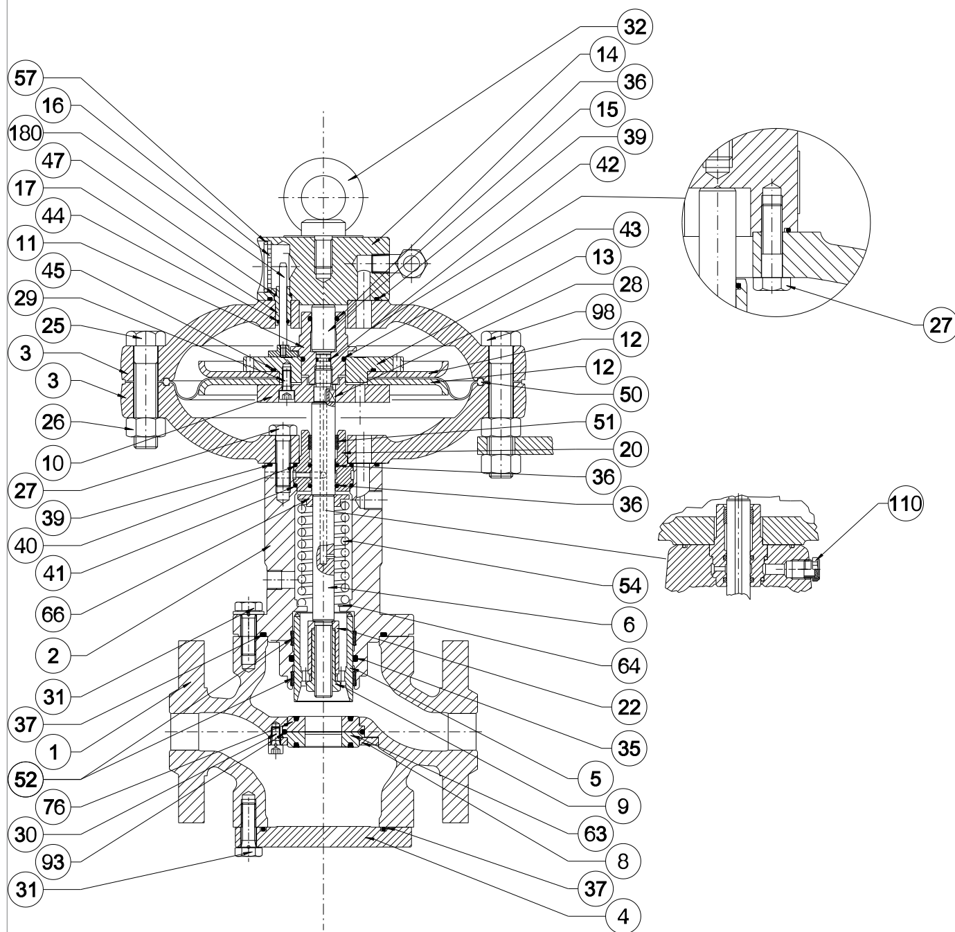
Regulador REFLEX 819/FO 1"
