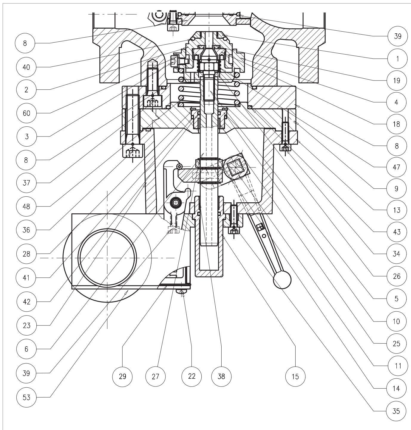
Fig. 9.71. Válvula de bloqueo incorporada SB/82 1"
