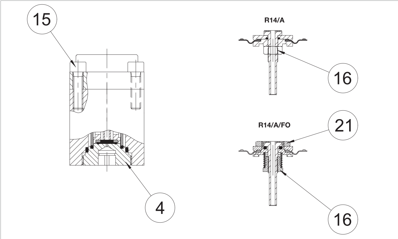
Fig. 9.43. Pares de apriete prerreductor R14/A/FO y R14/a
