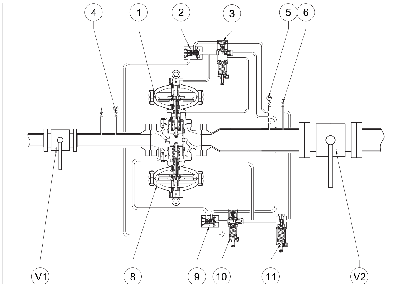
Fig. 8.31. Puesta en servicio del regulador PM/819 con monitor integrado y válvula aceleradora M/A
