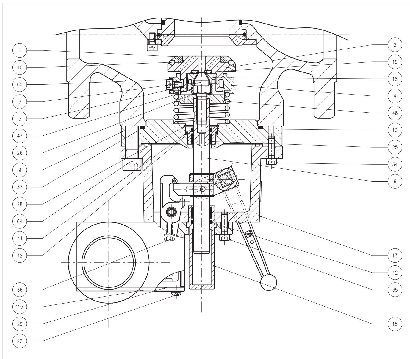
Fig. 9.72. Válvula de bloqueo incorporada SB/82 2"÷3"
