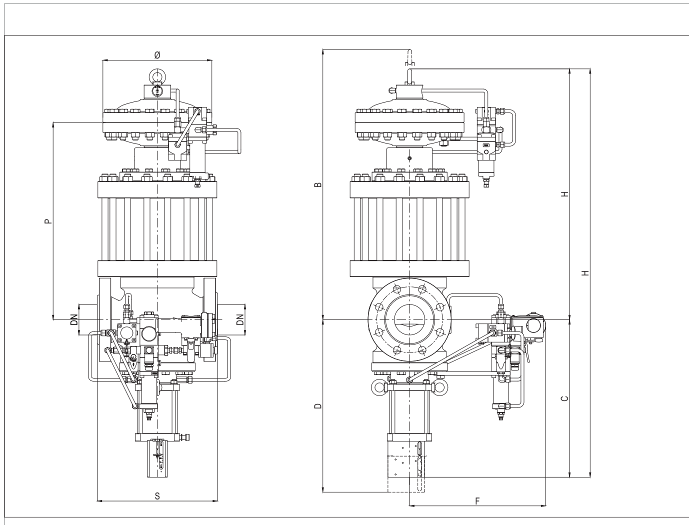
Fig. 5.21. Características físicas REFLUX 819/FO + DB/819 + HB/819
