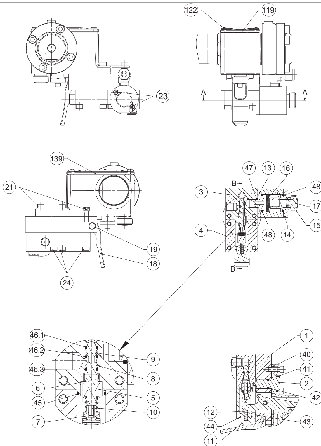
Válvula 3/2
