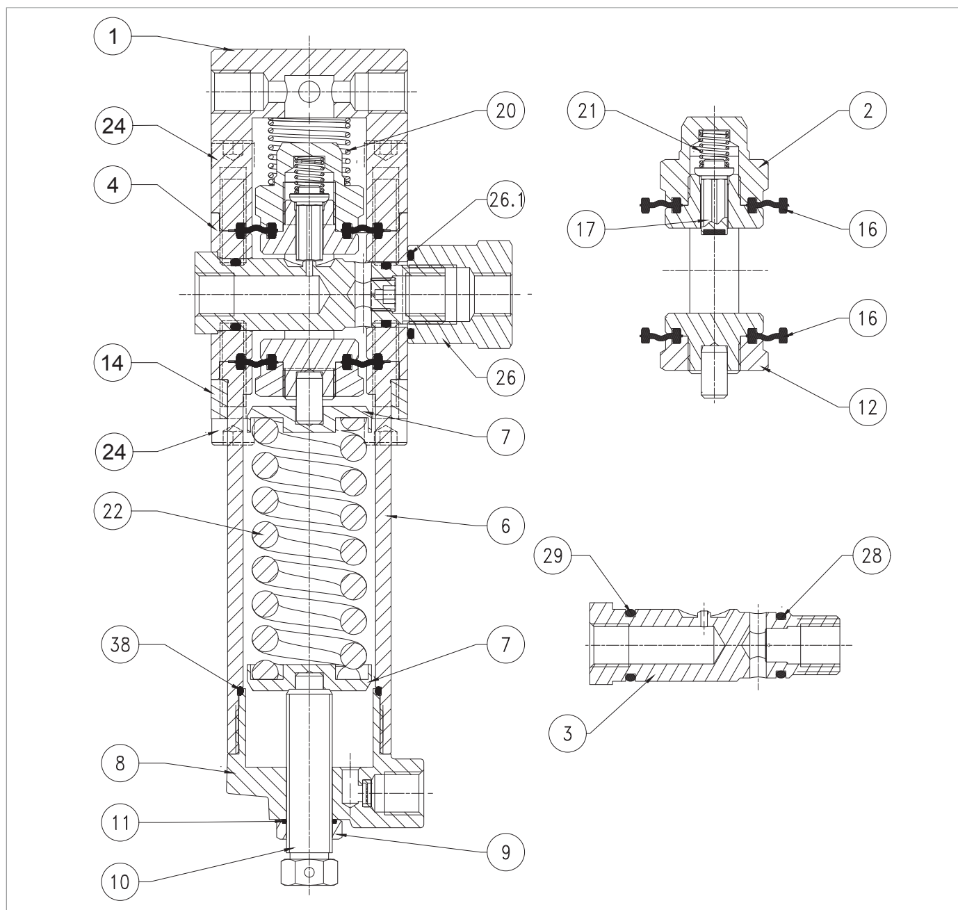
Fig. 9.66. PILOTO 207/A/ FO y 207/A
