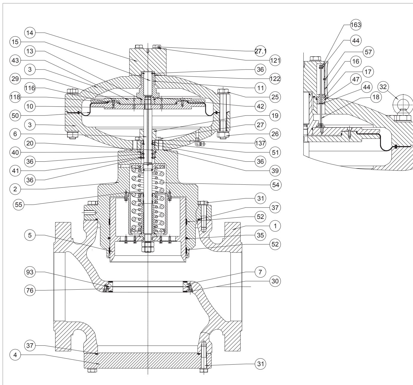
Fig. 9.59. Regulador REFLUX 819/FO 12"
