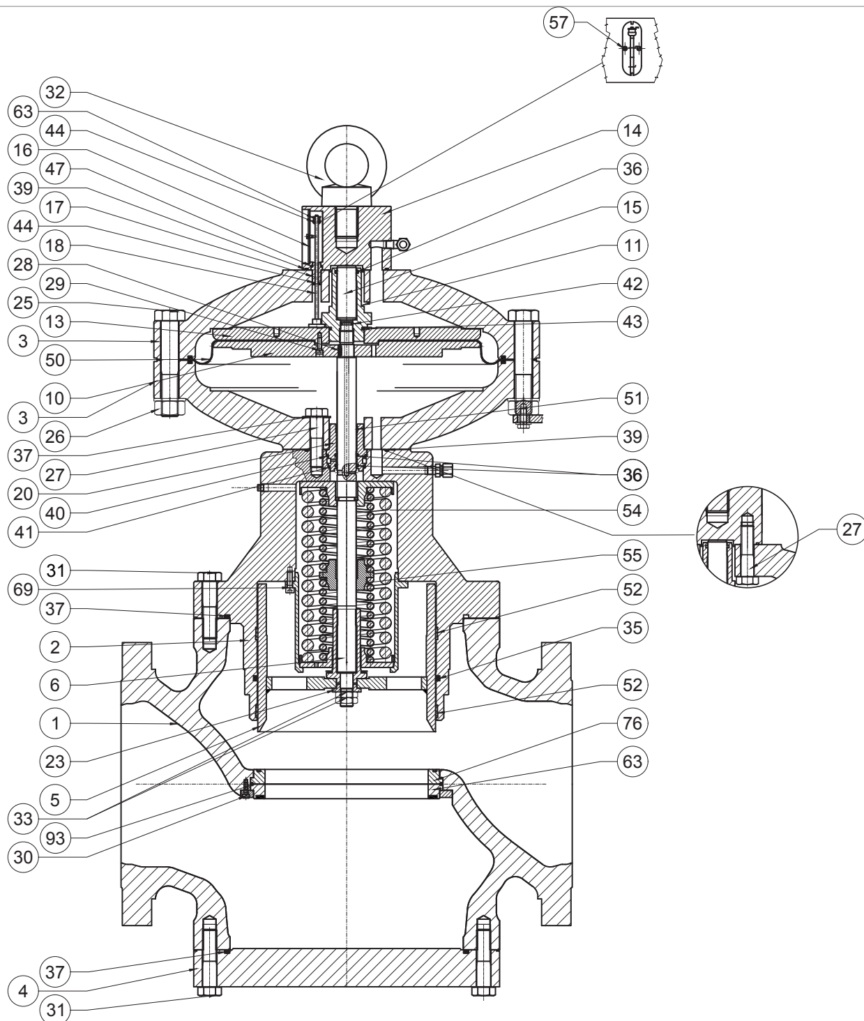
Regulador REFLEX 819/FO 10"
