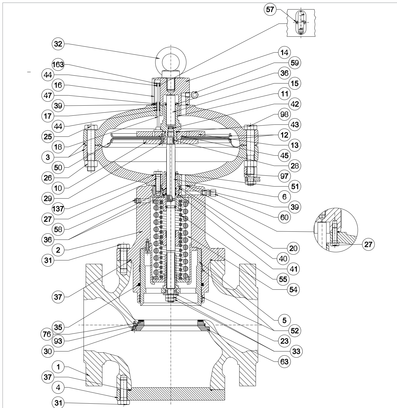
Regulador REFLEX 819/FO 4" ÷ 8"
