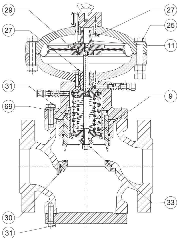
Pares de apriete REFLUX 819/FO
