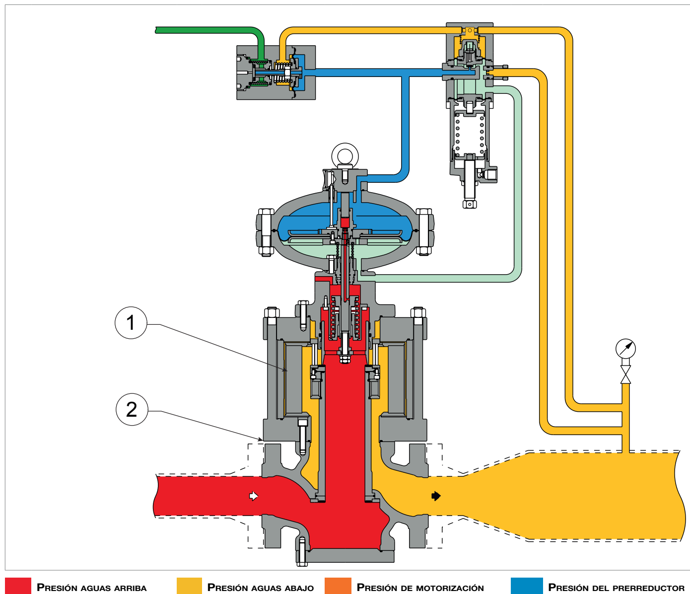
Fig. 4.3. Silenciador DB/819 integrado
