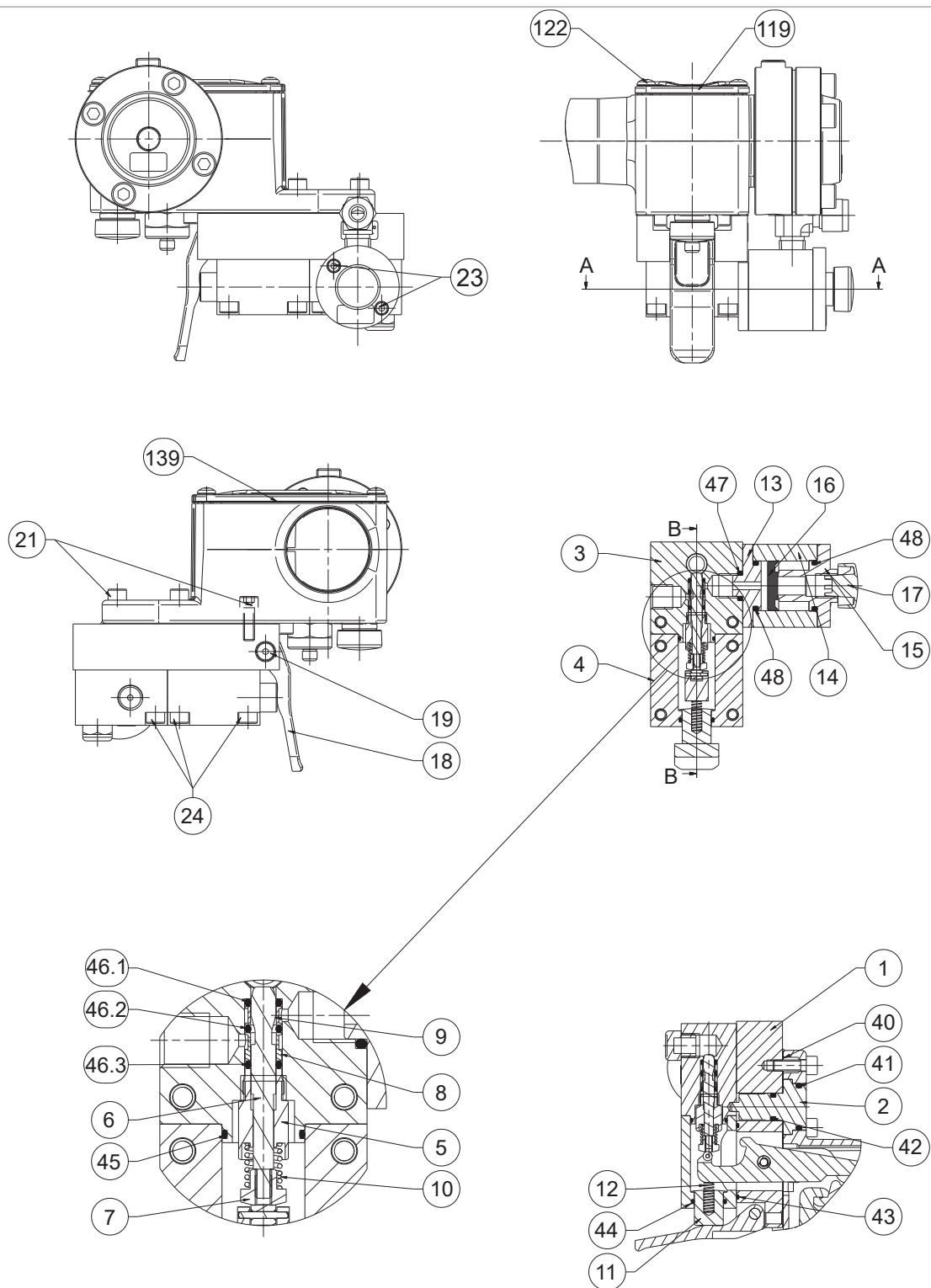
Fig. 9.84. Válvula 3/2
