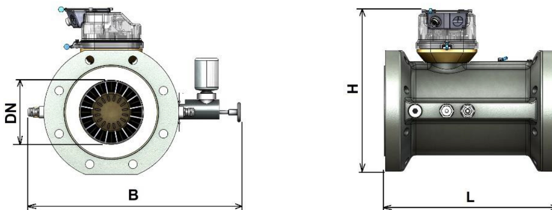
Figura 17 Dimensioni del corpo in alluminio iM-TM
