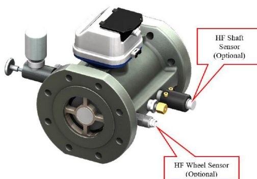
Figura 15 Sensori ad alta frequenza
