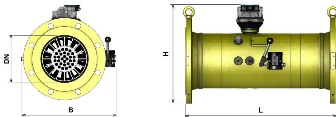
Figura 16 Dimensioni del corpo in acciaio iM-TM
