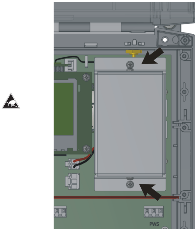
Figura 53 Viti contenitore batterie
