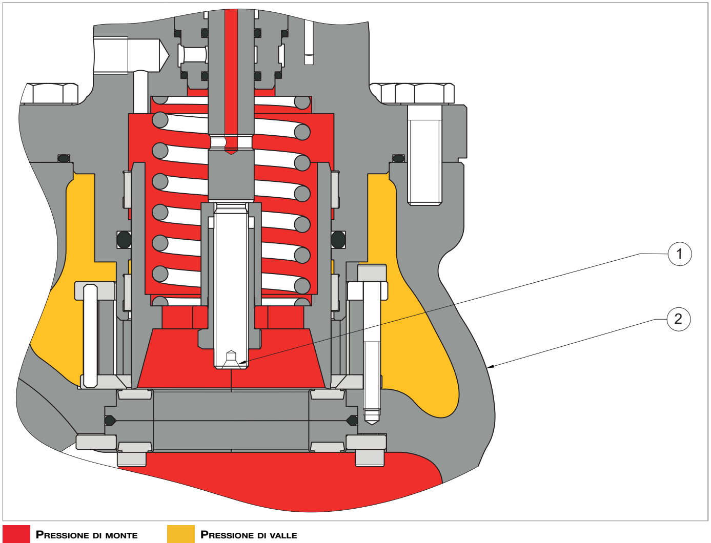
Fig. 4.4. Silenziatore incorporato LDB/171
