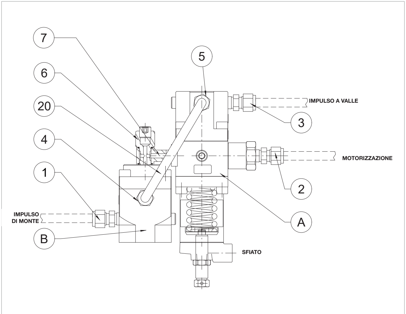
Fig. 9.64. Pilota 200/A
