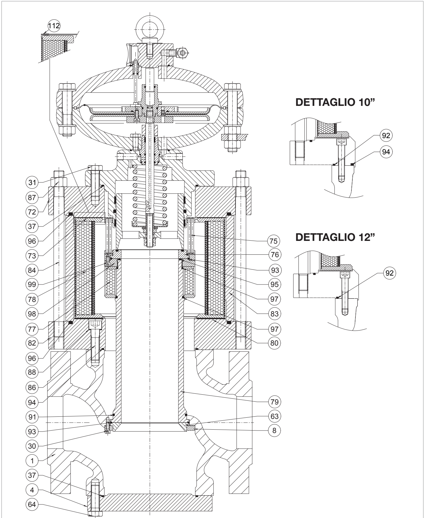
Fig. 9.60. Silenziatore DB/819
