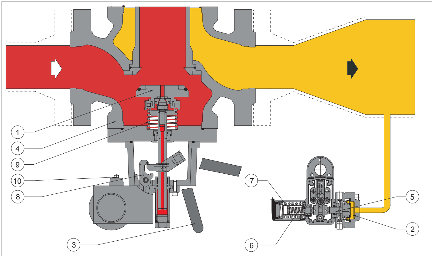
Fig. 4.10. REFLUX 819/FO con válvula de bloqueo incorporada SB/82
