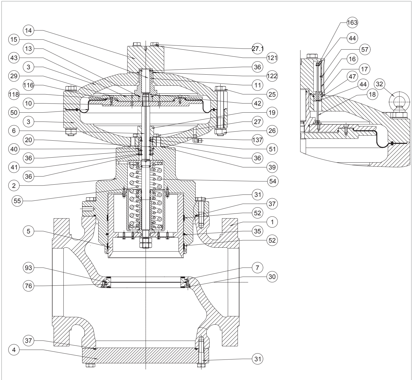
Regulador REFLUX 819/FO 12"
