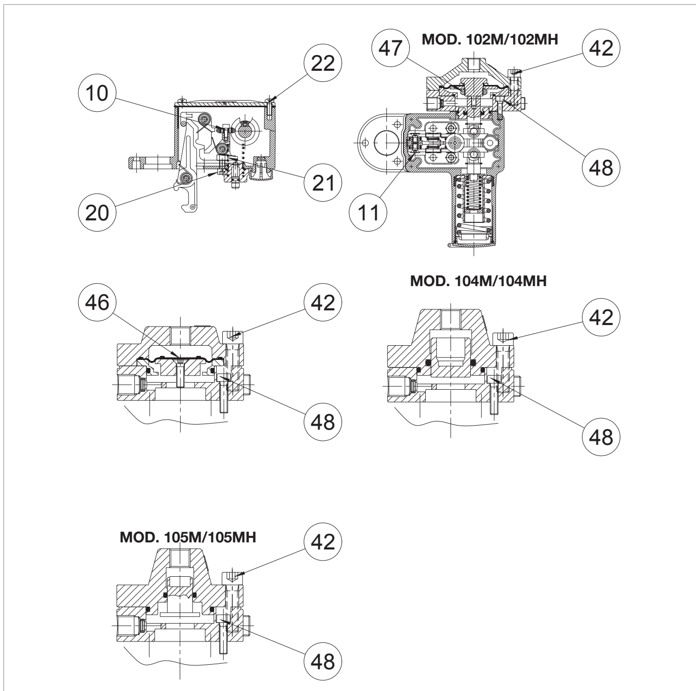
Fig. 9.49. Pares de apriete presostatos modelos 102M/102MH a 105M/105MH
