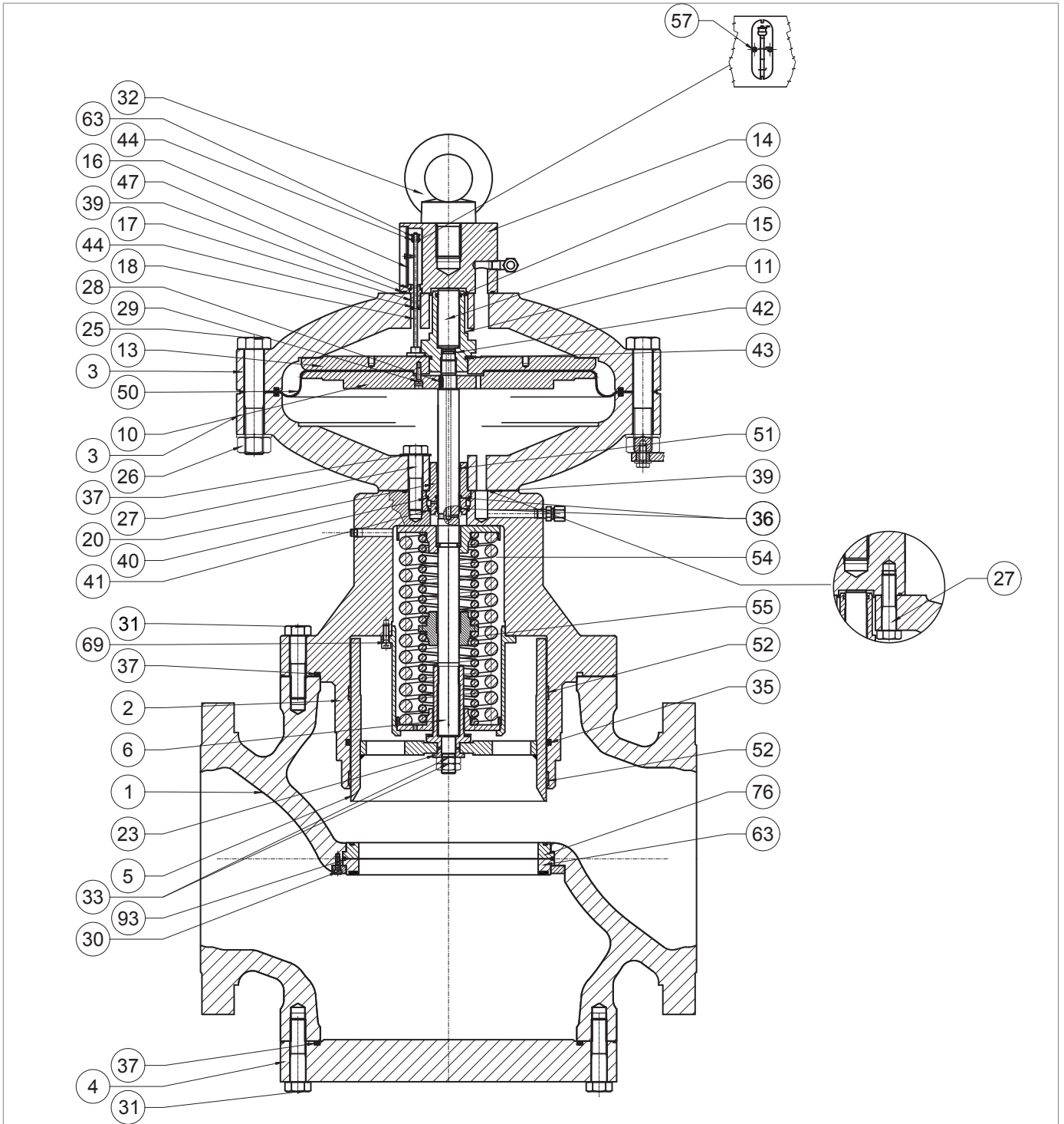
Regulador REFLUX 819/FO 10''
