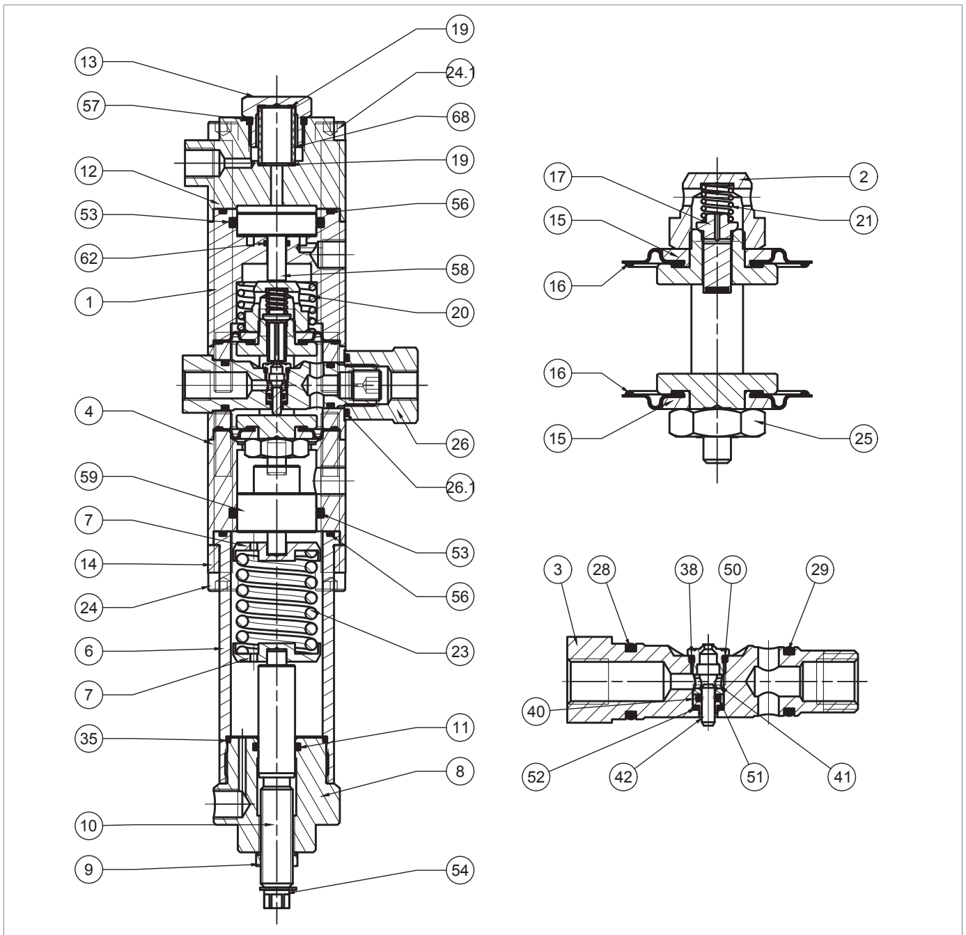
Fig. 9.82. Regulador de presión R44/SS
