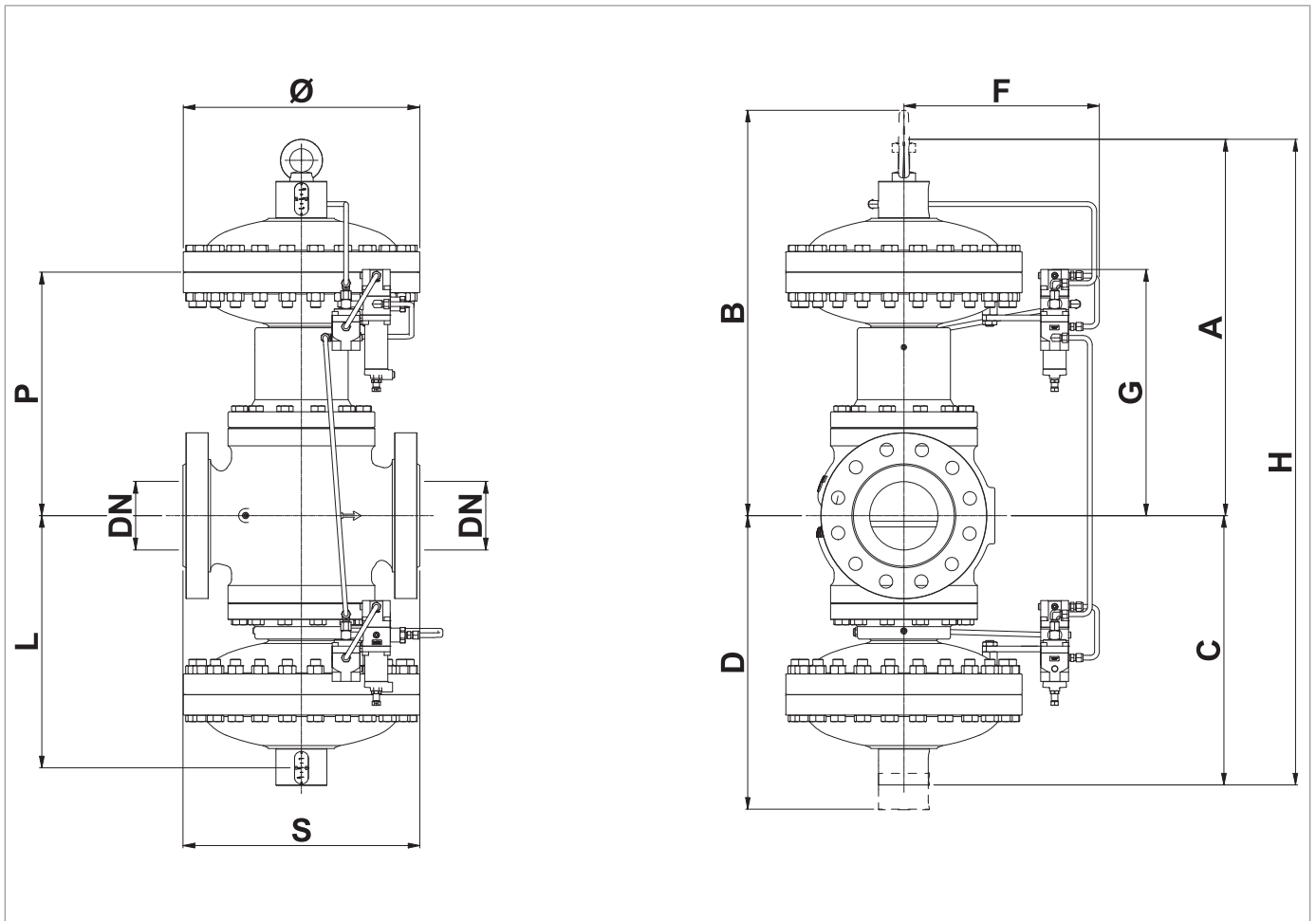
Fig. 5.16. Características físicas REFLUX 819/FO + PM/819
