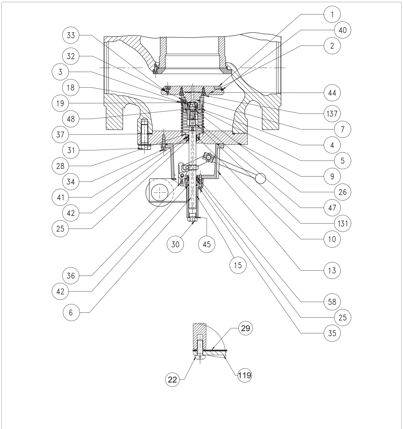
Fig. 9.73. Válvula de bloqueo incorporada SB/82 4" ÷ 8"
