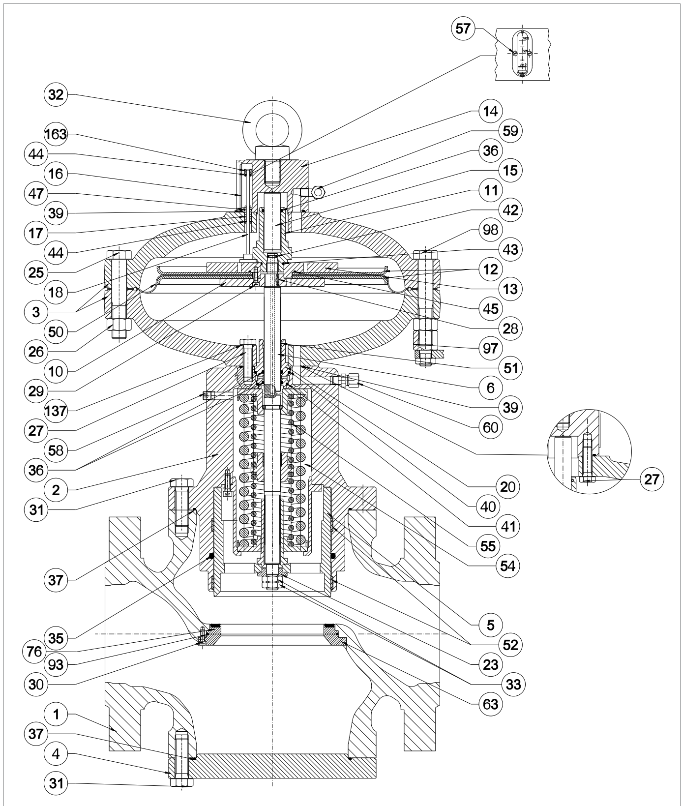
Fig. 9.57. Regulador REFLUX 819/FO 4" ÷ 8"
