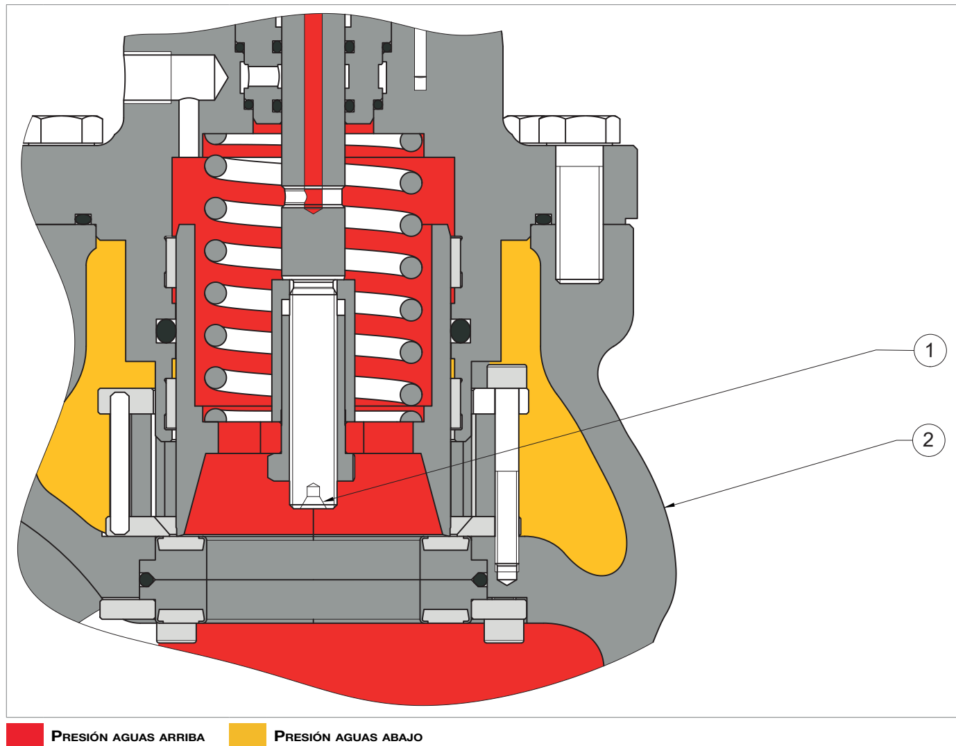
Fig. 4.4. Silenciador incorporado DB/171
