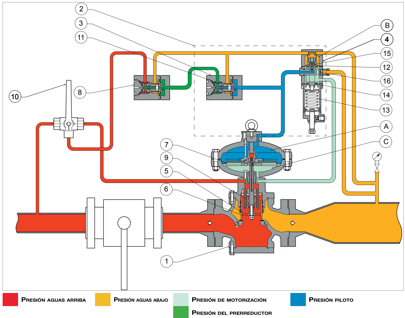
Fig. 4.2. Funcionamiento REFLUX 819/FO
