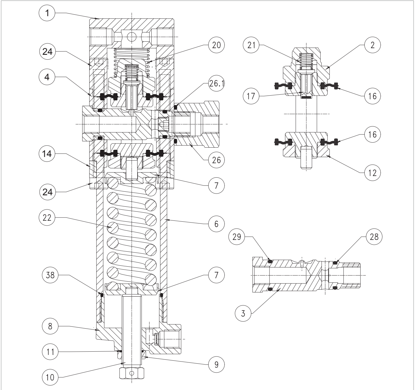
Piloto 207/A/FO y 207/A
