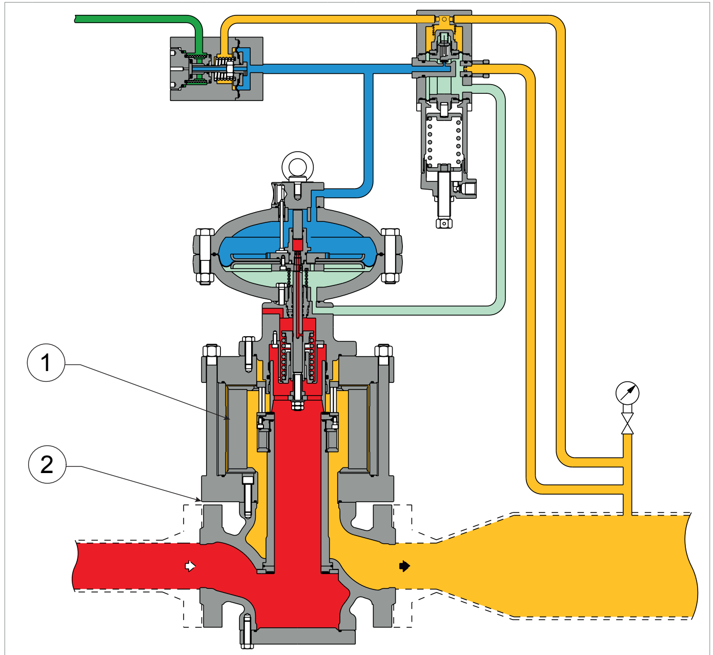
Fig. 4.3. Silenciador DB/819 integrado
