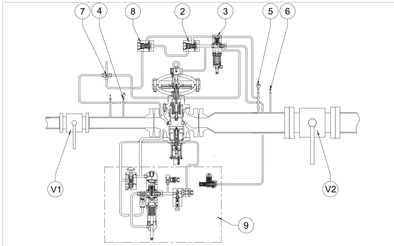
Fig. 8.35. Estanqueidad de la válvula de bloqueo incorporada SB/97
