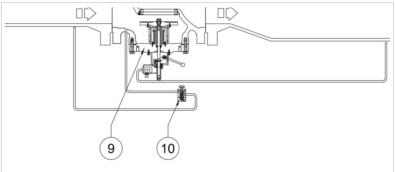
Fig. 8.33. Detalle by-pass HP2/2 para válvula de bloqueo incorporada SB/82 10"
