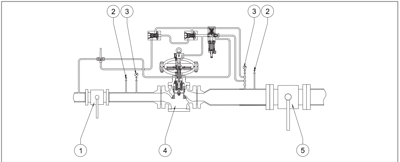
Fig. 6.22. Instalación en línea
