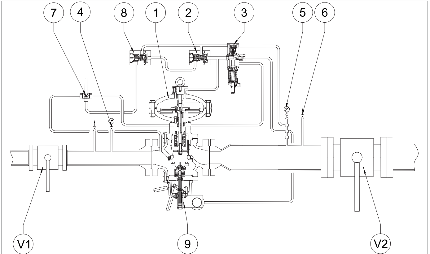
Fig. 8.32. Estanqueidad de la válvula de bloqueo incorporada SB/82
