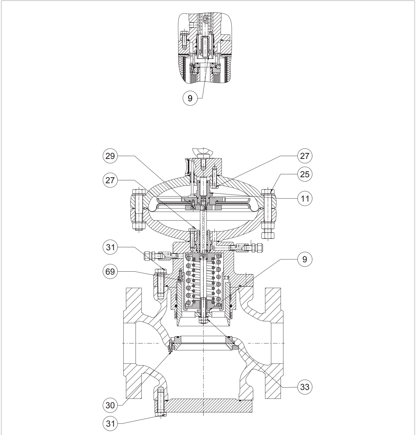
Pares de apriete REFLUX 819/FO
