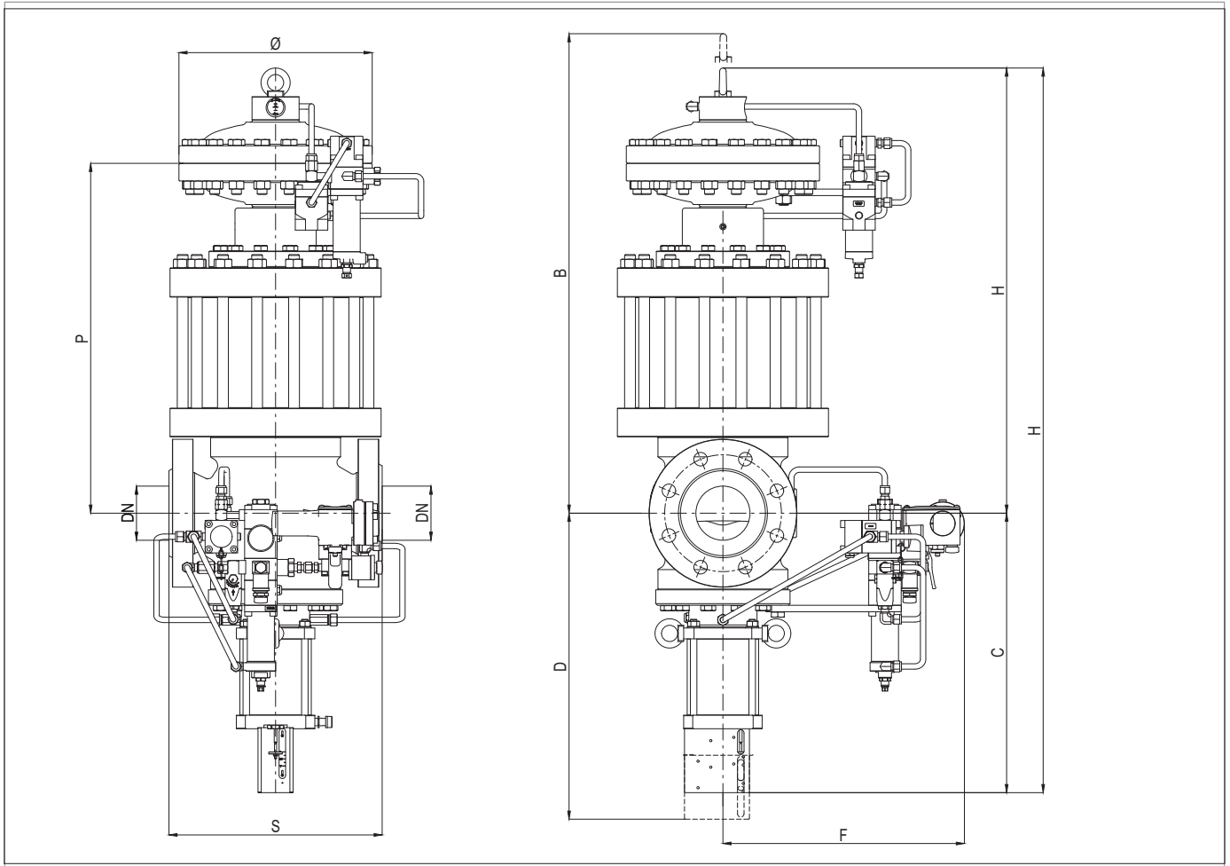
Fig. 5.21. Características físicas REFLUX 819/FO + DB/819 + HB/97
