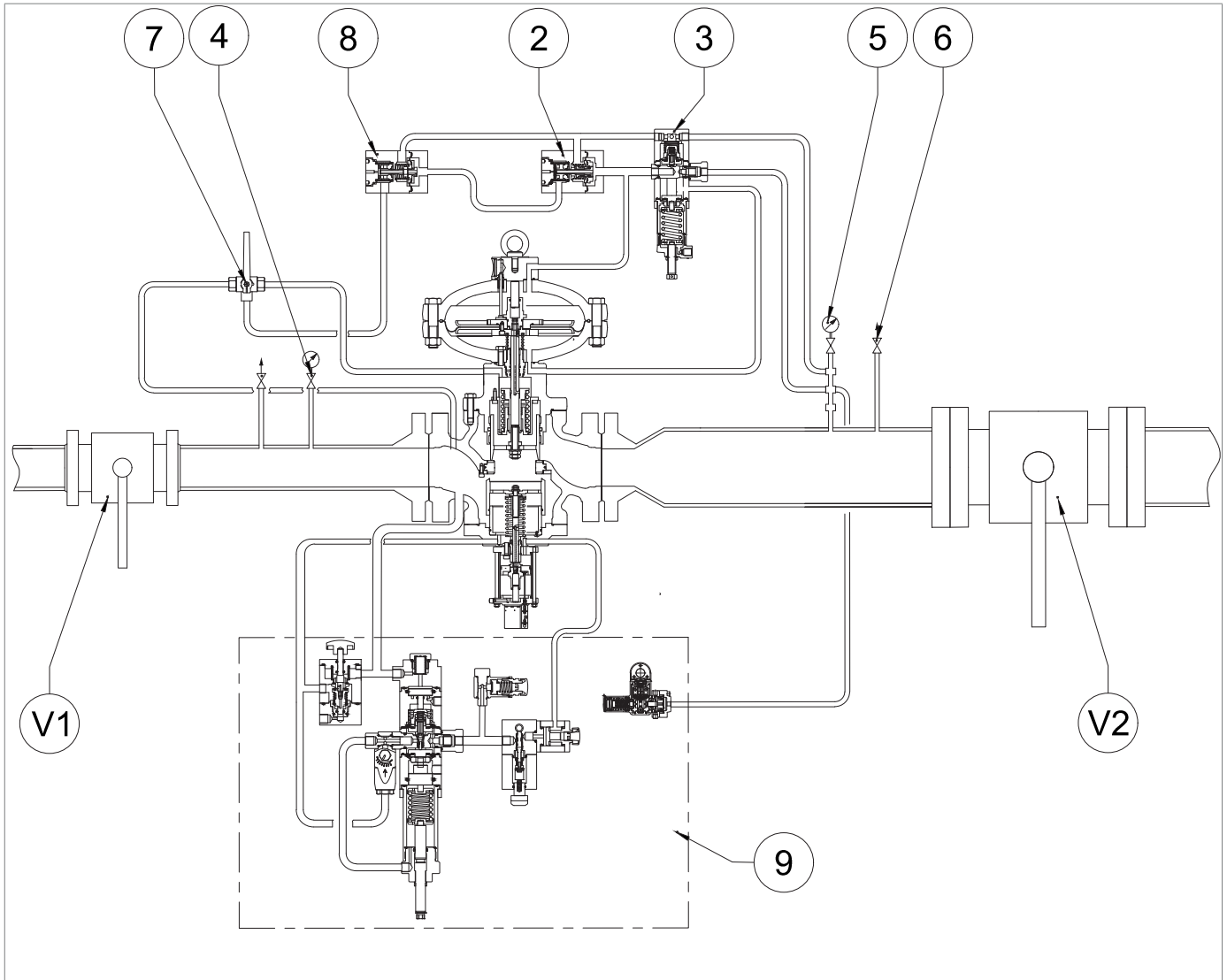
Fig. 8.35. Estanqueidad de la válvula de bloqueo incorporada SB/97
