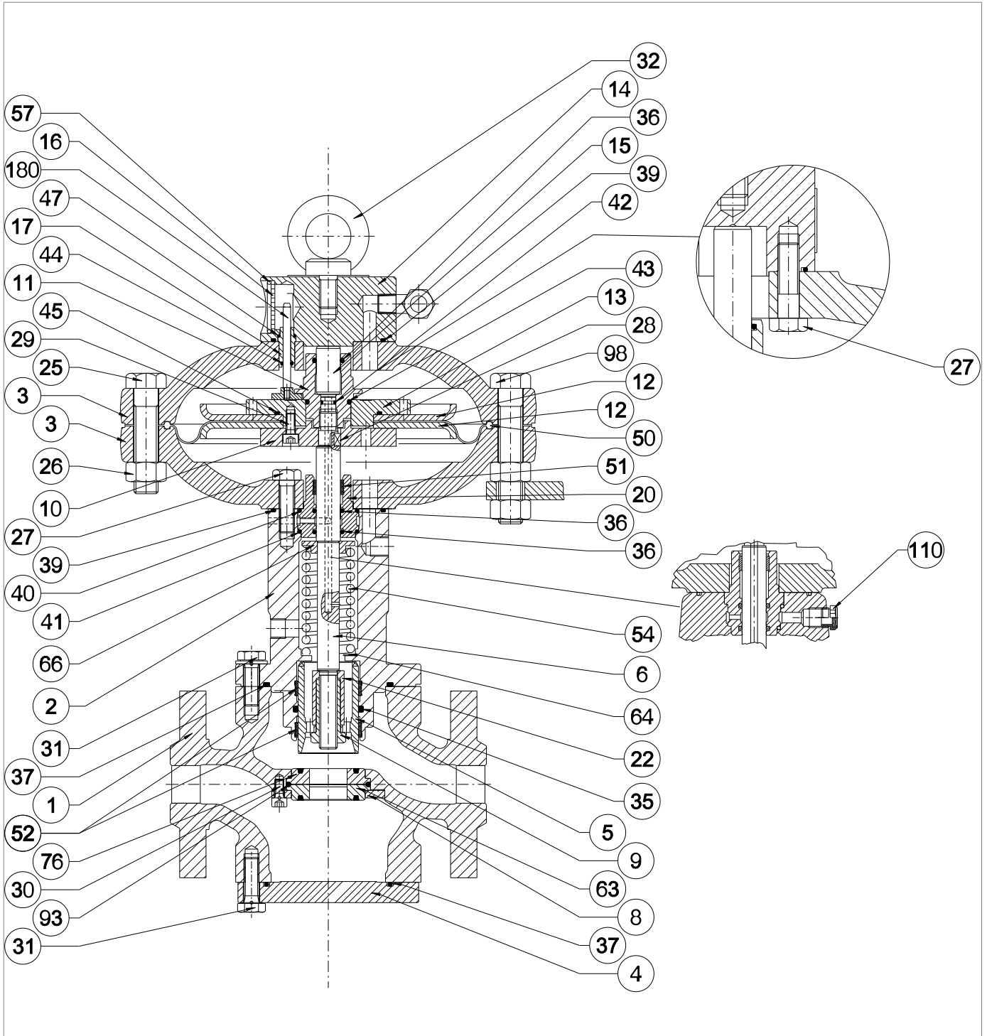
Regulador REFLUX 819/FO 1"
