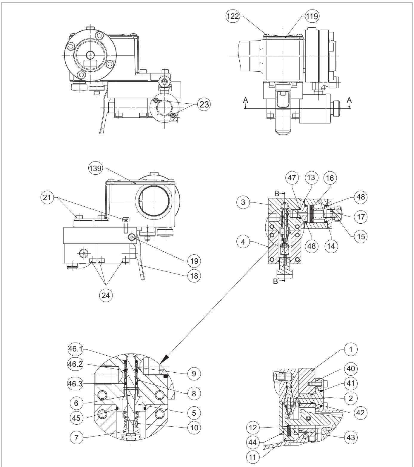
Fig. 9.84. Válvula 3/2
