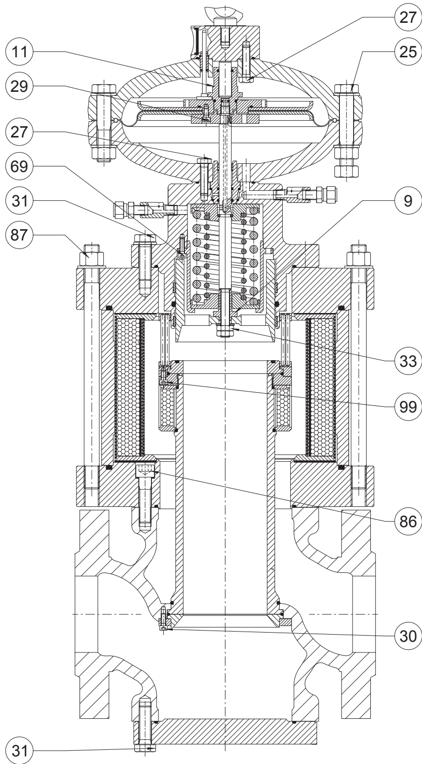
Pares de apriete REFLEX 819/FO + Silenciador DB/819
