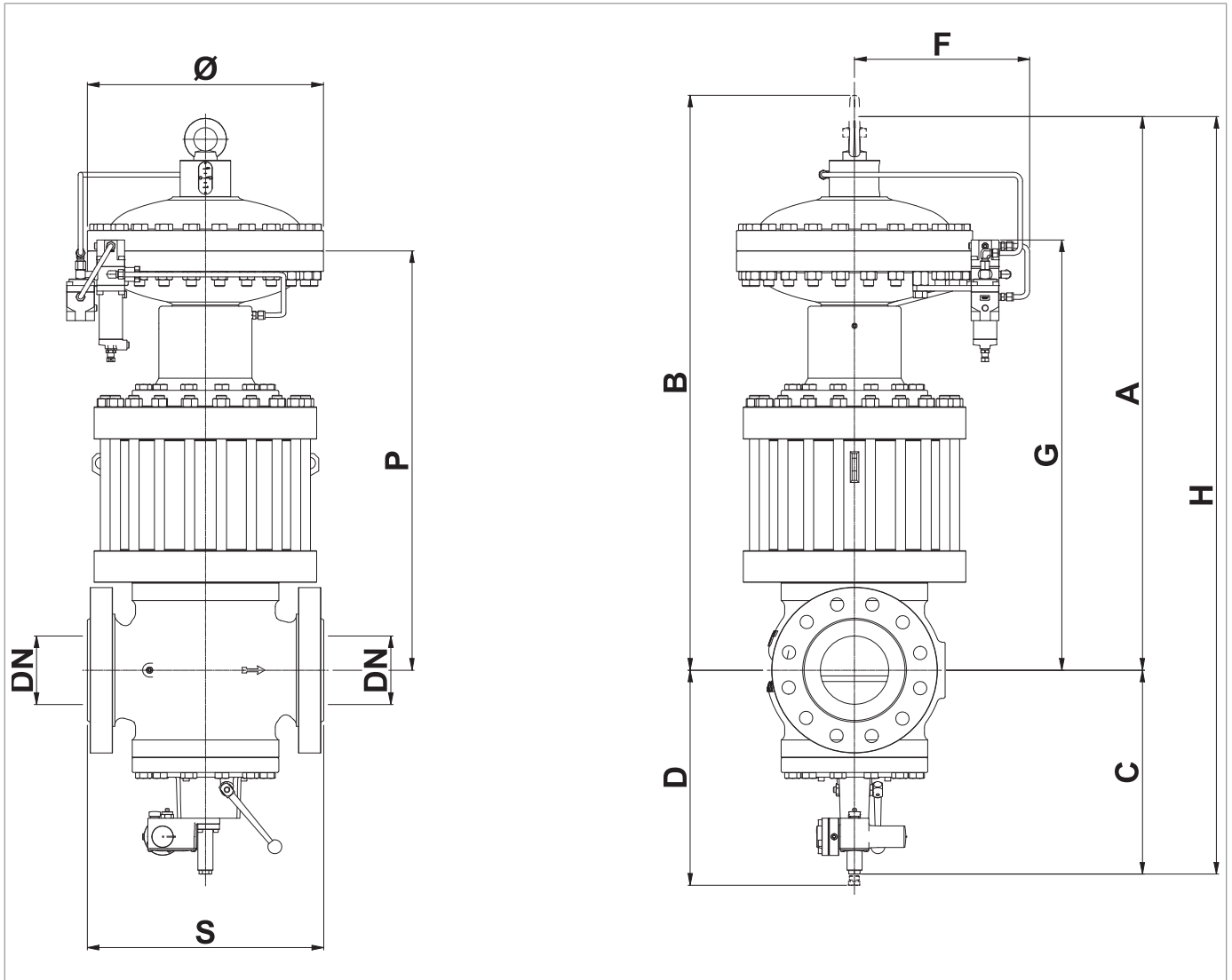
Fig. 5.20. Características físicas REFLUX 819/FO + DB/819 + SB/82
