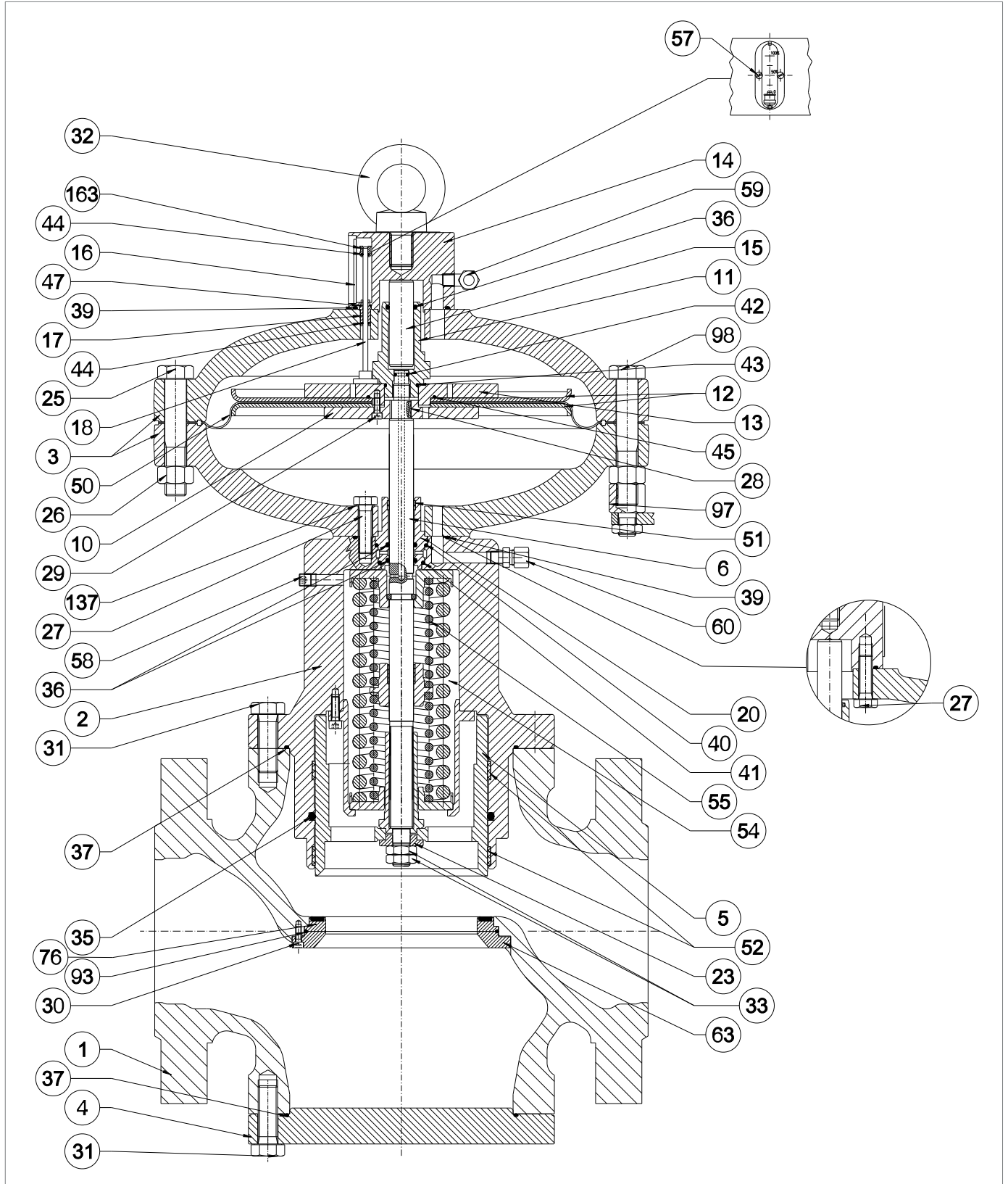
Regulador REFLUX 819/FO 4" ÷ 8"
