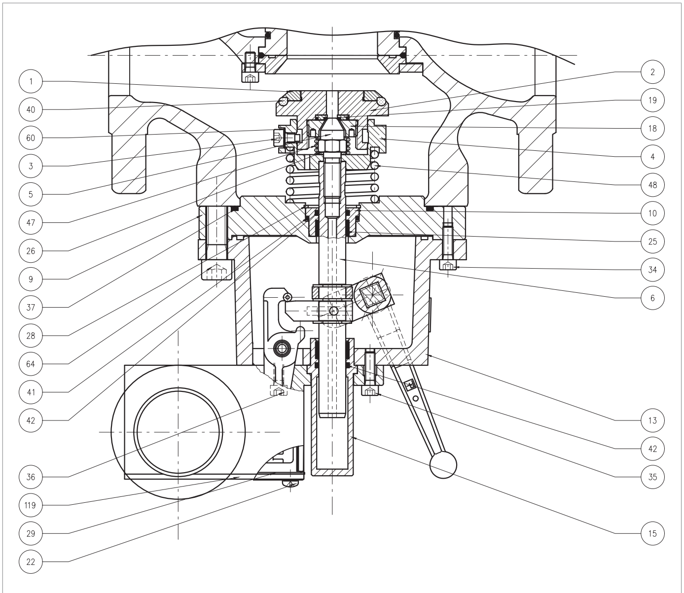
Fig. 9.72. Válvula de bloqueo incorporada SB/82 2" ÷ 3"
