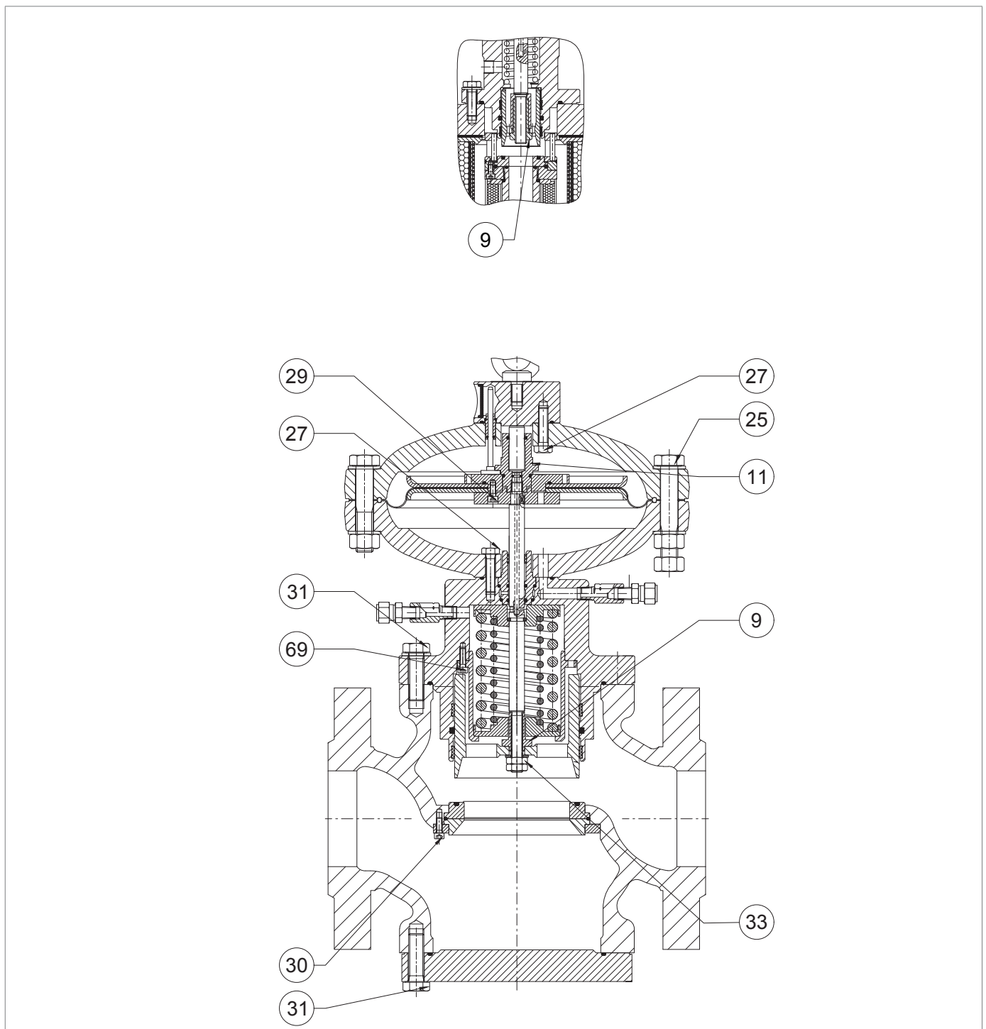
Fig. 9.39. Pares de apriete REFLUX 819/FO
