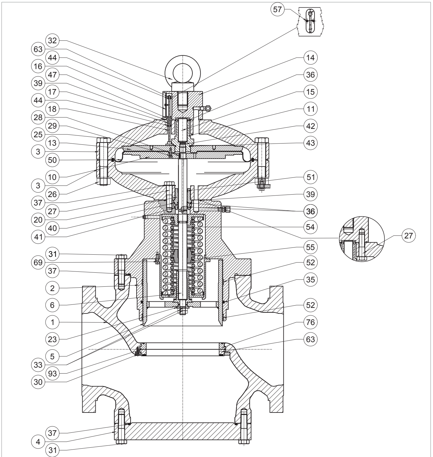
Fig. 9.58. Regulador REFLUX 819/FO 10"
