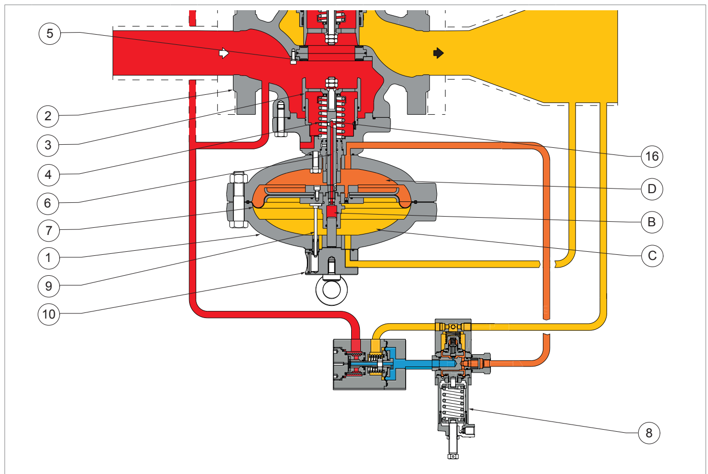
Fig. 4.6. Funcionamiento del monitor integrado
