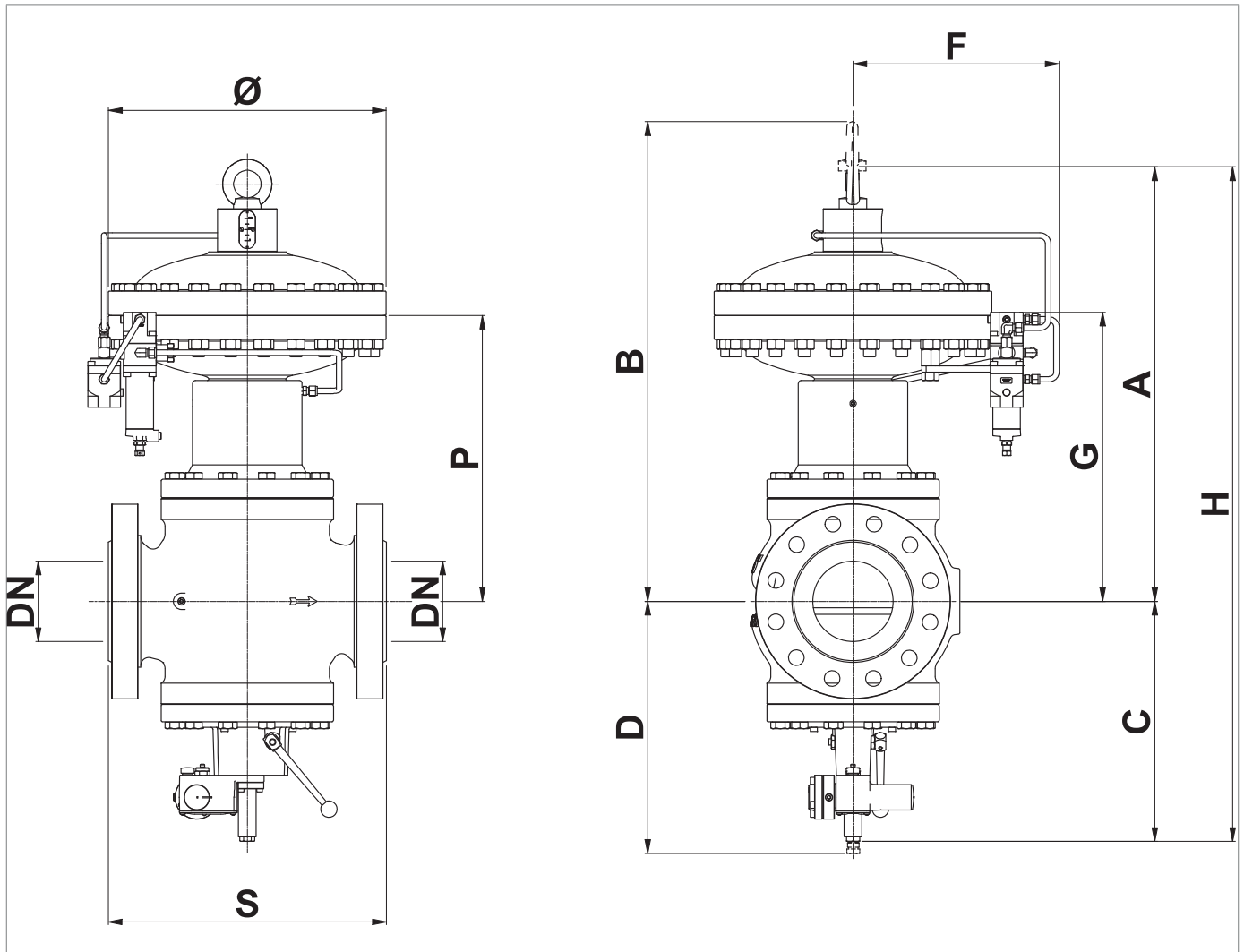
Fig. 5.17. Características físicas REFLUX 819/FO + SB/82
