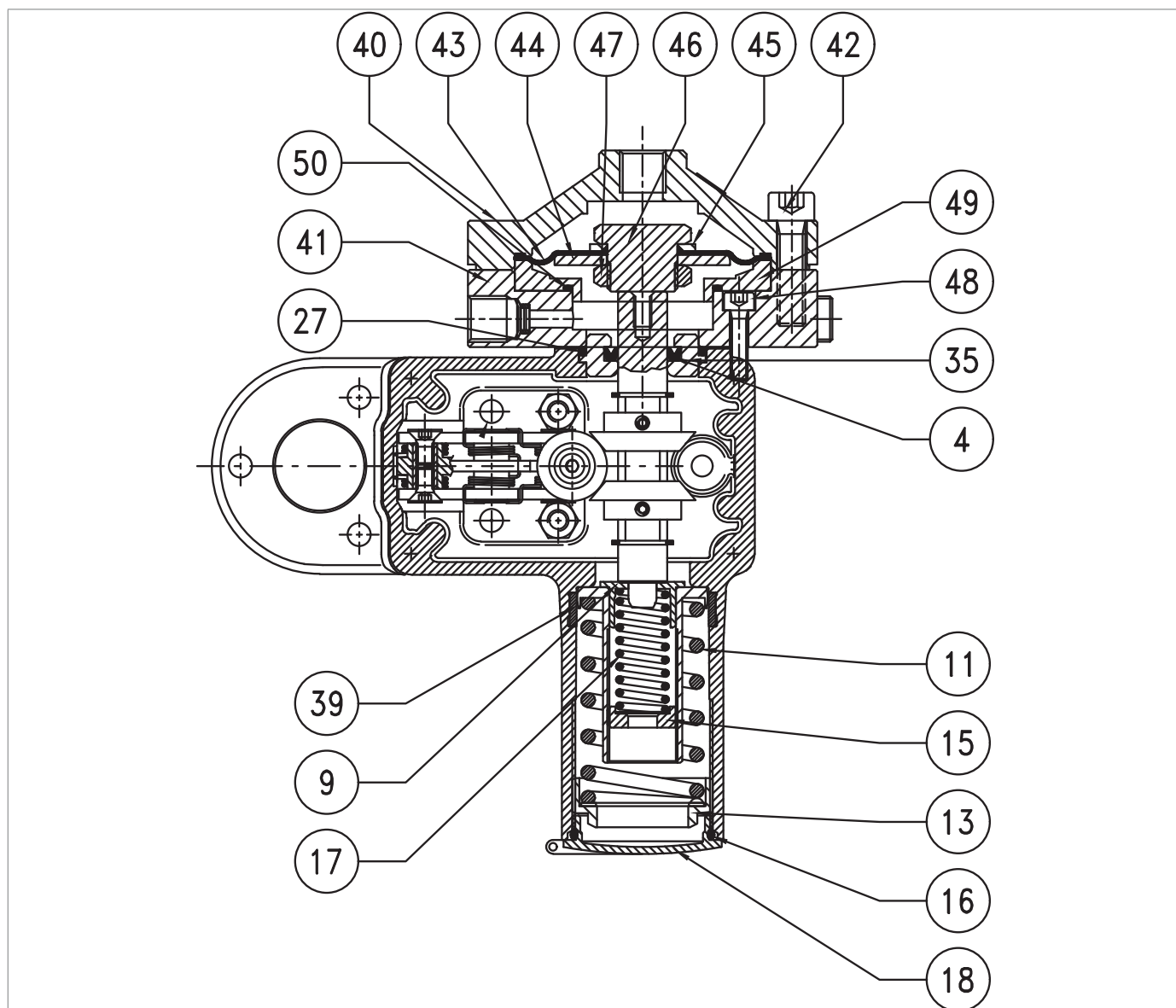
Fig. 9.27. Pressostat Mod. 102M/102MH
