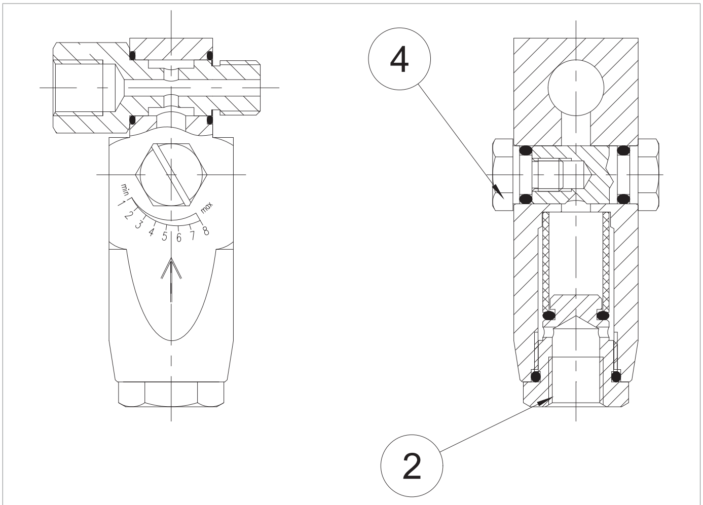
Fig. 9.18. Couples de serrage de la vanne de laminage AR100
