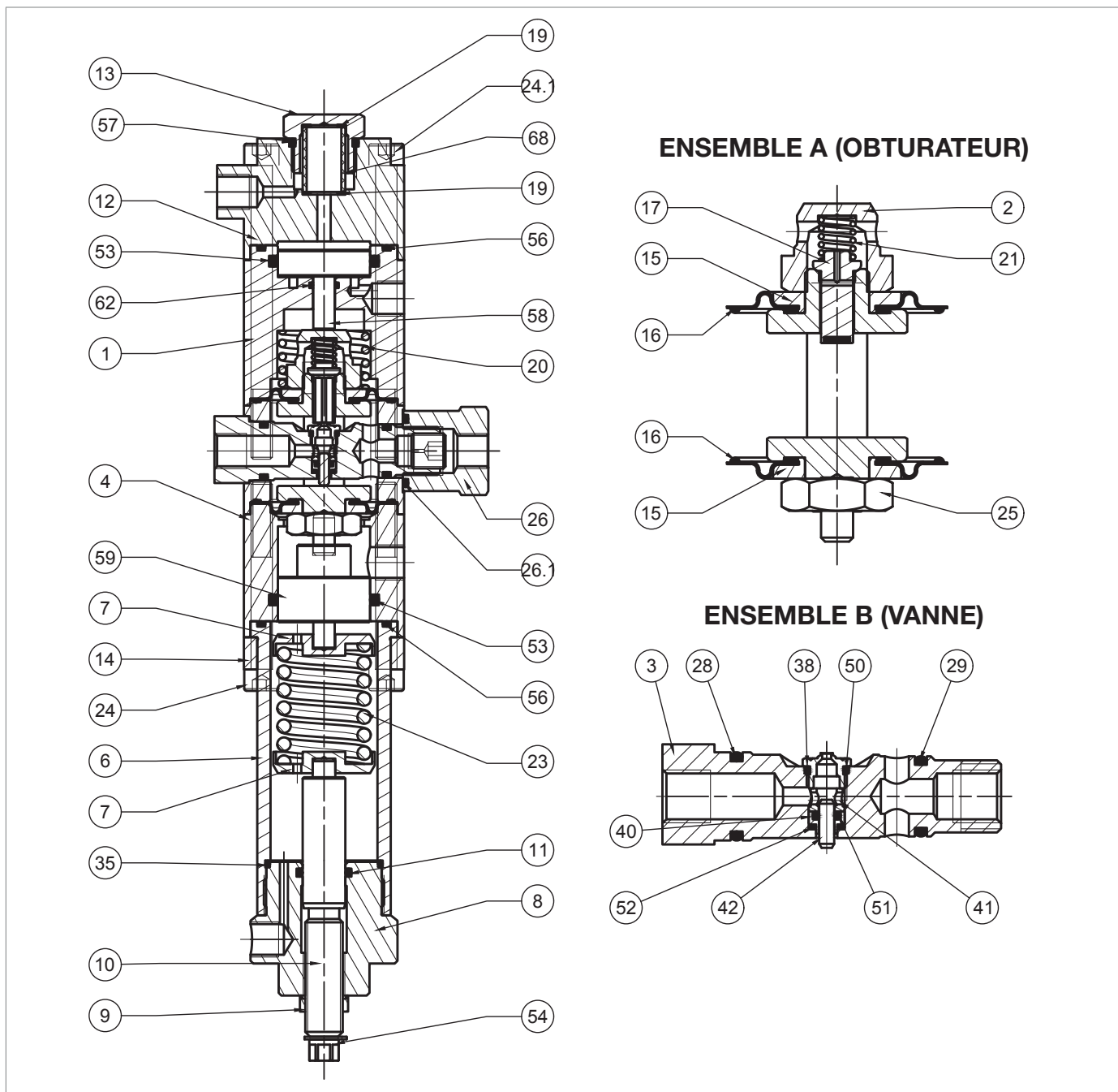
Fig. 9.24. Régulateur de pression R44/SS
