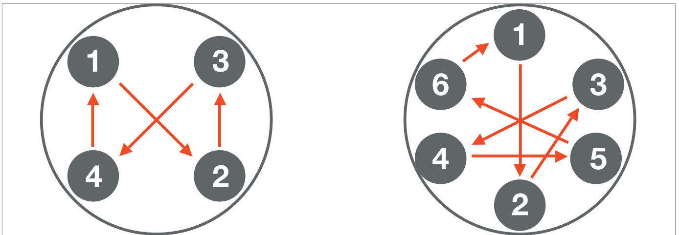
Fig. 9.20. Schéma en croix
