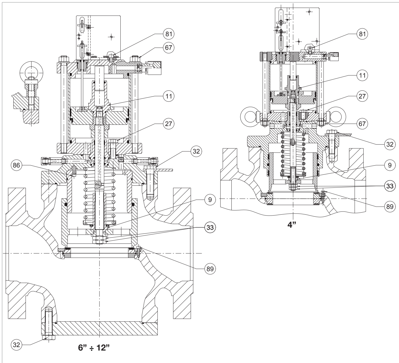
Fig. 9.15. Couples de serrage du clapet de sécurité intégré HBC 975
