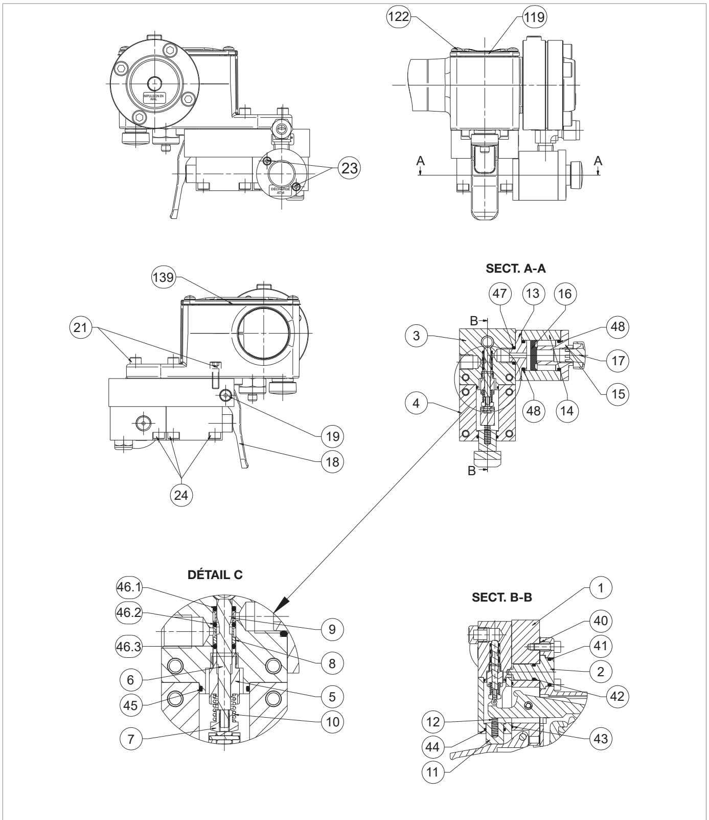
Fig. 9.31. Vanne 3/2
