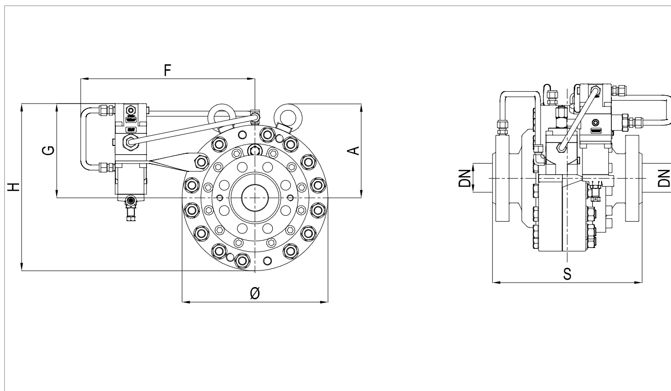
Fig. 5.11. Caratteristiche fisiche ASX 176 (+LDB/176)
