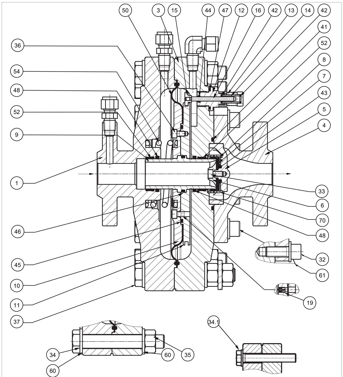
Fig. 9.44. Regolatore ASX 176 con silenziatore LDB/176 1"
