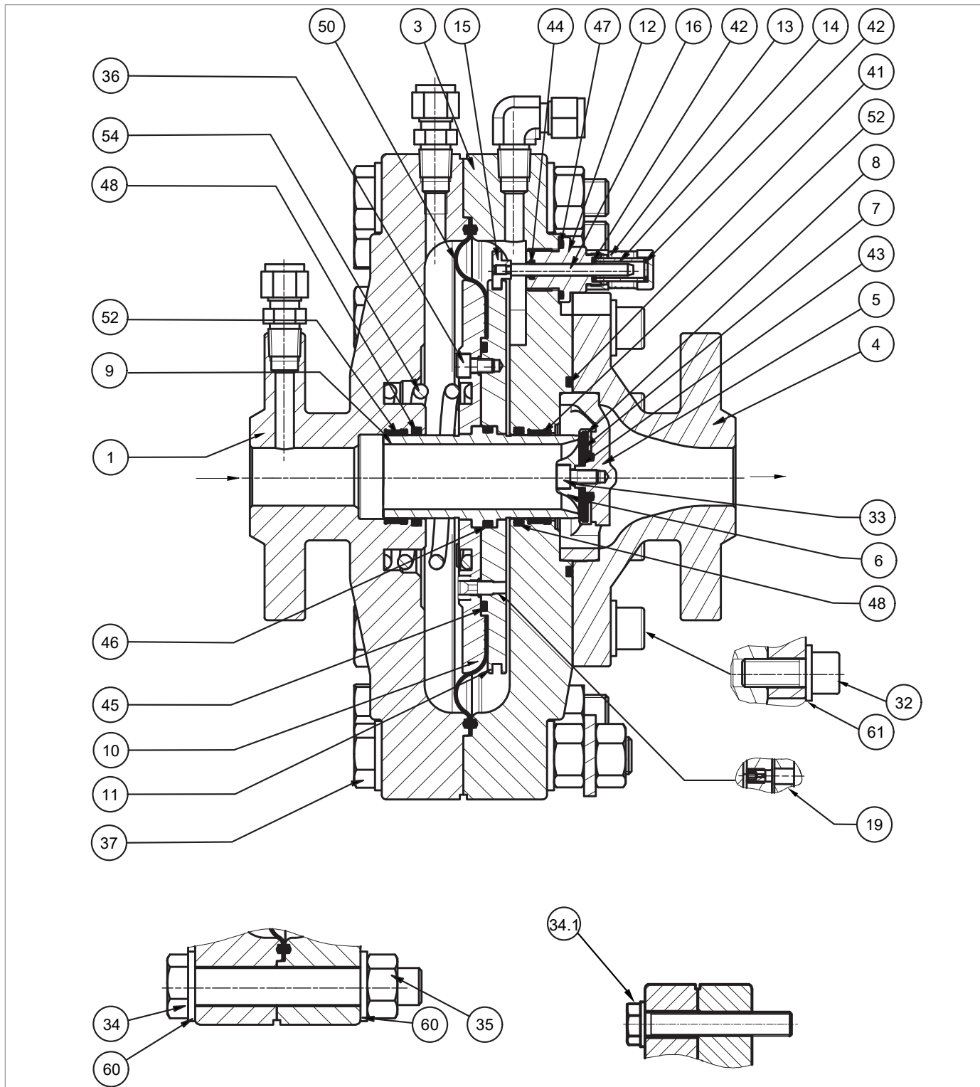
Fig. 9.42. Regolatore ASX 176 1"
