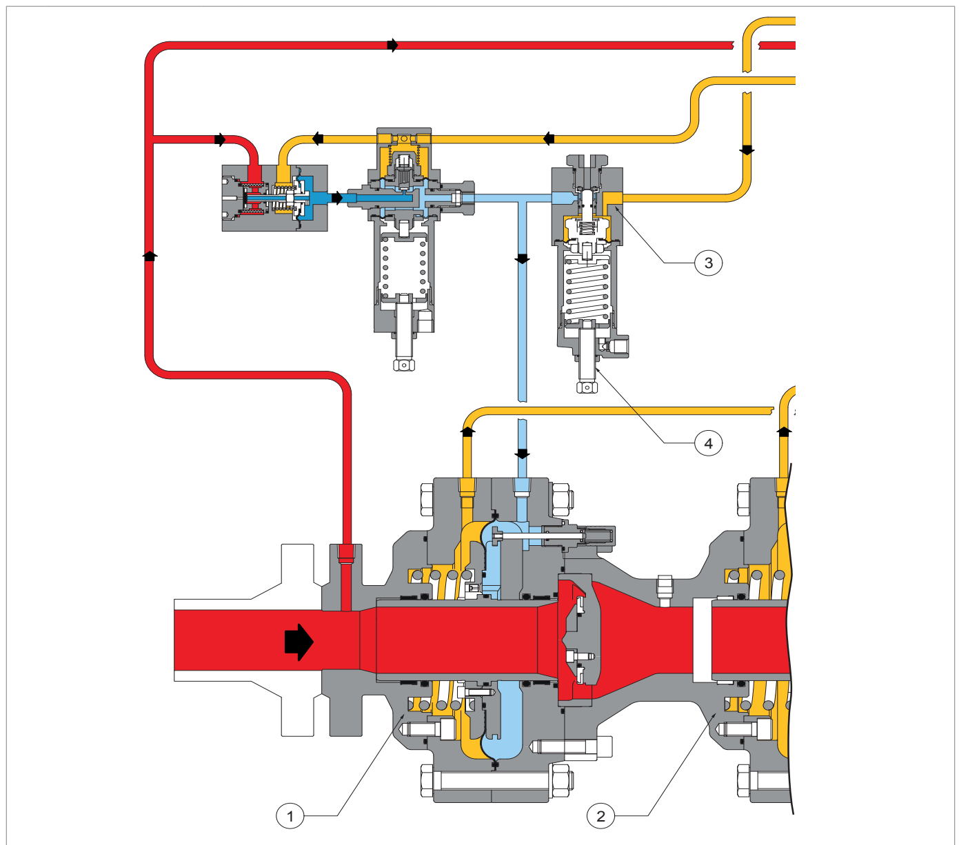
■ PRESSIONE DI MONTE ■ PRESSIONE DI VALLE ■ PRESS. PRERIDUTTORE ■ PRESSIONE MOTORIZZAZIONE MONITOR
