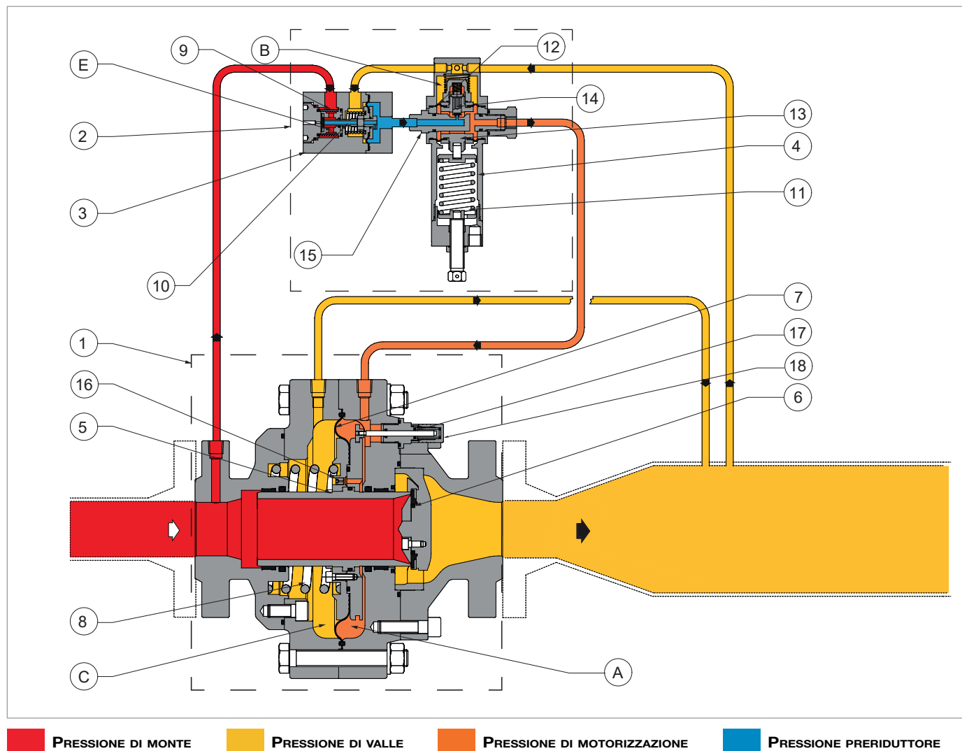
Fig. 4.2. Funzionamento ASX 176
